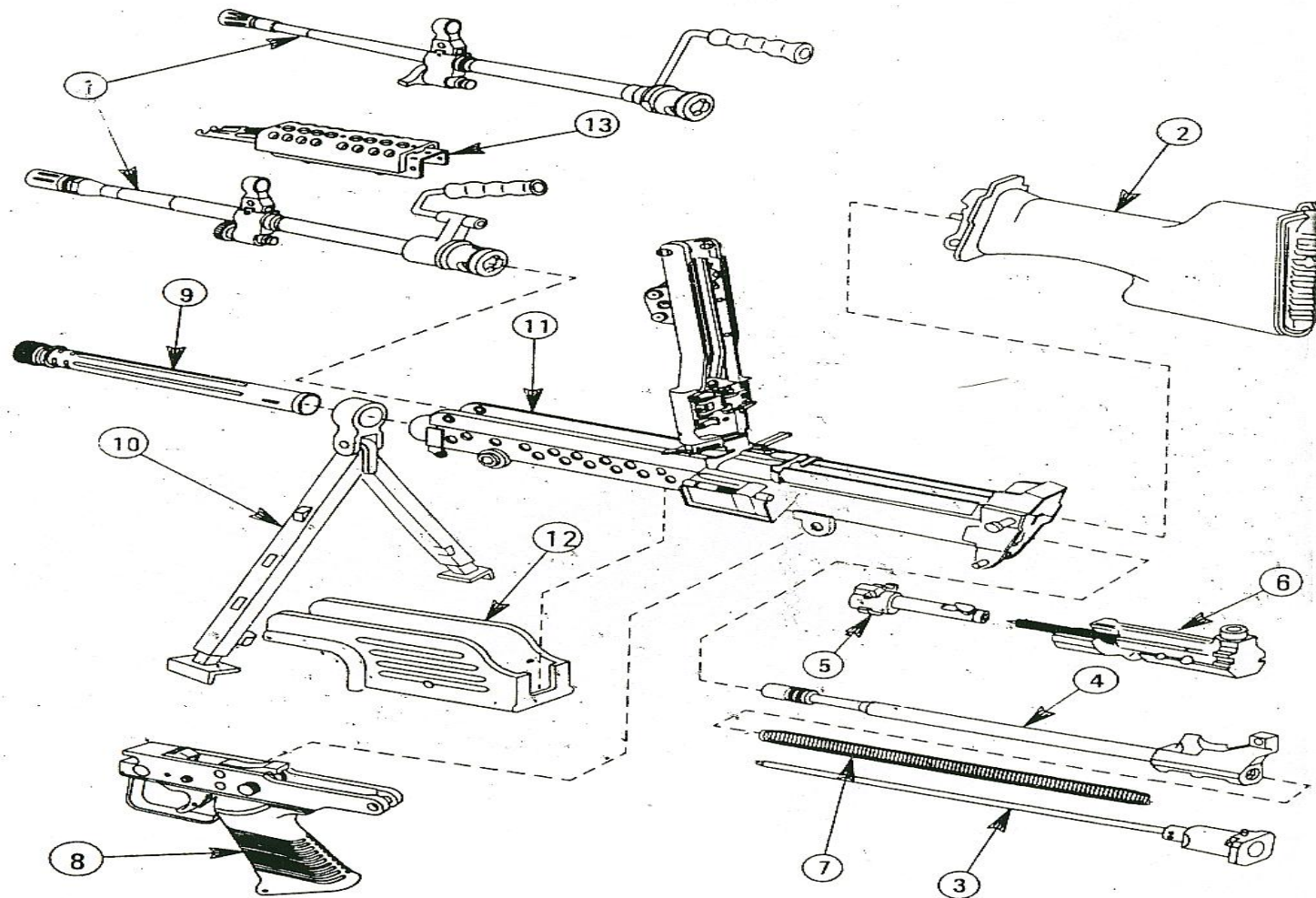
ภาพที่ 1 องค์ประกอบหลักของปืนกลขนาด 5.56 มม. เอ็ม 249
