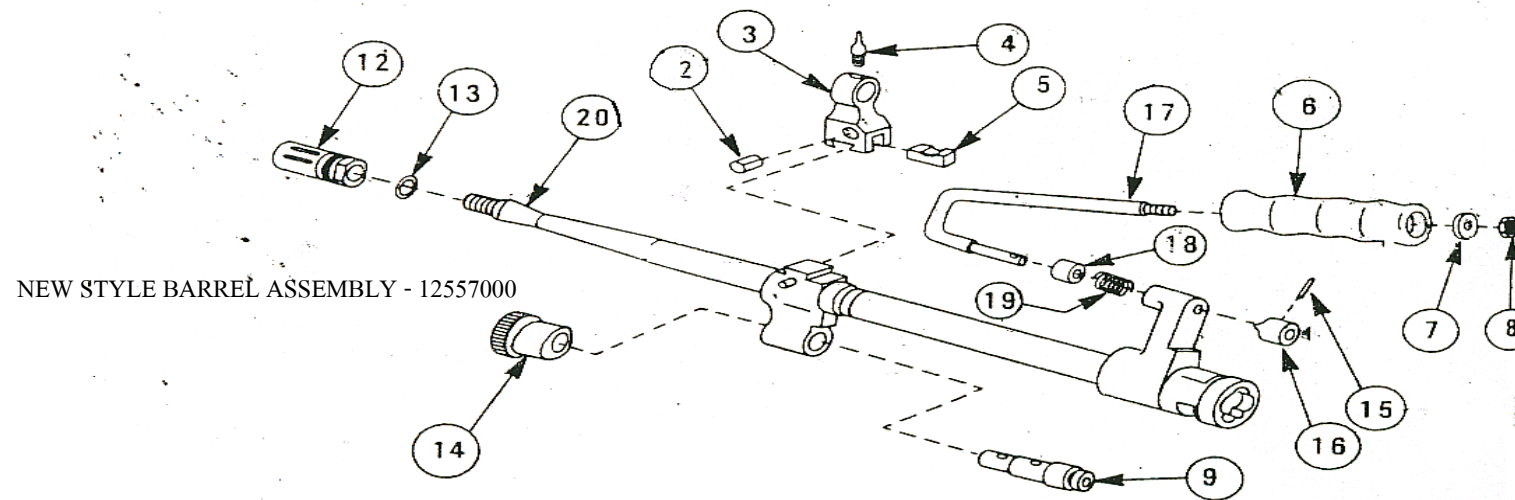
ภาพที่ 2 ชุดล่ากล้องปืน
