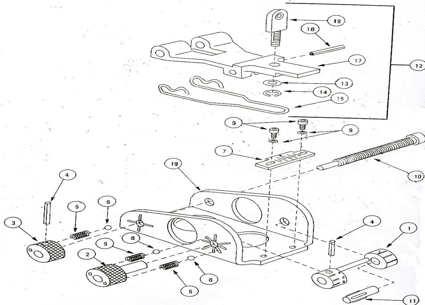
ภาพที่ 10 ชุดศูนย์หลัง
