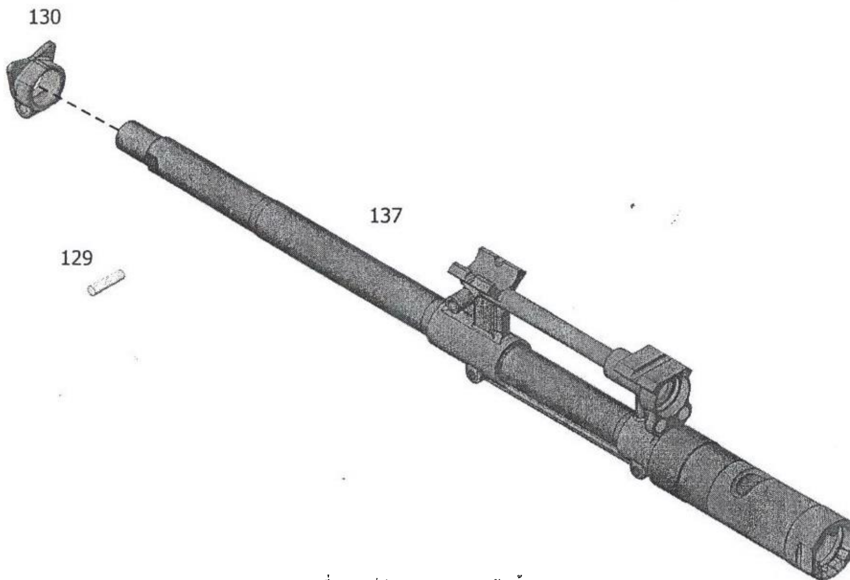
ภาพที่ 35 องค์ประกอบของชุดล่ากล้องสั้น
