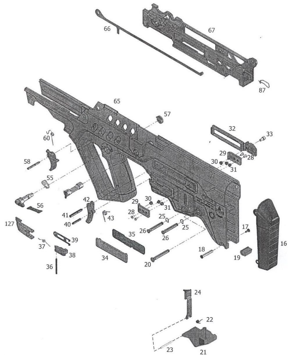
ภาพที่ 14 ชุดองค์ประกอบของชุดโครป็น (2/2)
