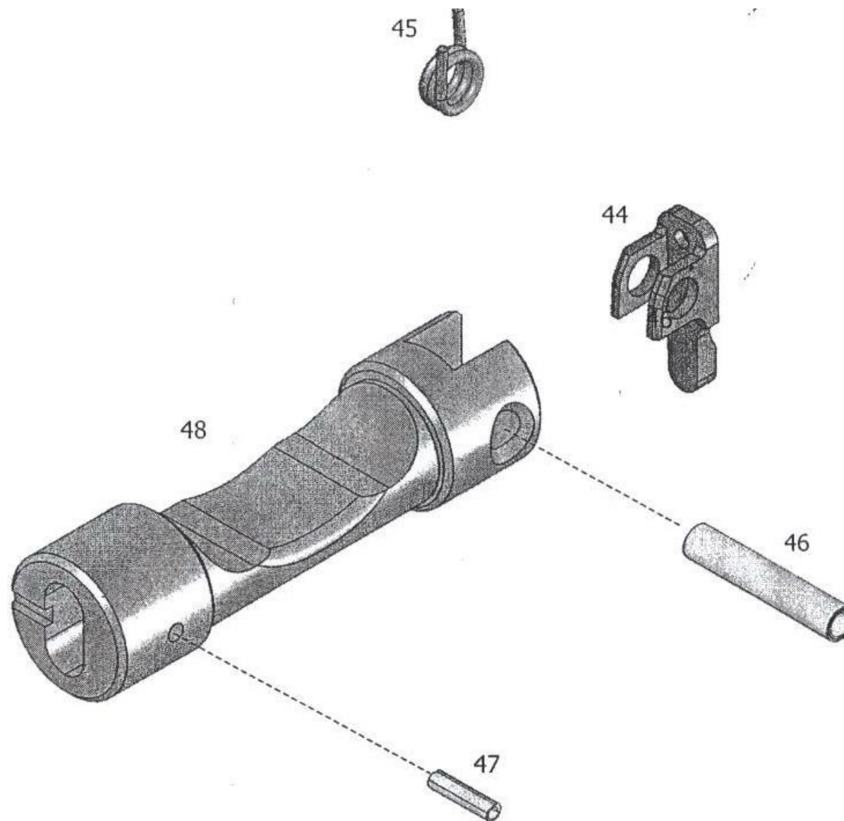
ภาพที่ 16 องค์ประกอบของชุดกลอนยึดลำกล้องปืน
