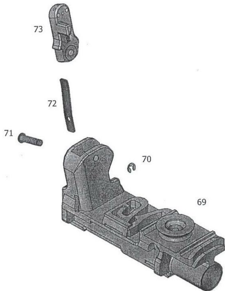
ภาพที่ 31 องค์ประกอบของชุดกระบอกสูบแก๊ส
