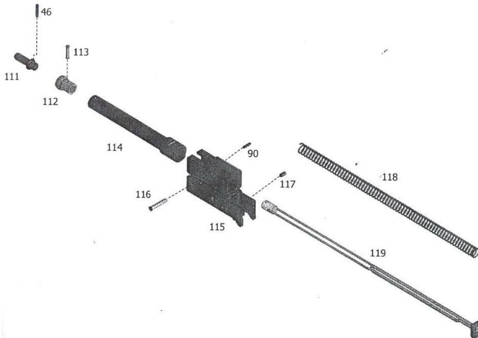
ภาพที่ 43 องค์ประกอบของชุดโครงนำลูกเลื่อน
