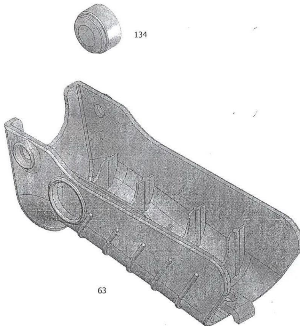
ภาพที่ 6 องค์ประกอบของประกับรองมือ
