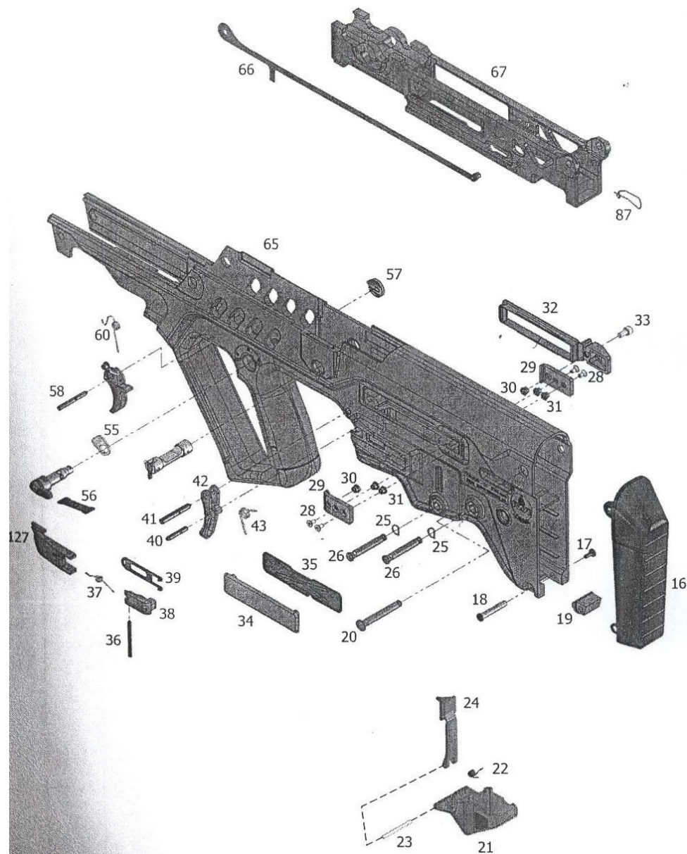
ภาพที่ 13 ชุดองค์ประกอบของชุดโครงปืน (1/2)
