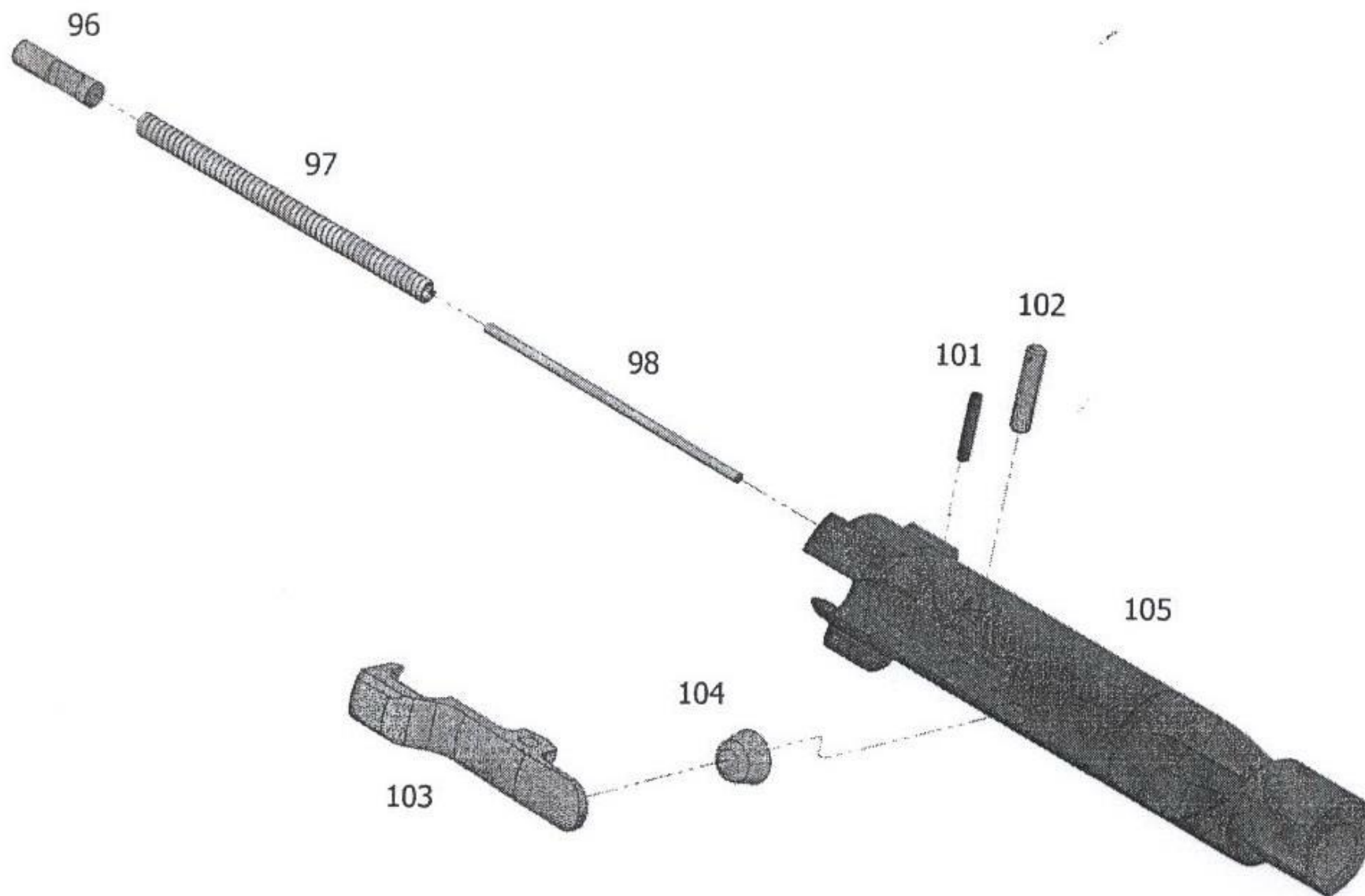
ภาพที่ 41 องค์ประกอบของชุดลูกเลื่อนแบบคัตปล็อกด้านซ้าย
