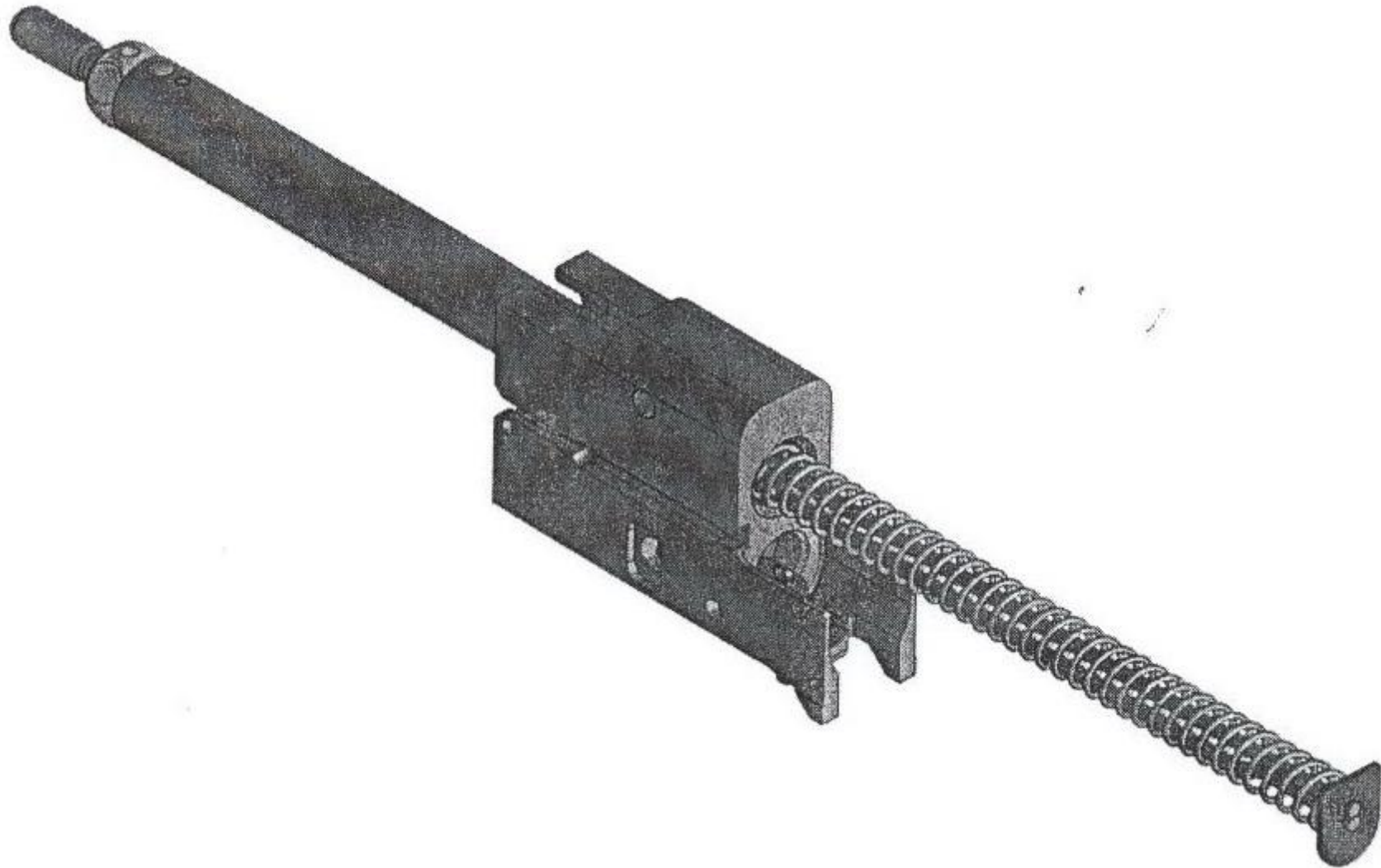
ภาพที่ 42 ชุดโครงนำลูกเลื่อน
