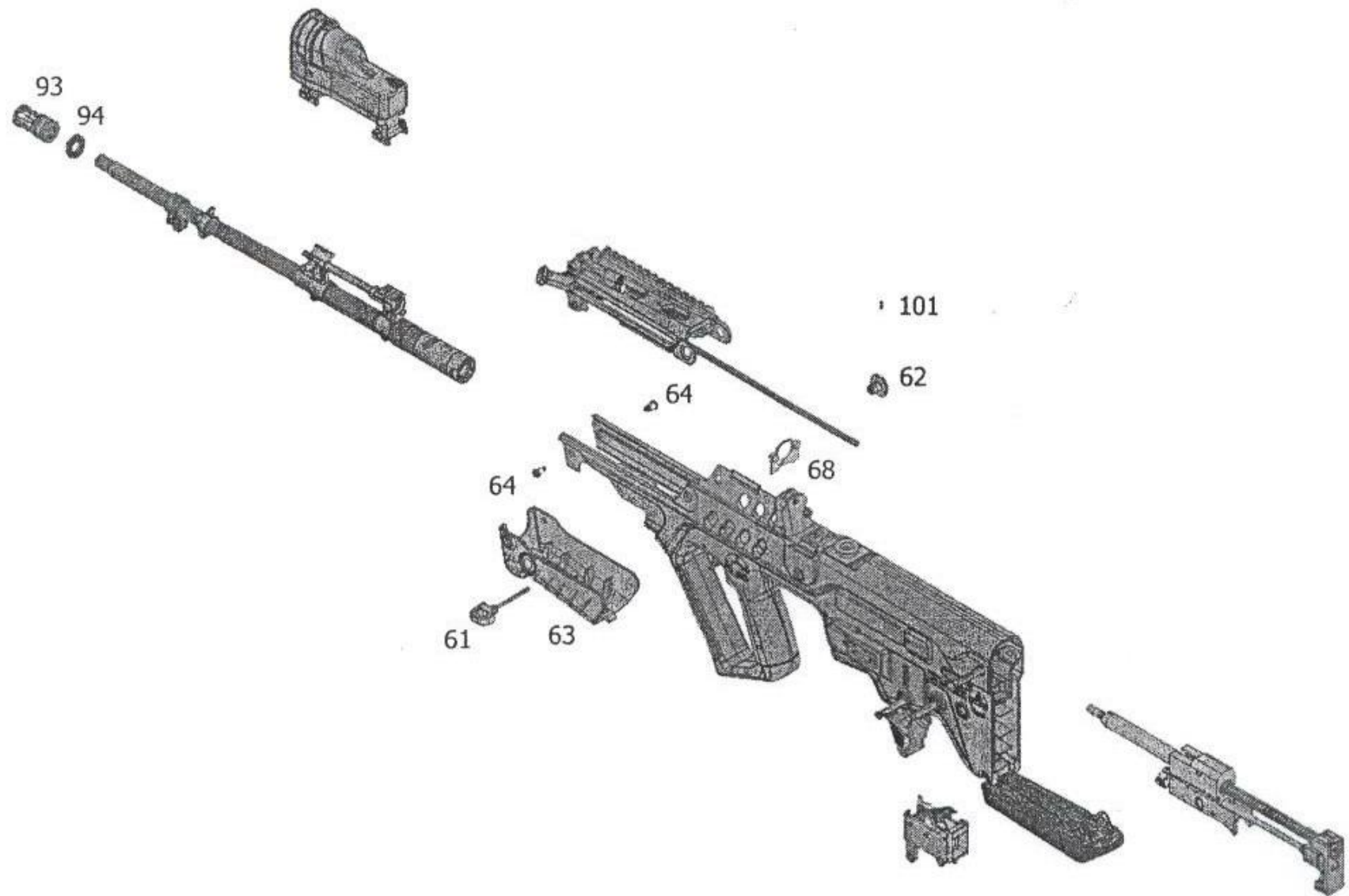
ภาพที่ 2 องค์ประกอบของปืนเล็กยาวทาวอร์ ทาร์ - 21 ขนาด 5.56 มม.
