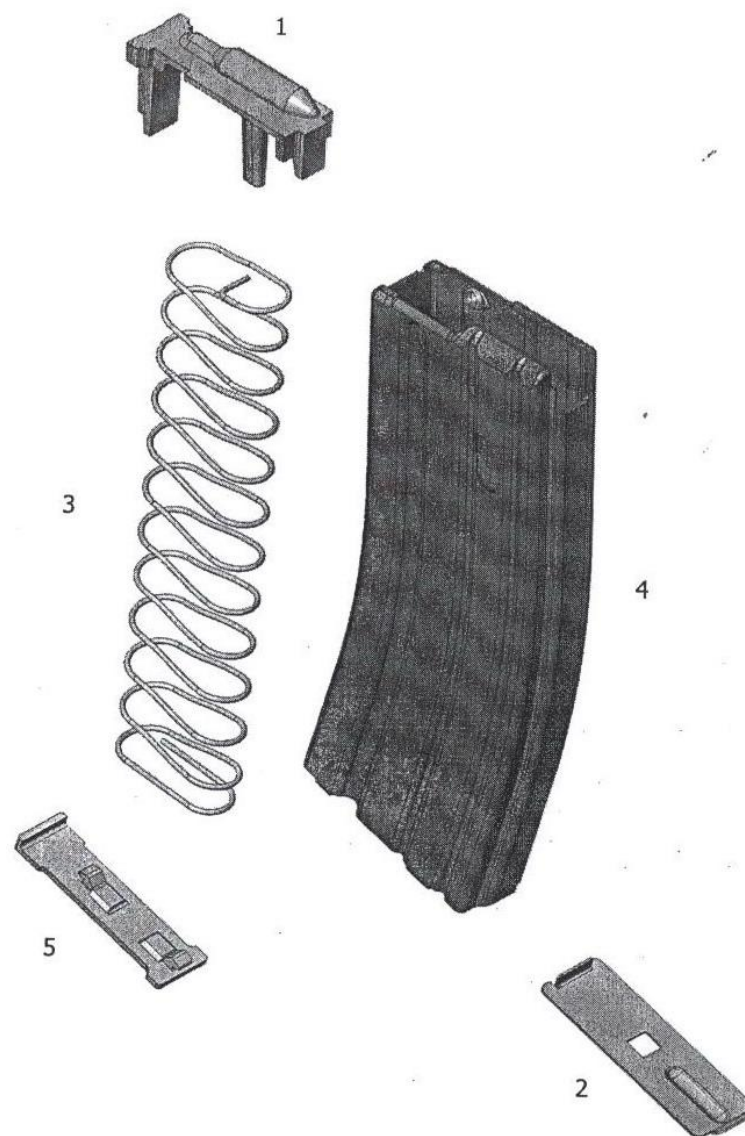
ภาพที่ 55 องค์ประกอบของซองกระสุน
