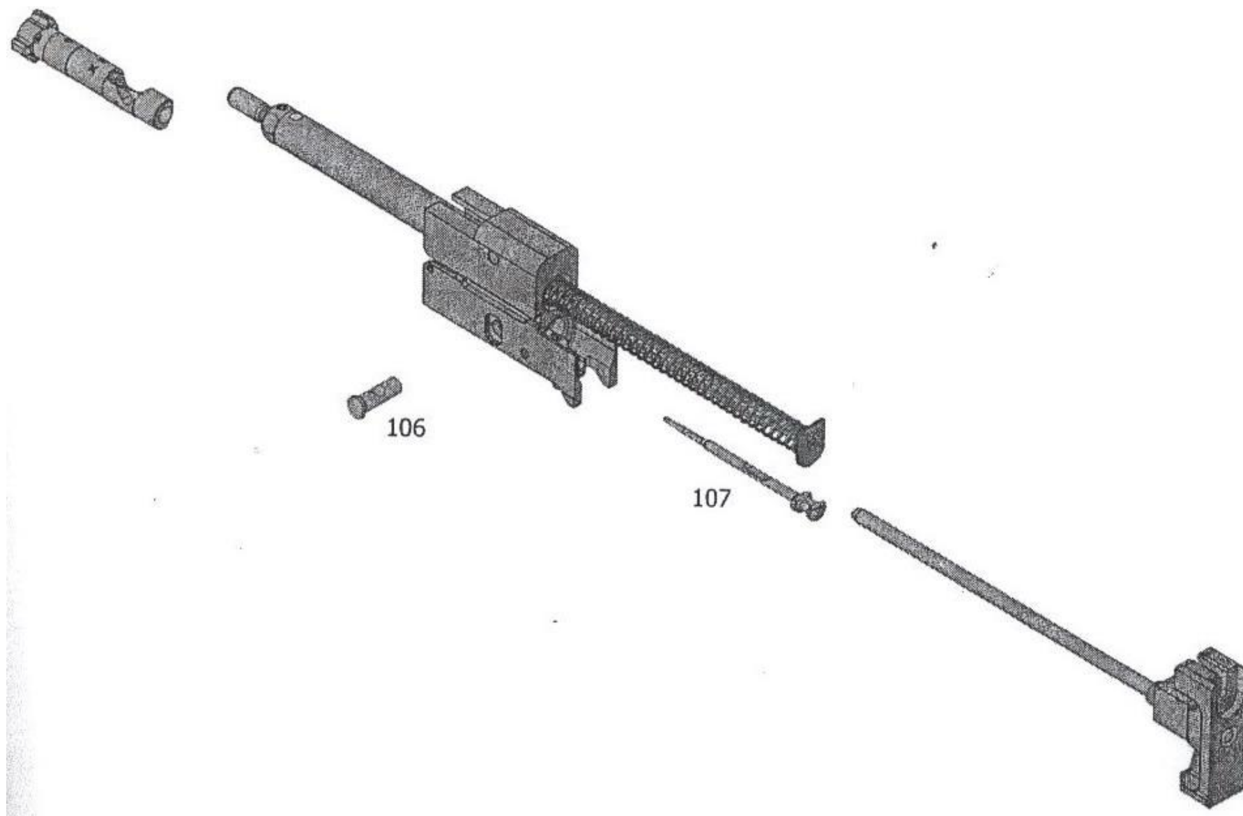
ภาพที่ 37 องค์ประกอบของชุดเคลื่อนถอย
