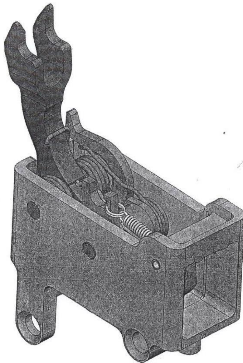
ภาพที่ 46 ชุดเครื่องลั่นไก
