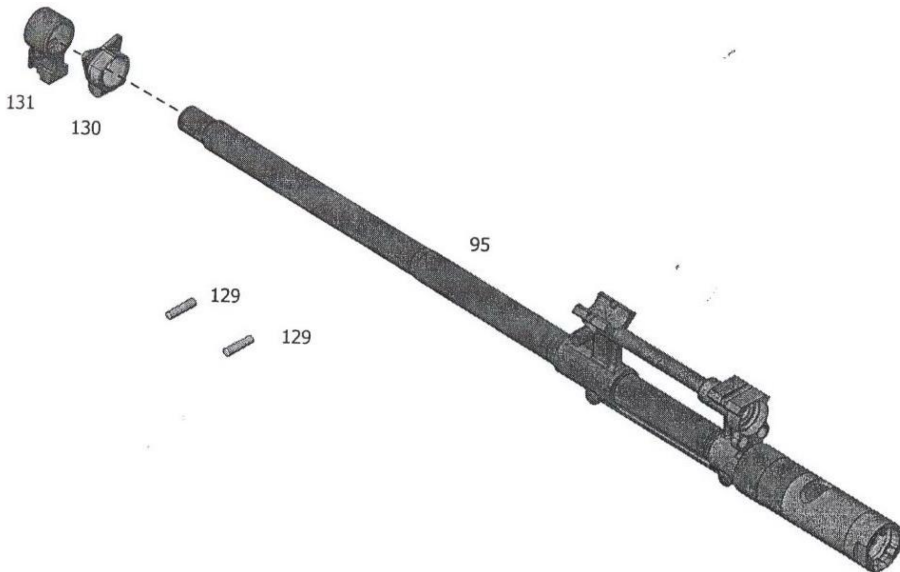
ภาพที่ 33 องค์ประกอบของชุดลากสือ่งปืน
