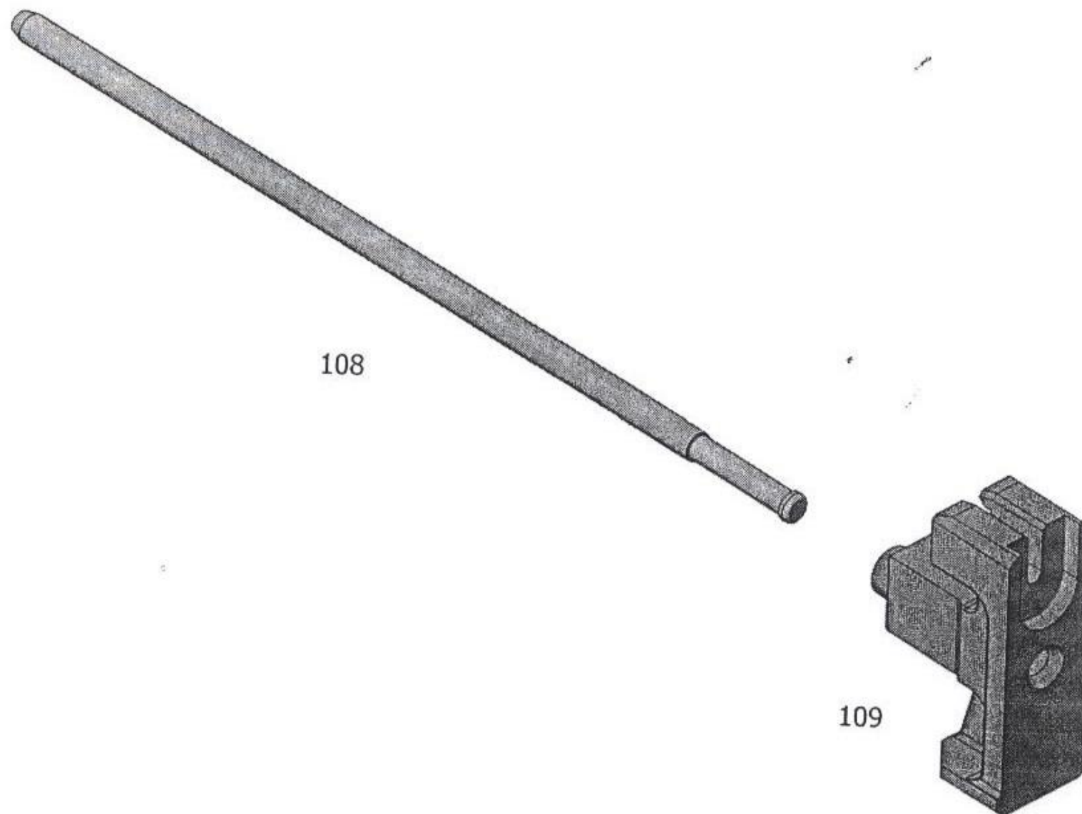
ภาพที่ 45 องค์ประกอบของชุดแกนนำโรคนำลูกเลื่อน
