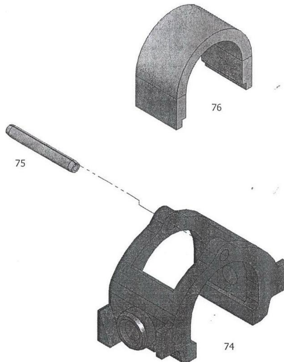
ภาพที่ 25 องค์ประกอบของชุดปลดกรักษาการทรงตัวของศูนย์เตียง
