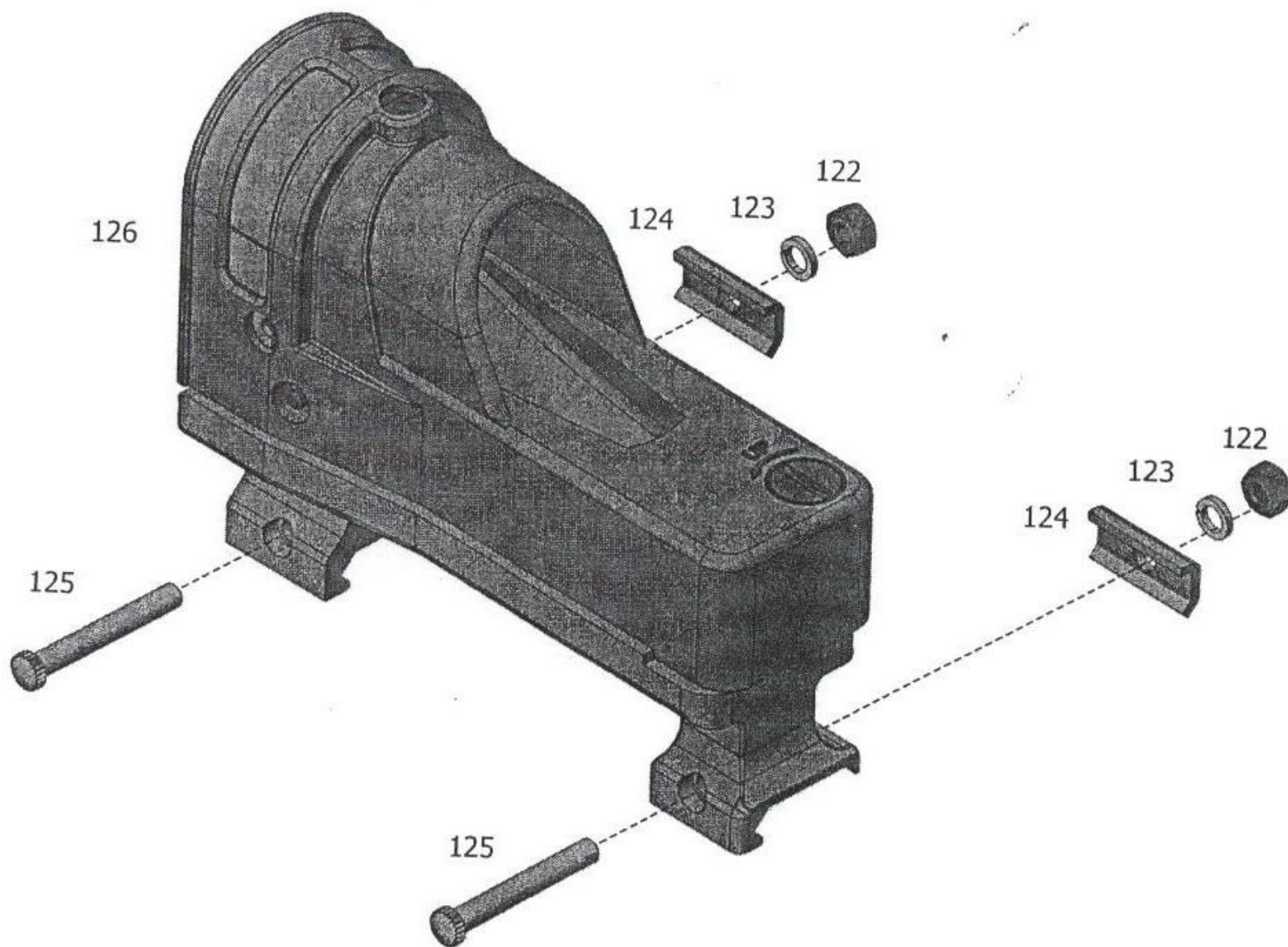
ภาพที่ 49 องค์ประกอบของชุดกล้องเล็งสะท้อนแสงเมโปร - 21
