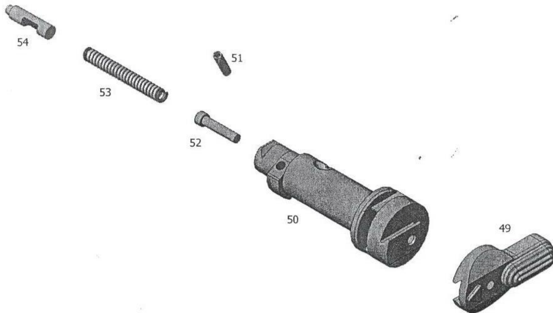
ภาพที่ 18 องค์ประกอบของชุดคันบังคับการยิง
