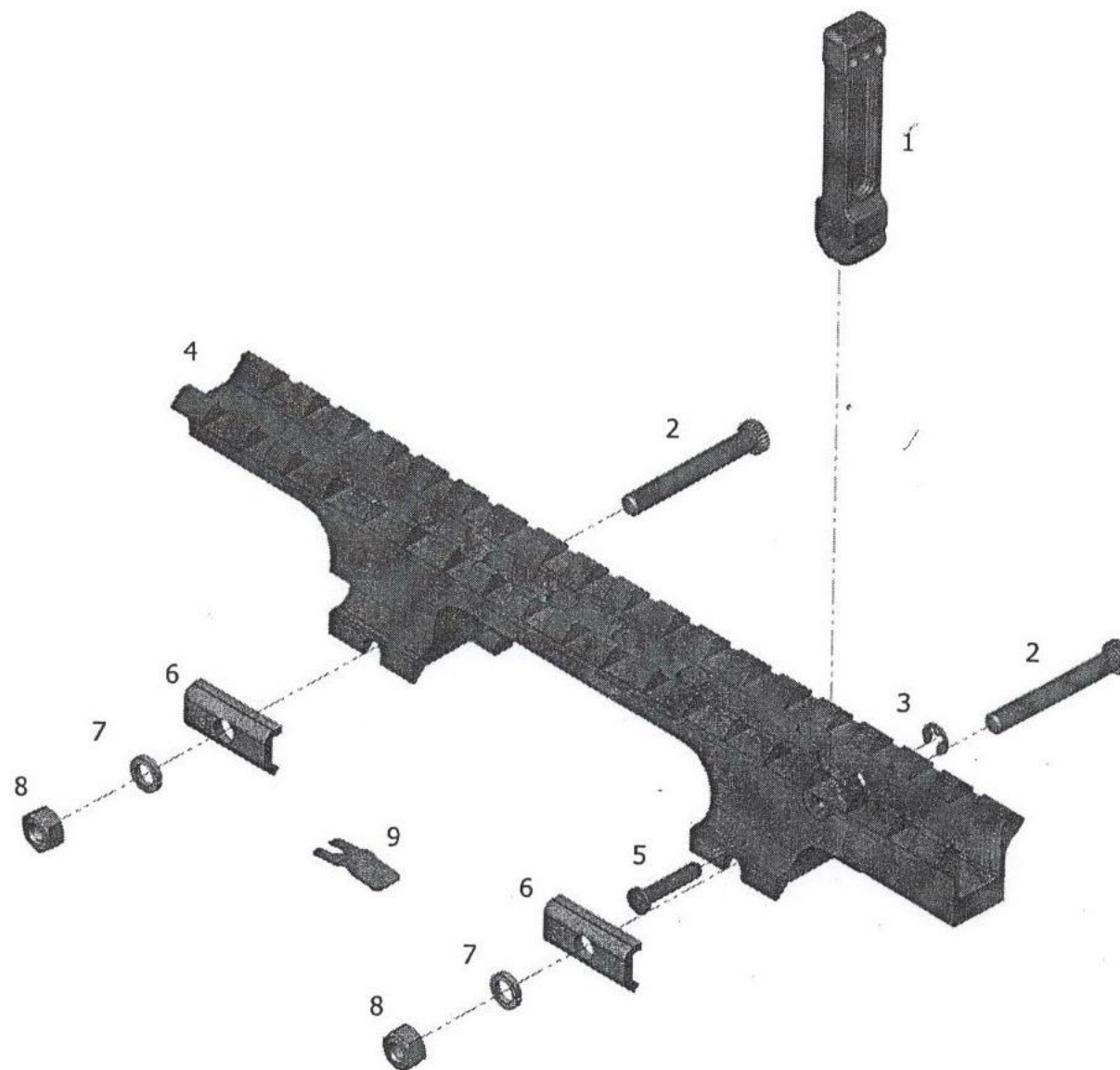
ภาพที่ 58 องค์ประกอบของแขนรางอนกประสงค์
