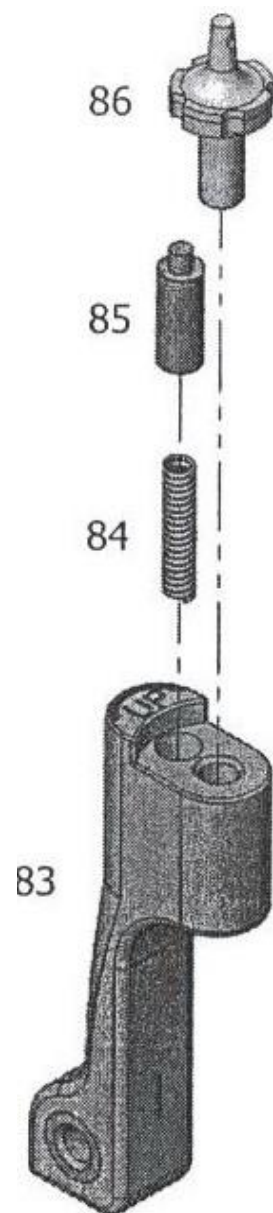
ภาพที่ 23 องค์ประกอบของชุดใบศูนย์หน้า
