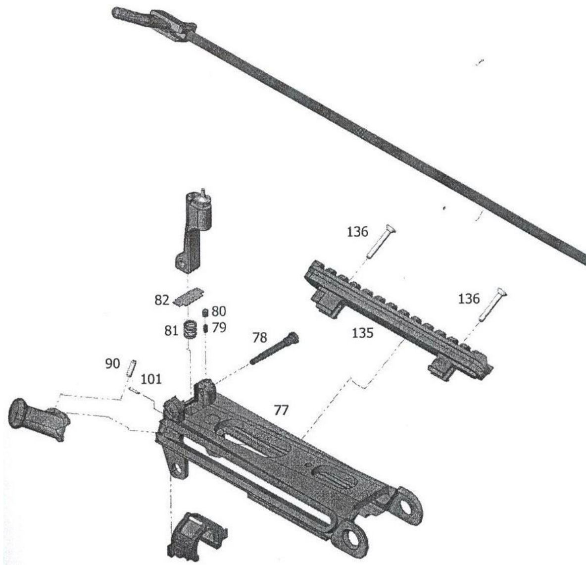
ภาพที่ 21 องค์ประกอบของชุดโรจนำคันเร่งลูกเลื่อน
