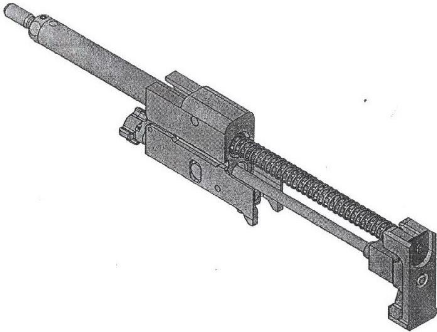
ภาพที่ 36 ชุดเคลื่อนถอย
