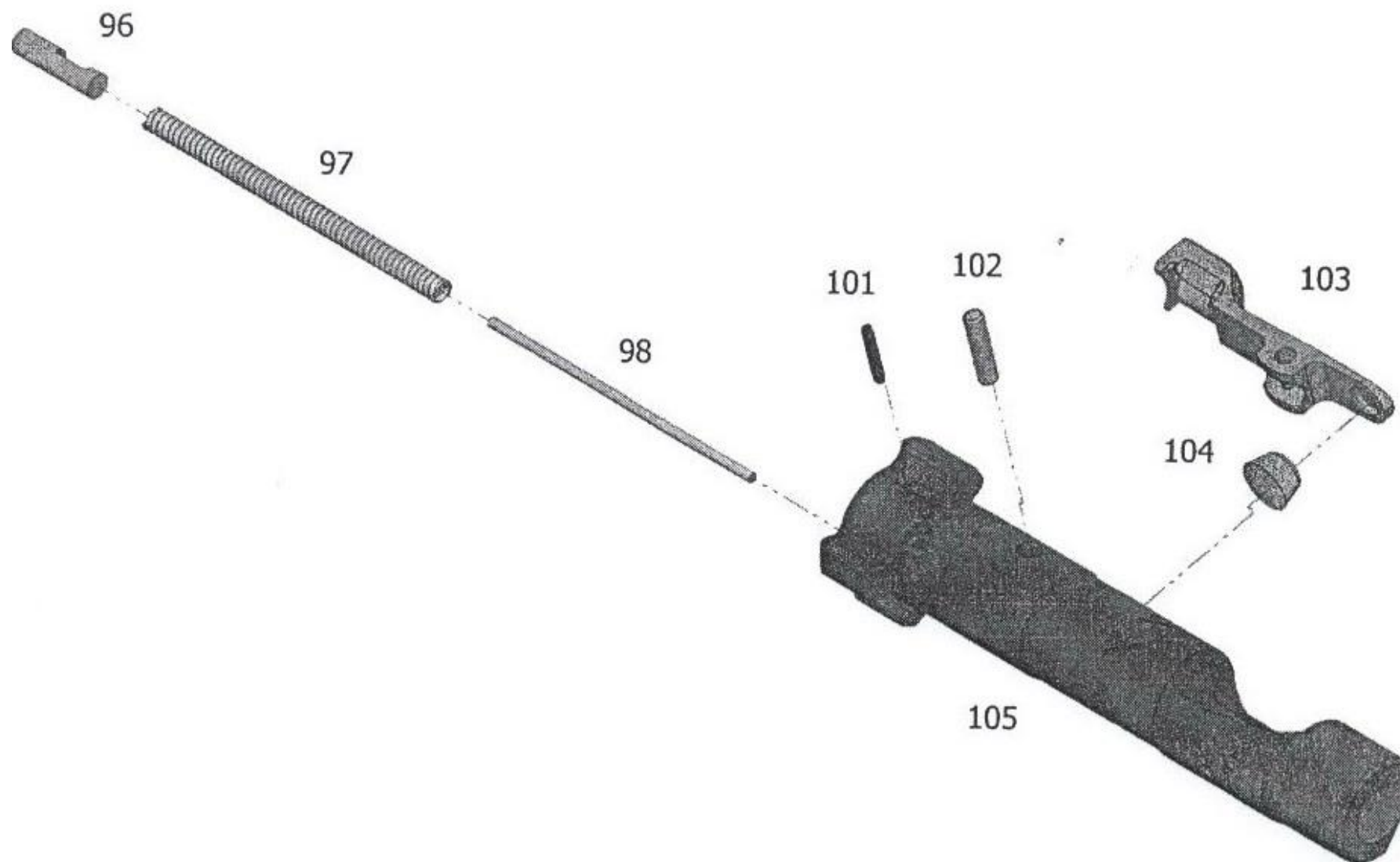
ภาพที่ 39 องค์ประกอบของชุดลูกเลื่อนแบบคัตปล็อกด้านขวา
