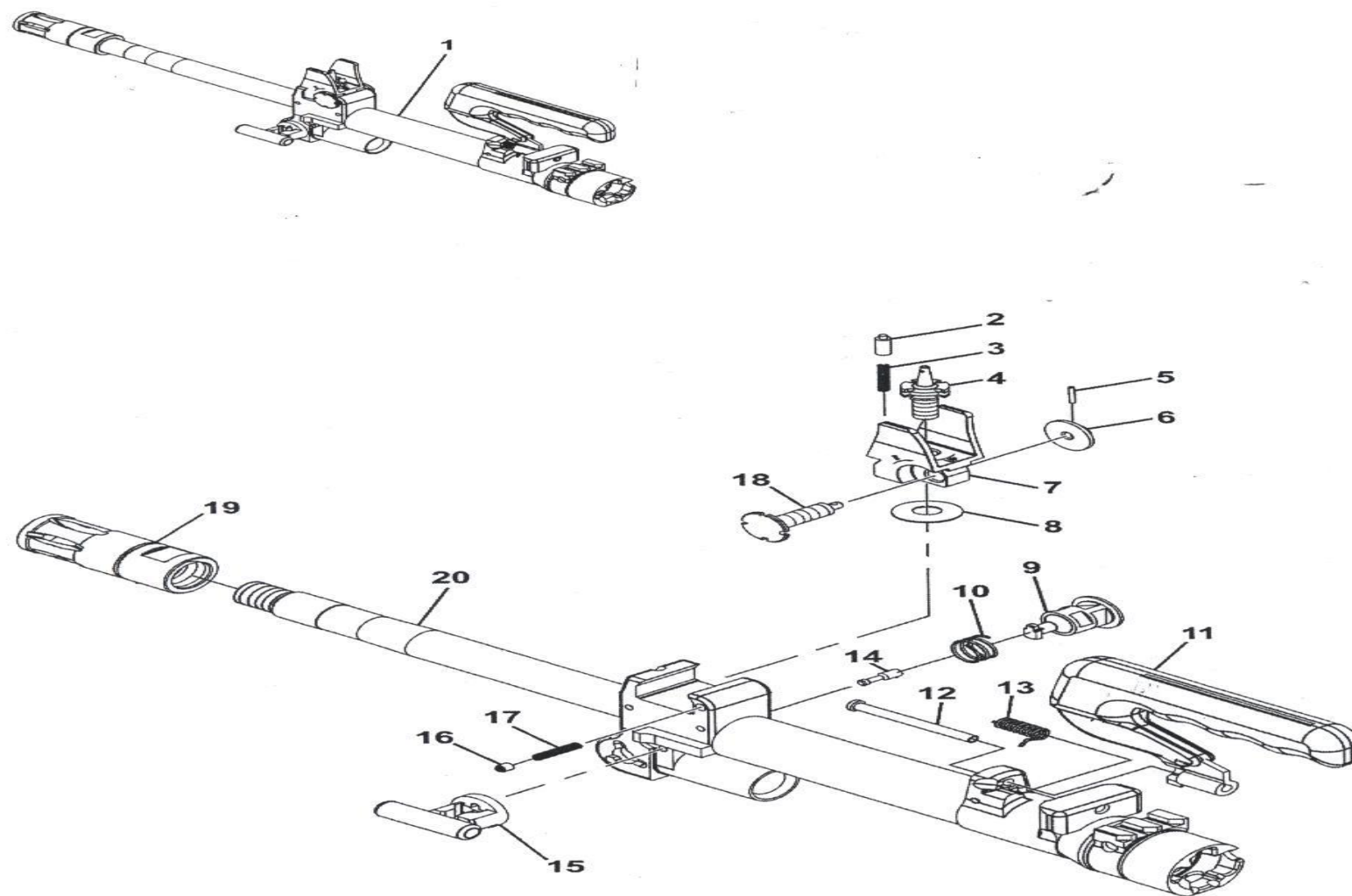
ภาพที่ 7 ชุดล่าก๊อง (สั๊น) พร้อมปลอกกดแรงแบบ RG
