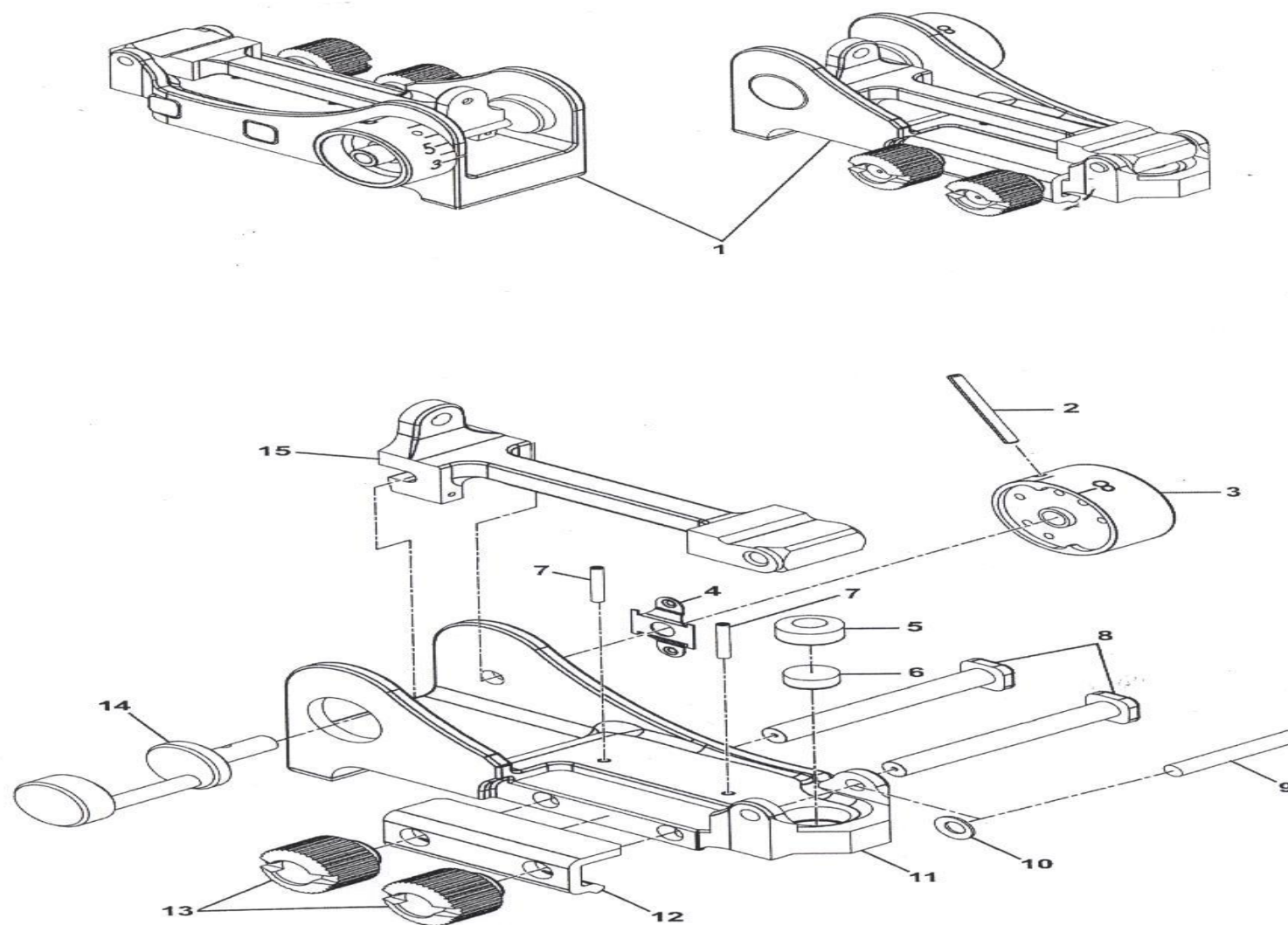
ภาพที่ 5 ชุดศูนย์หลังแบบถอดได้ของถ้ำกลิ้งชนิดยาว
