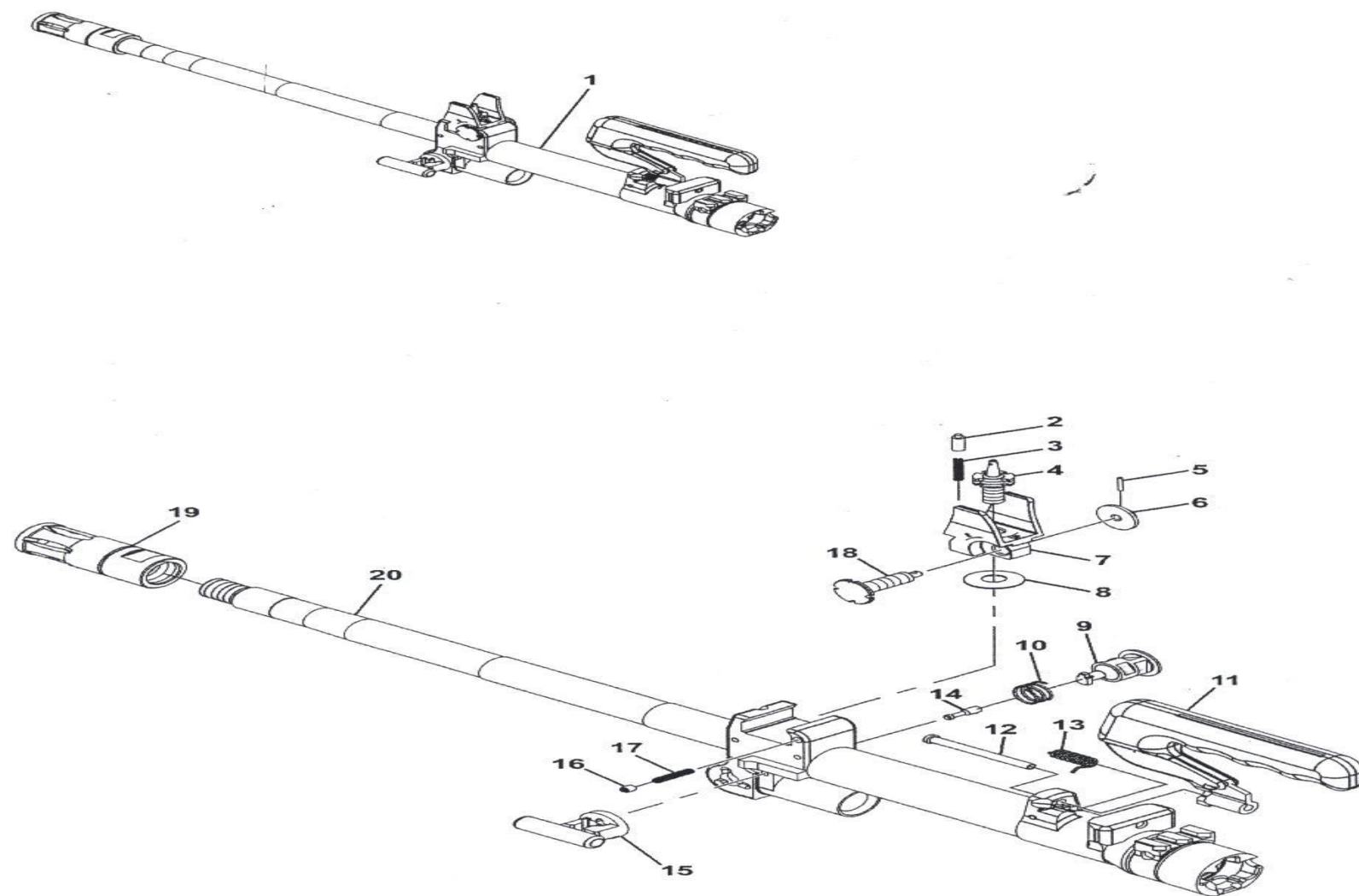
ภาพที่ 6 ชุดล่าก๊อ้ง พร้อมปลอกคดแรงแบบ RG
