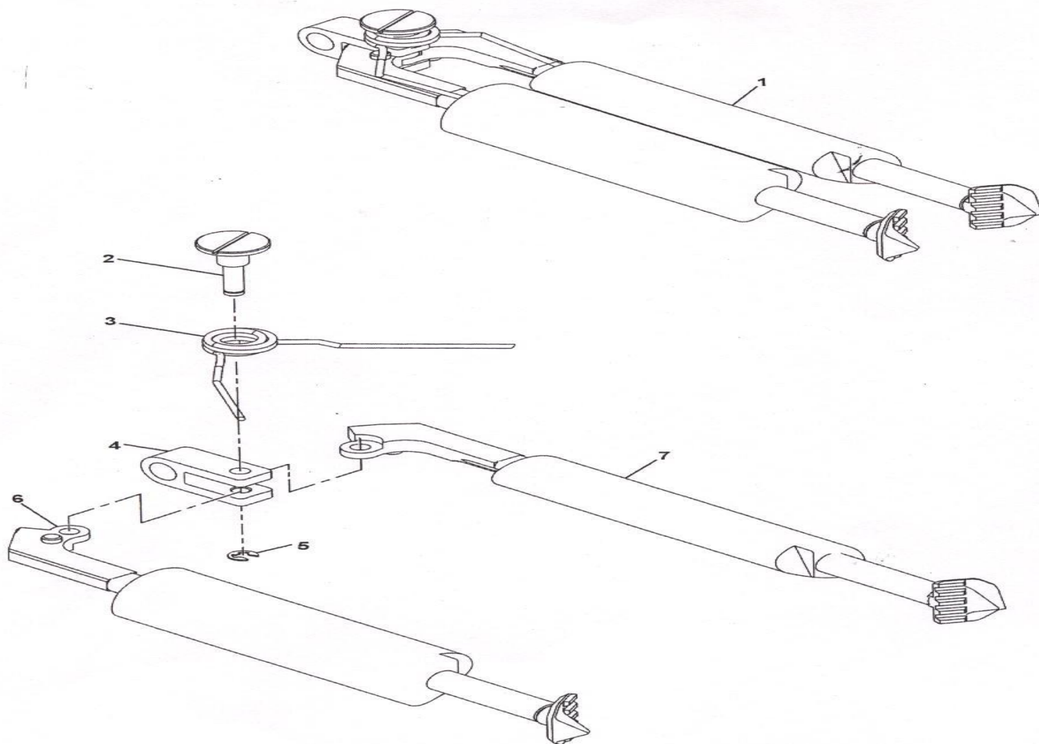
ภาพที่ 17 ชุดขาทราย
