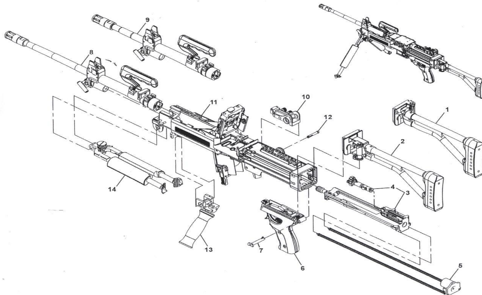
ภาพที่ 2 องค์ประกอบหลัก
