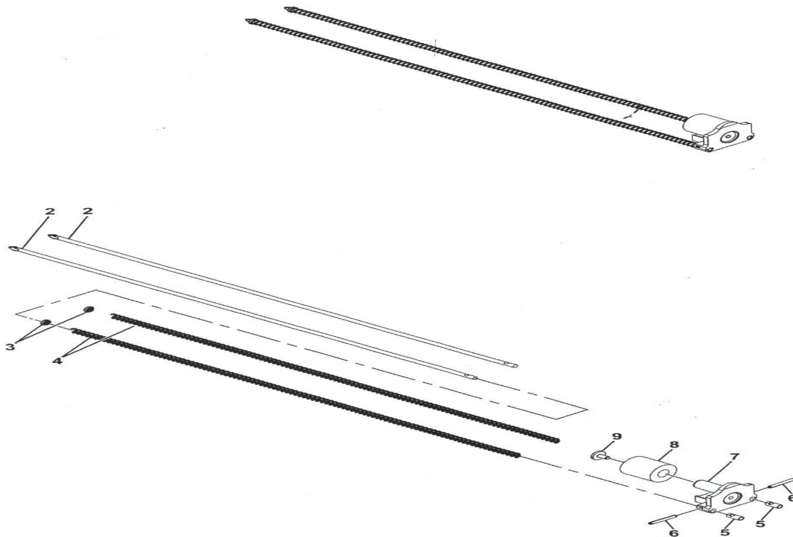
ภาพที่ 9 ชุดแหนบส่งลูกเลื่อน
