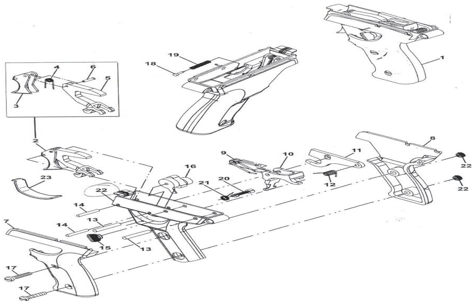
ภาพที่ 10 ชุดเครื่องสั้นไก
