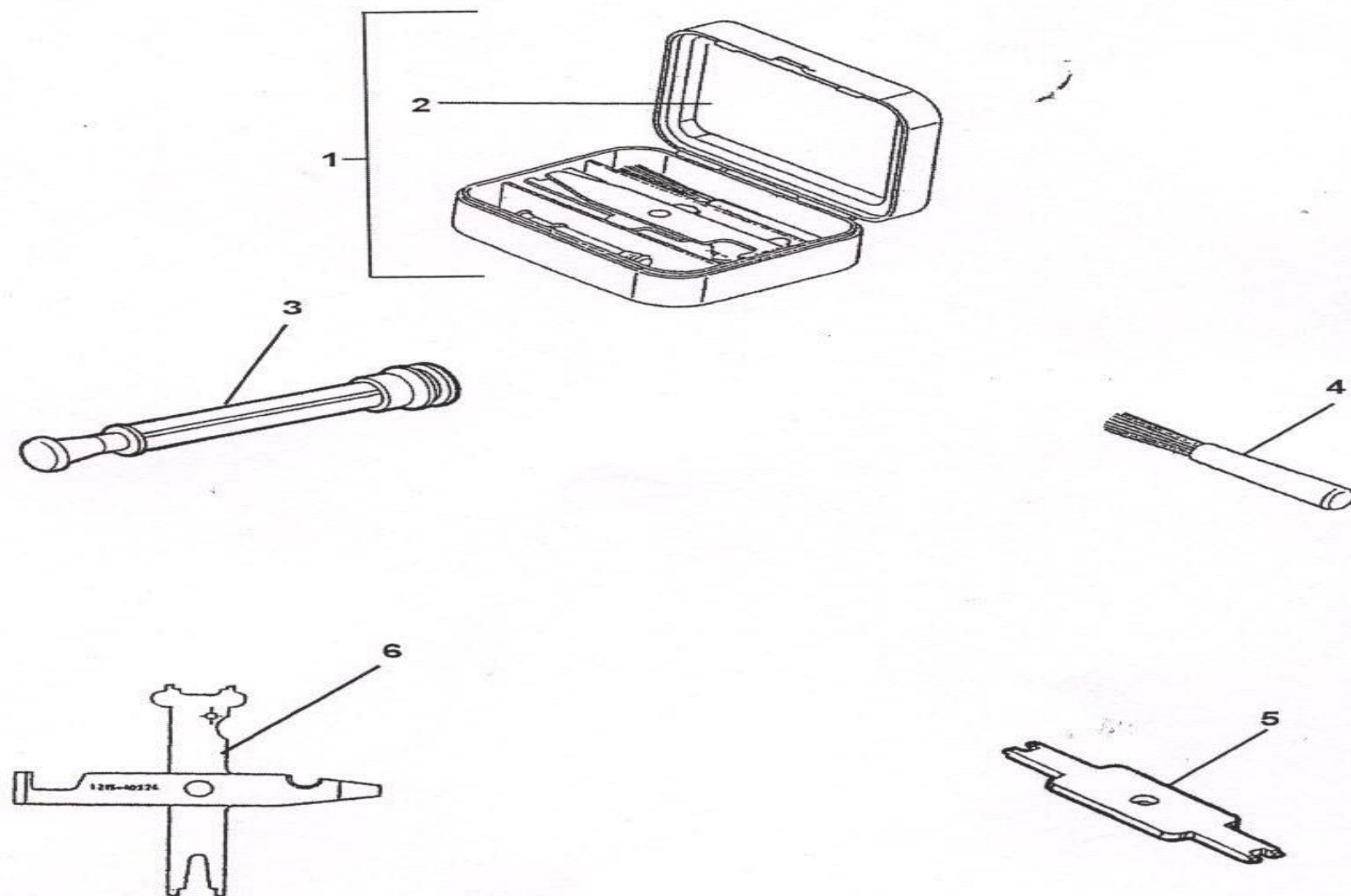
ภาพที่ 21 ชุดเครื่องมือทำความสะอาด
