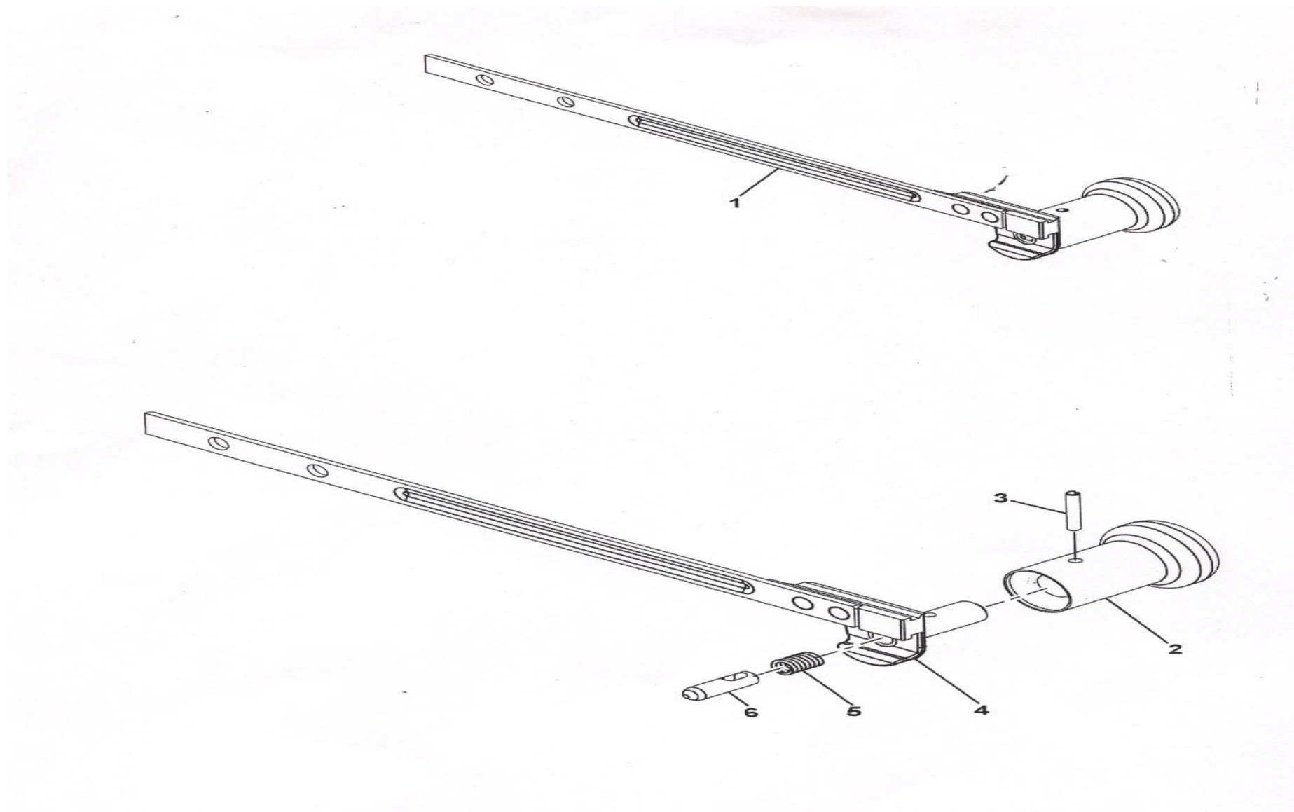
ภาพที่ 16 ชุดคันร้งลูกเลื่อน
