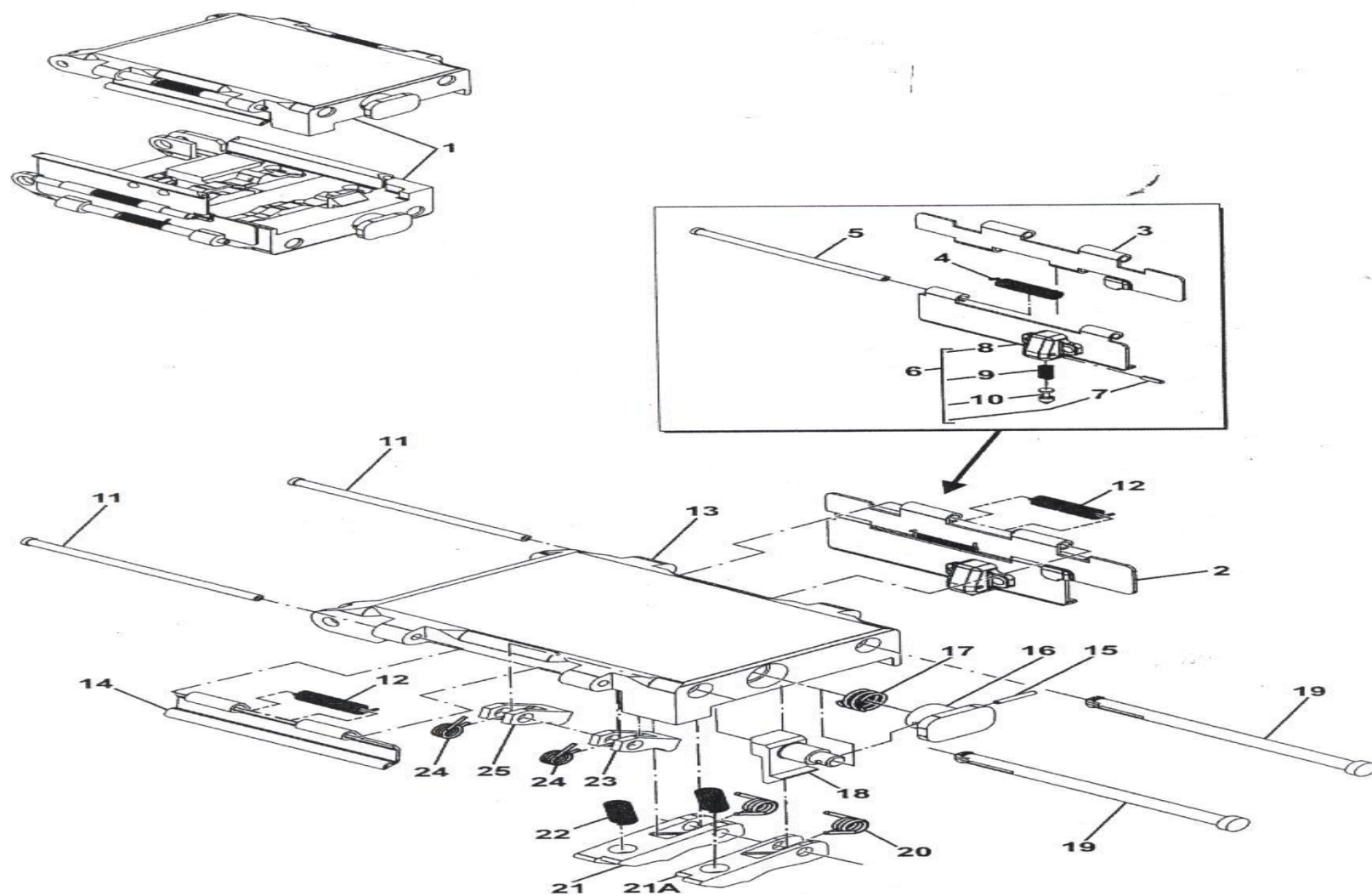
ภาพที่ 11 ชุดโครงปืน
