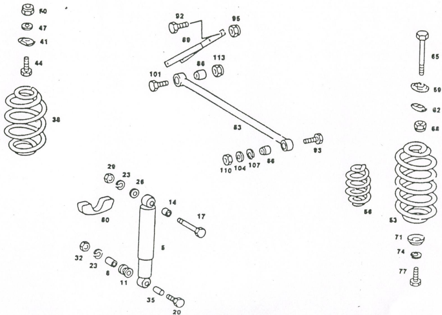
ภาพที่ 32/01-1 ระบบขดลวดและระบบกันสะเทือน
