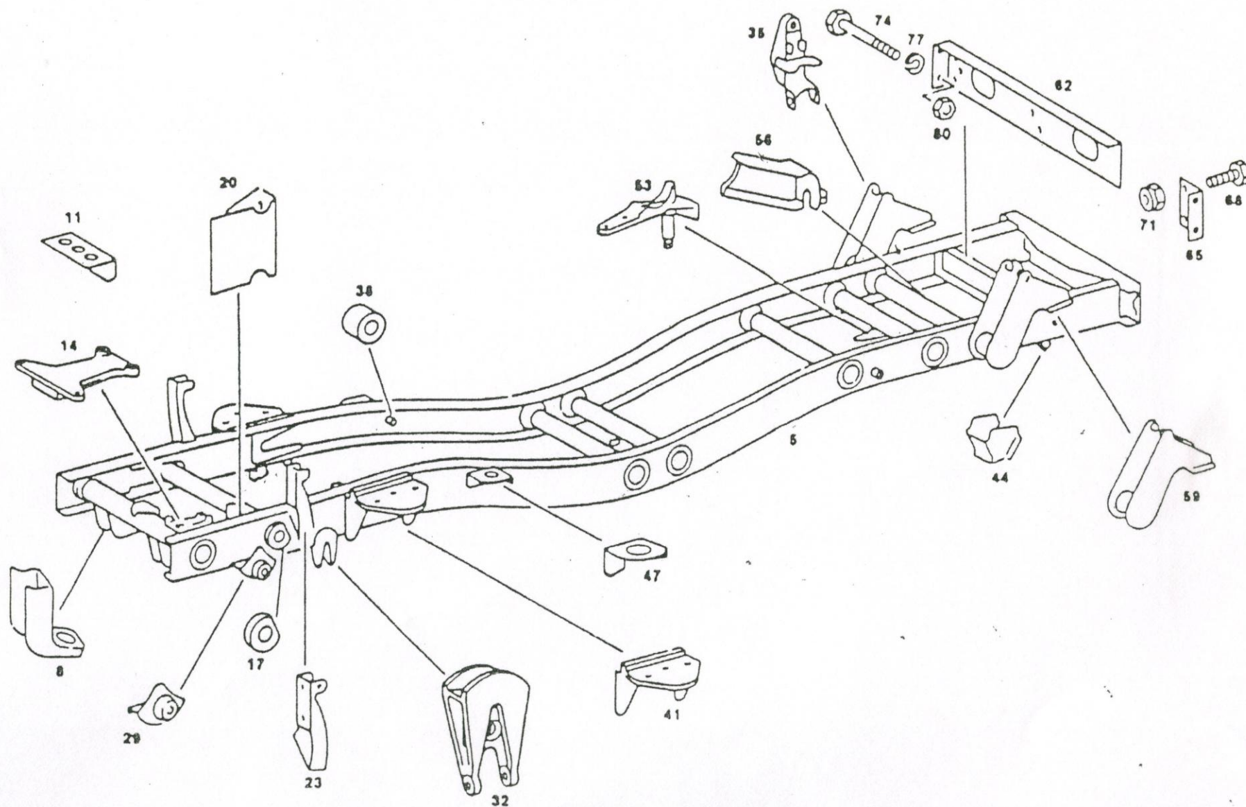
ภาพที่ 31/01-1 ระบบตัวถัง
