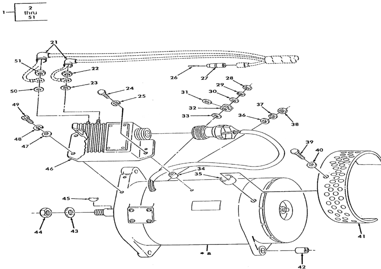
ภาพที่ 37 เครื่องกำเนิดไฟฟ้า ขนาด 200 แอมแปร์ (2)
