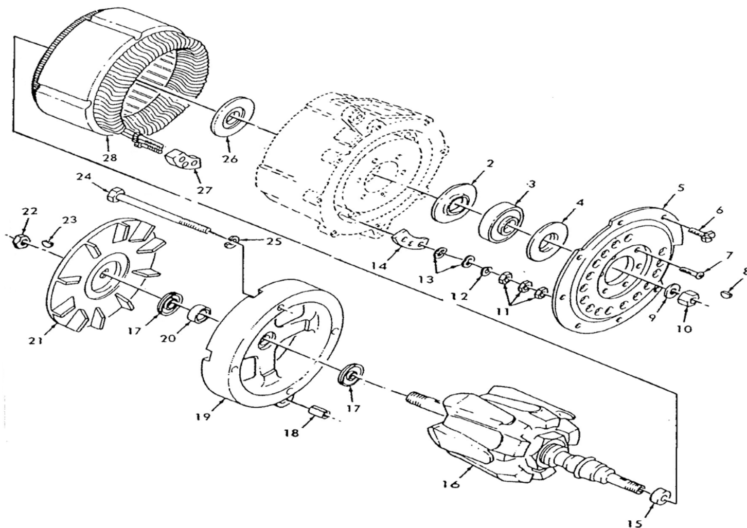
ภาพที่ 34 เครื่องกำเนิดไฟฟ้า ขนาด 200 แอมแปร์ (1)
