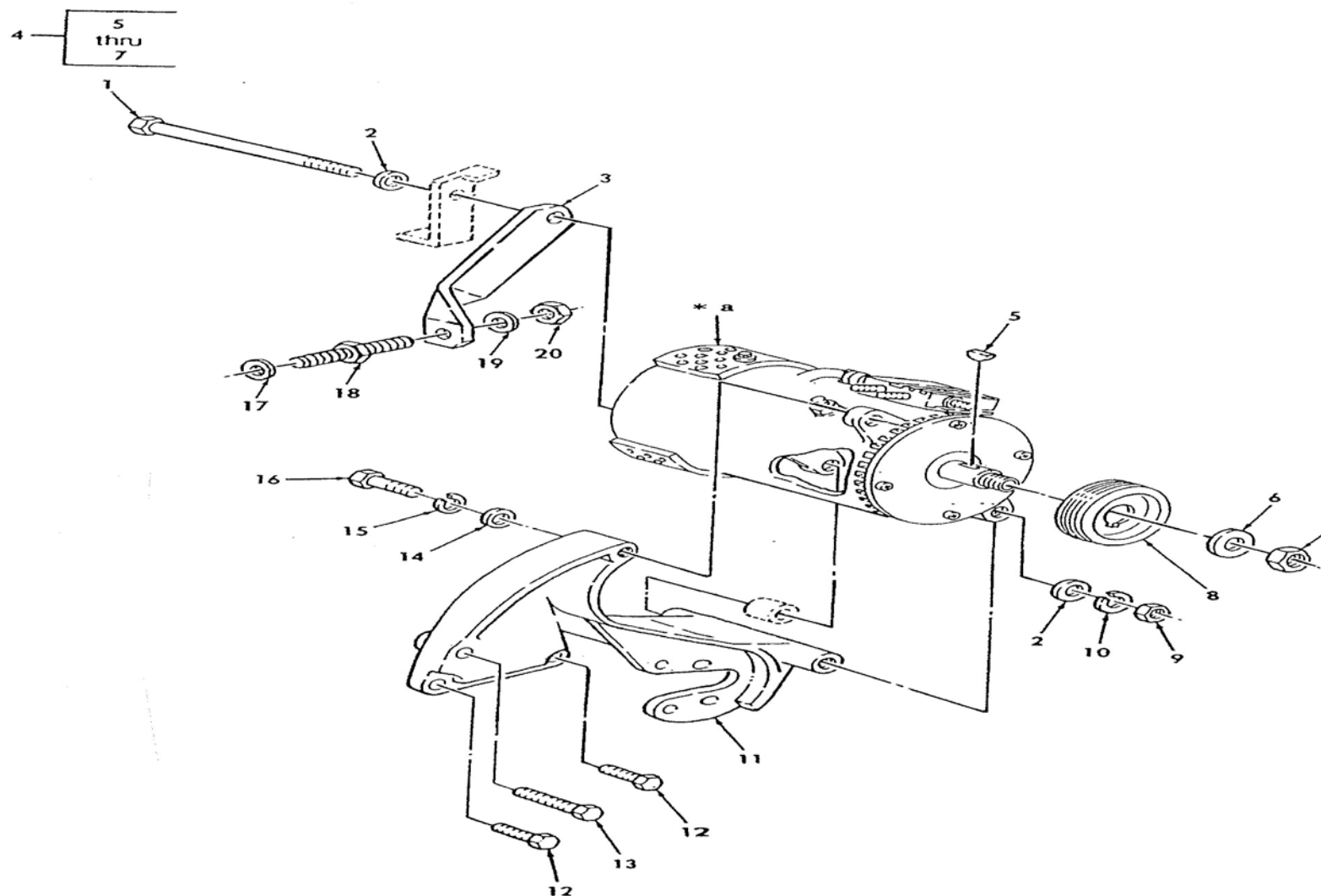
ภาพที่ 30 เครื่องกำเนิดไฟฟ้า 100 แอมแปร์
