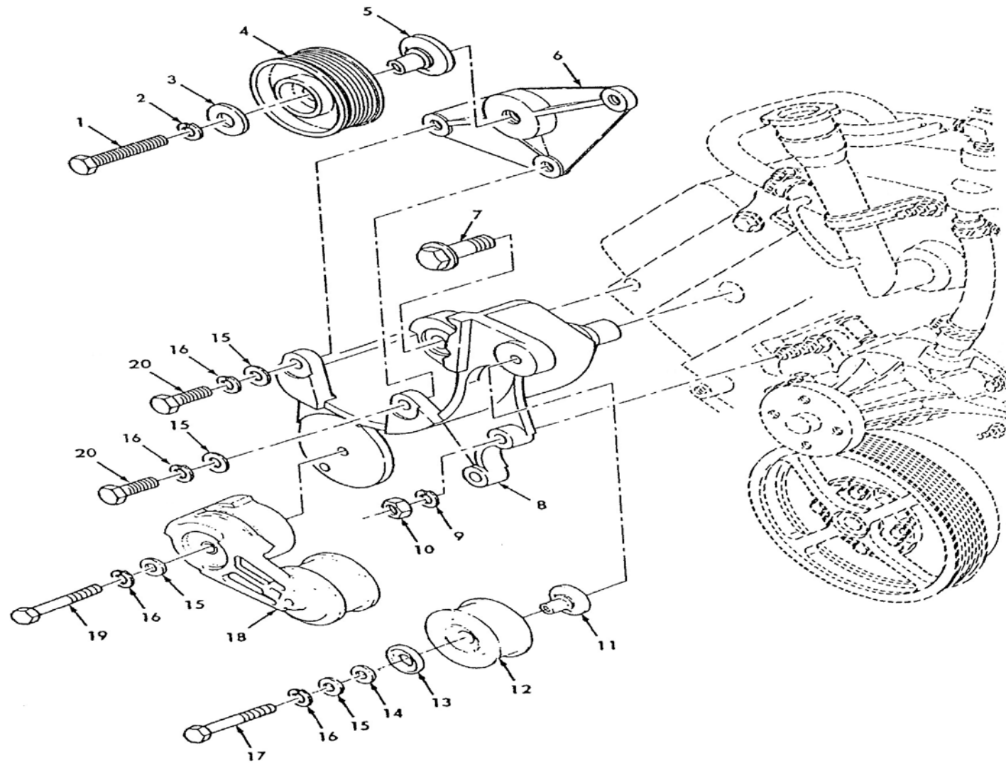
ภาพที่ 25 ชุดพูลเลย์ปรับจังหวะเดินเบา (1)
