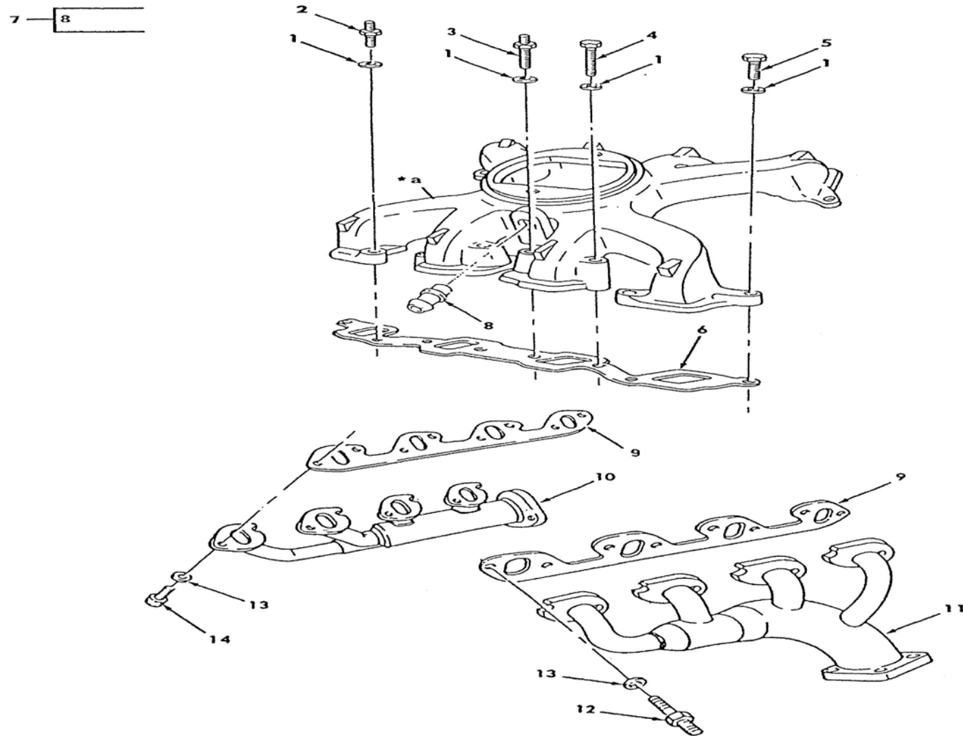
ภาพที่ 8 ชุดท่อร่วมไอดีและไอเสีย
