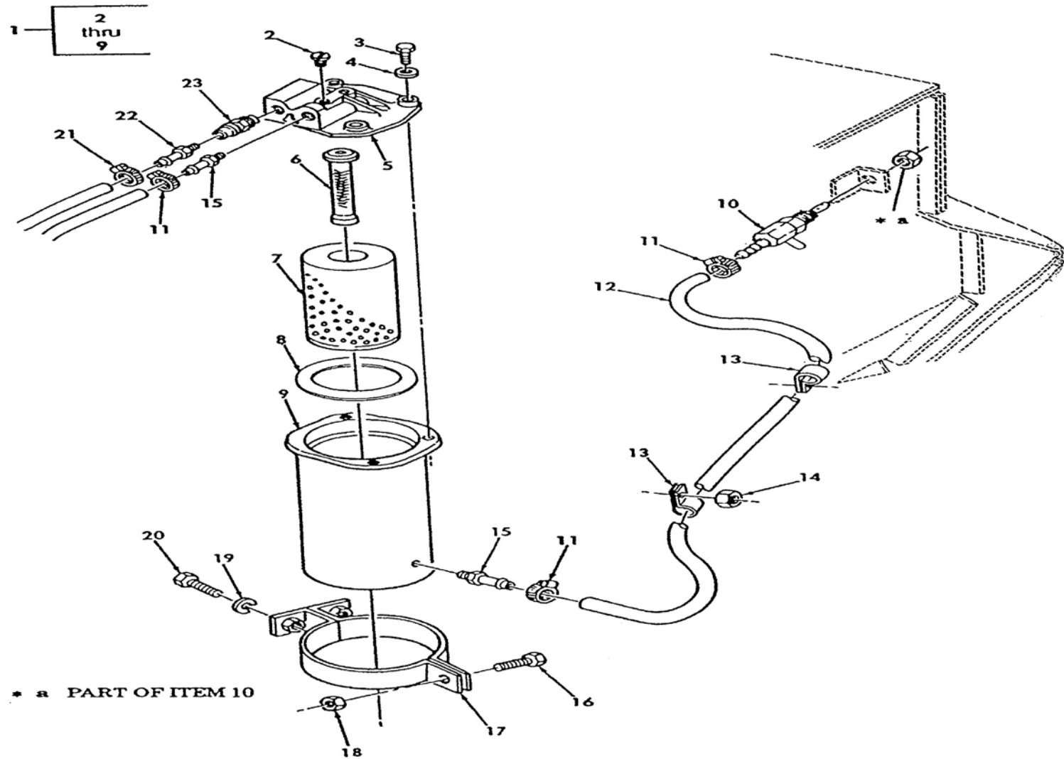
ภาพที่ 16 ชุดกรองเชื้อเพลิงและกรองตักน้ำ
