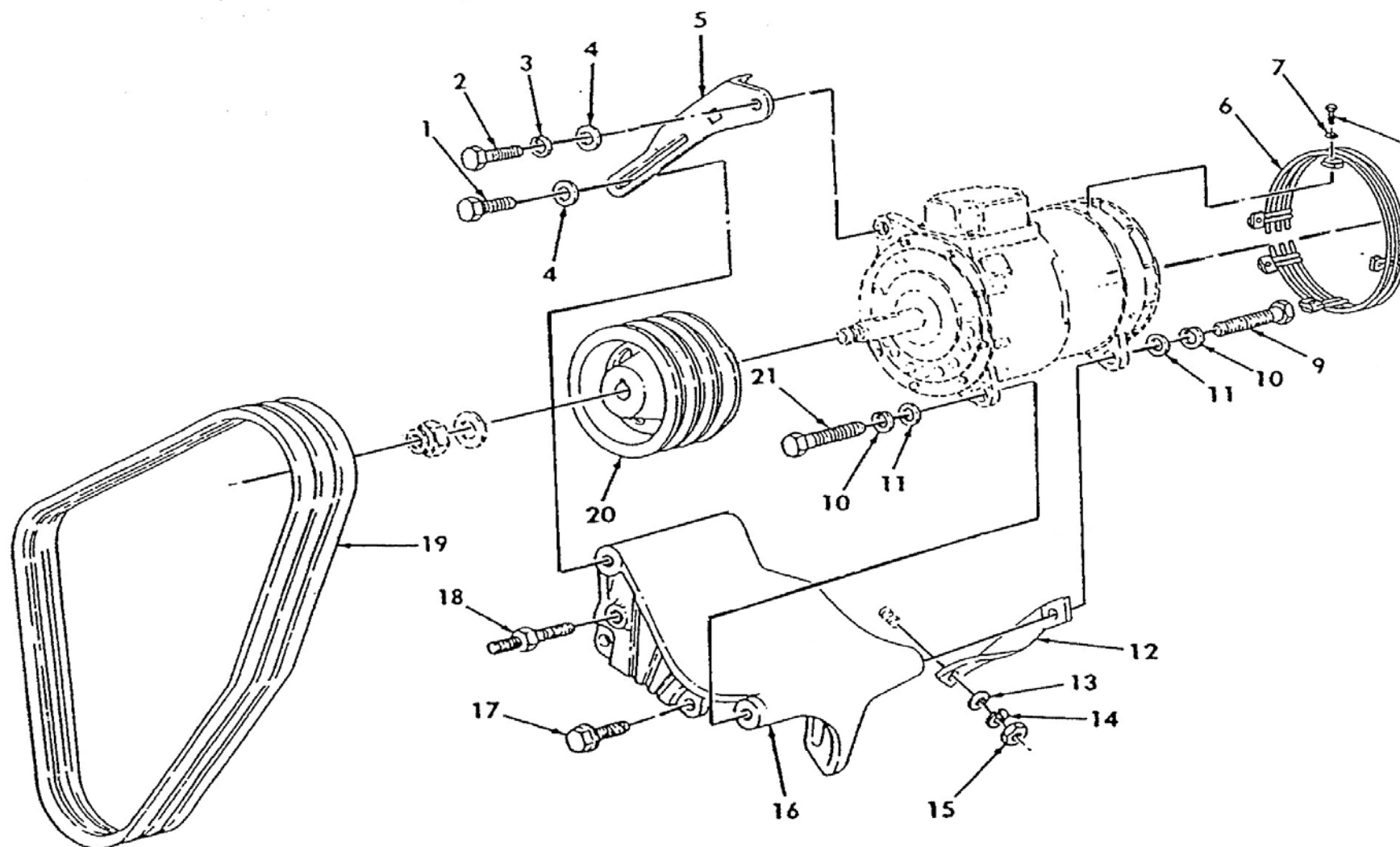
ภาพที่ 31 เครื่องกำเนิดไฟฟ้า 200 แอมแปร์
