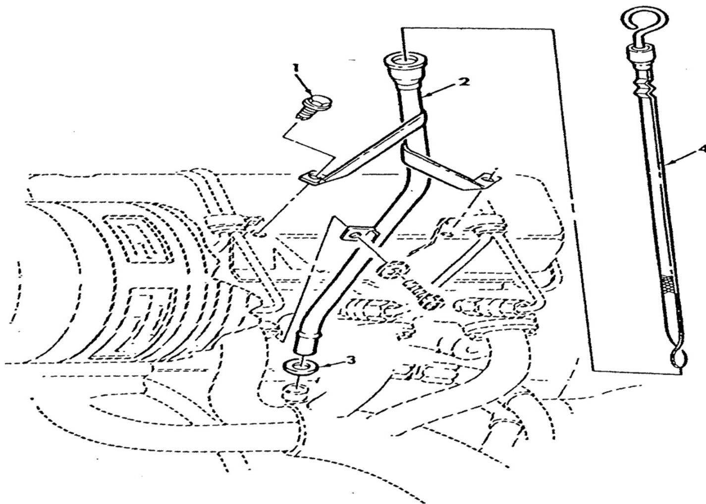
ภาพที่ 3 ชุดเหล็กวัดระดับน้ำมันเครื่อง
