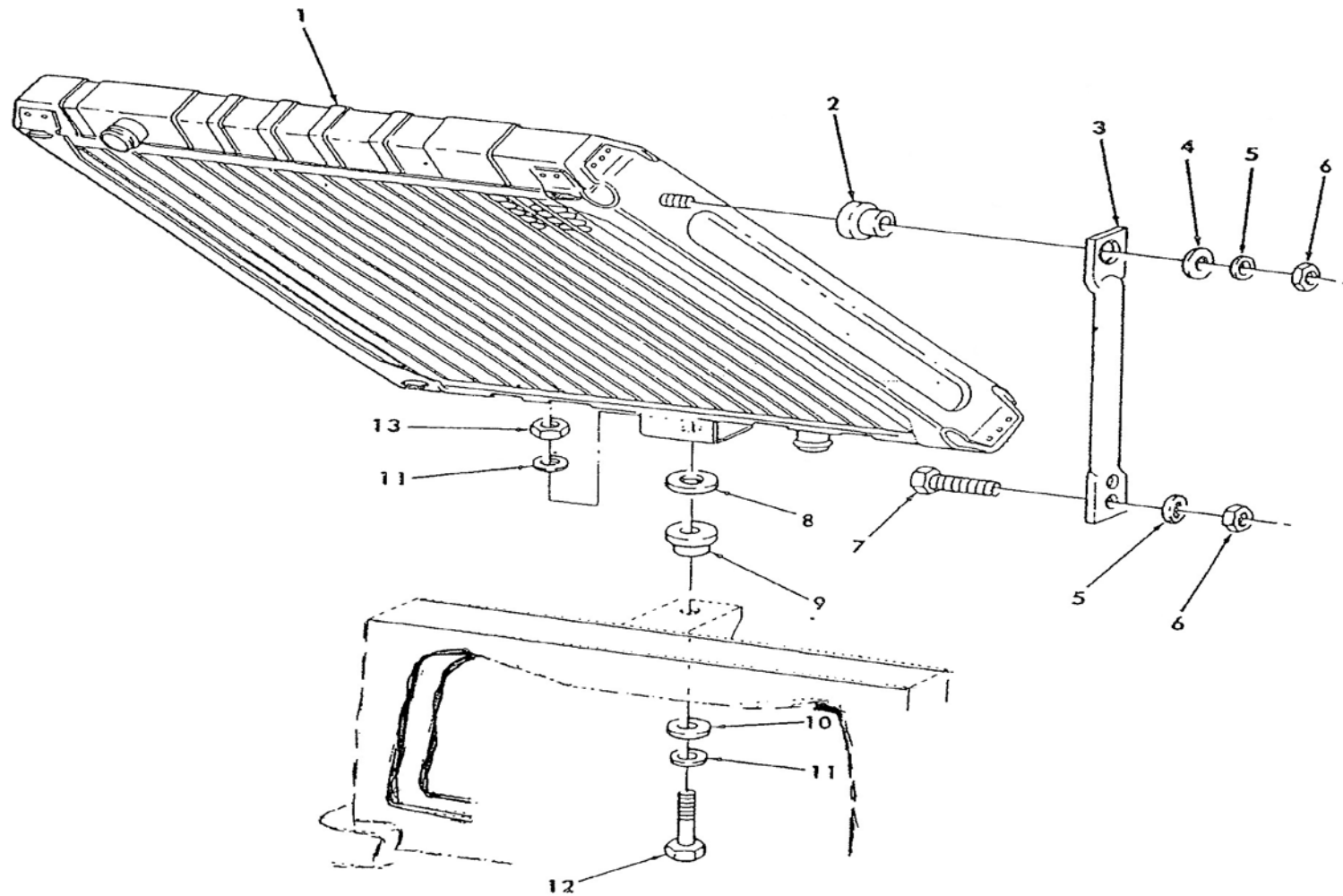
ภาพที่ 19 ชุดหม้อน้ำ
