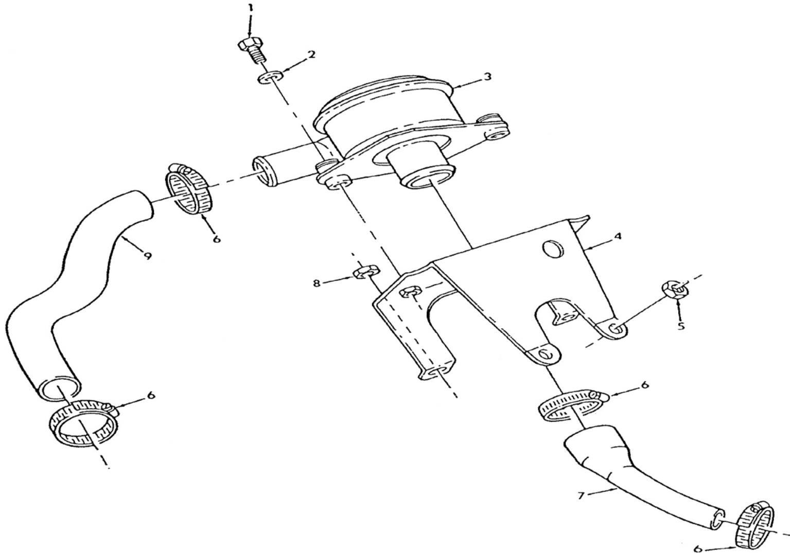
ภาพที่ 7 ชุดปรับแรงดันห้องข้อเหวี่ยง
