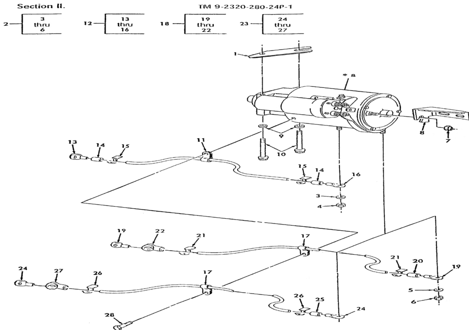
ภาพที่ 43 ชุดสายไฟมอเตอร์สตาร์ท
