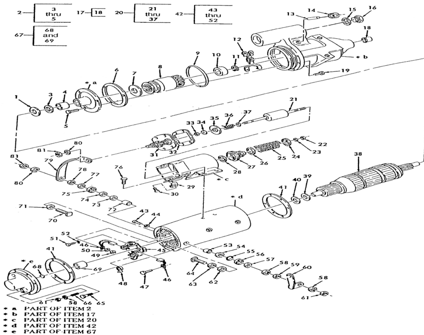
ภาพที่ 44 ชุดมอเตอร์สตาร์ท
