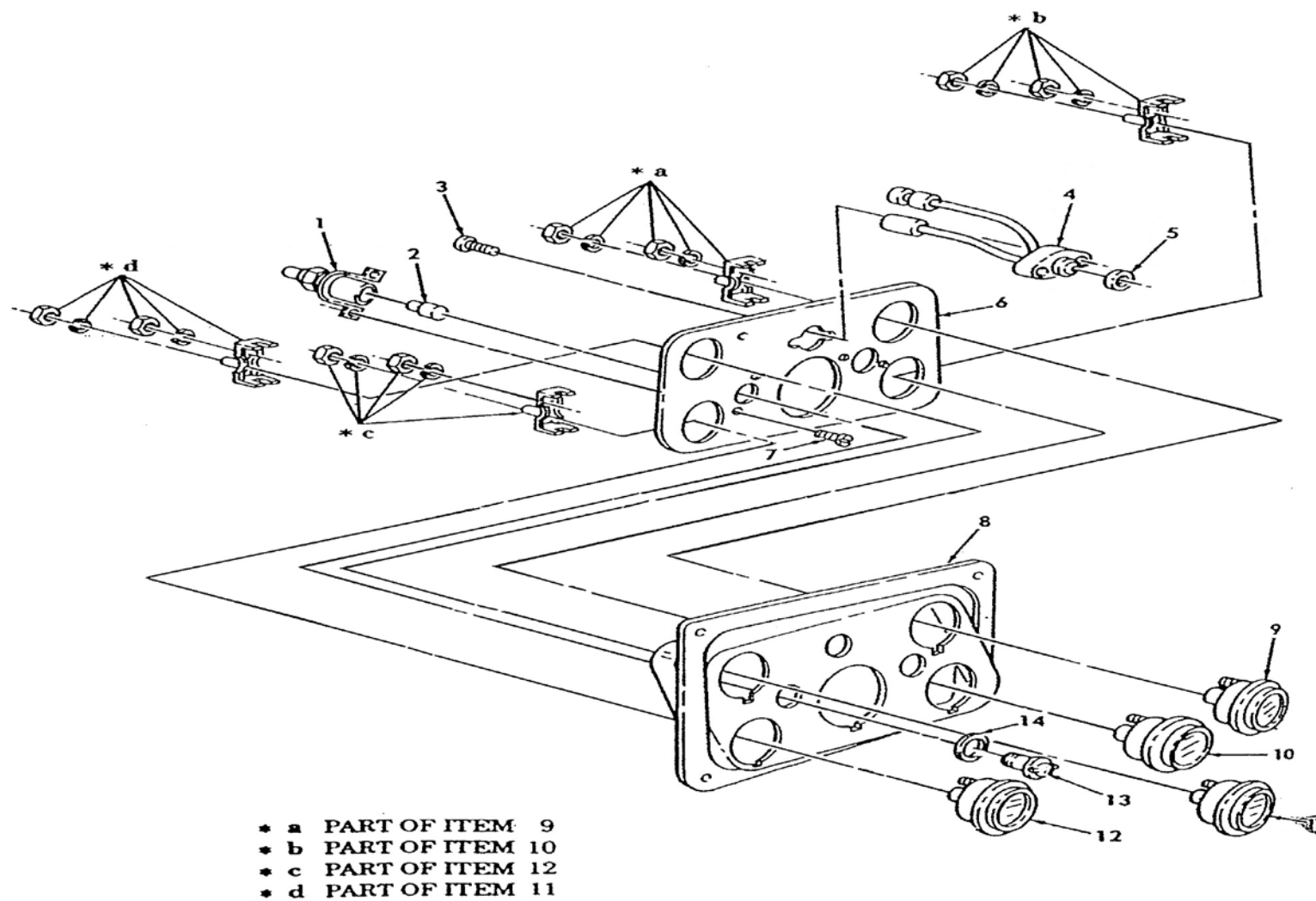
ภาพที่ 46 ชุดมาตรวัด
