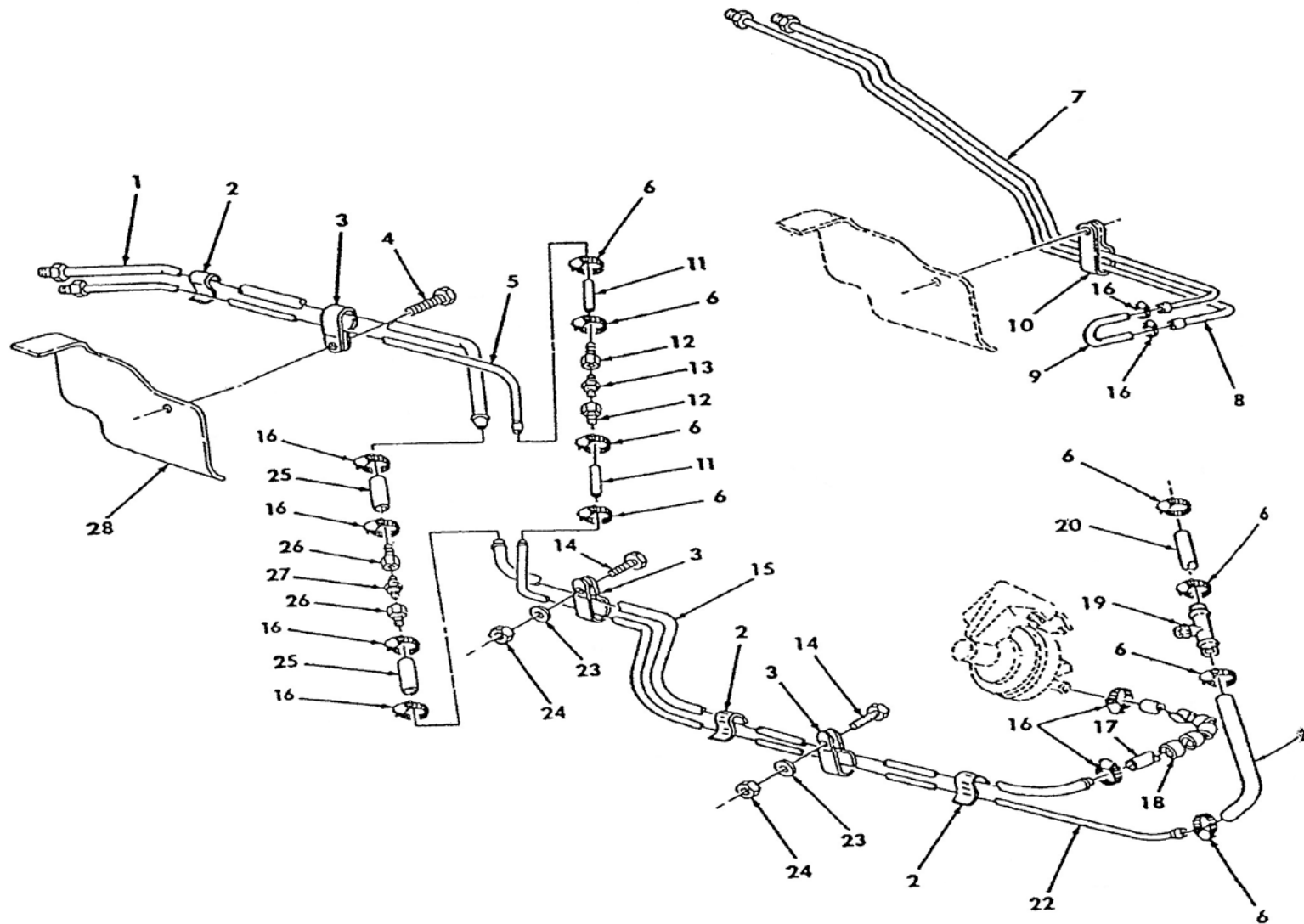
ภาพที่ 13 ชุดท่อเชื้อเพลิง
