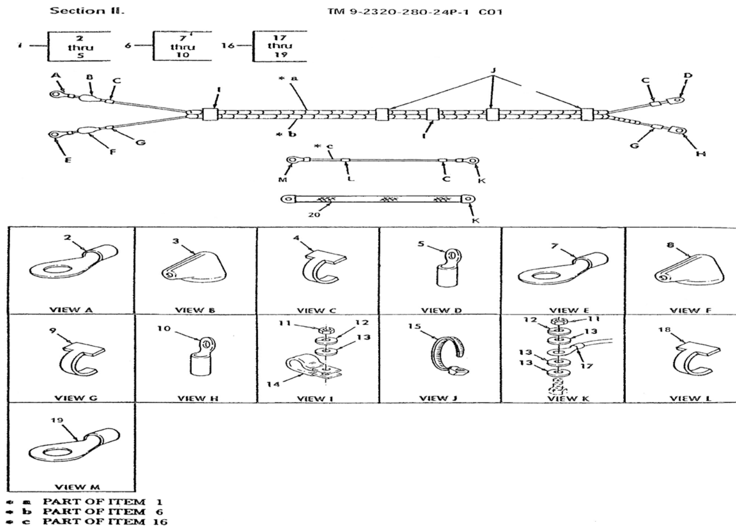
ภาพที่ 38 ชุดสายไฟของเครื่องกำเนิดไฟฟ้า A2 12 โวลต์ และ 24 โวลต์
