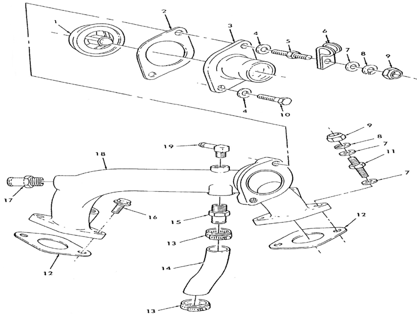
ภาพที่ 22 ชุดเทอร์โมสแตท
