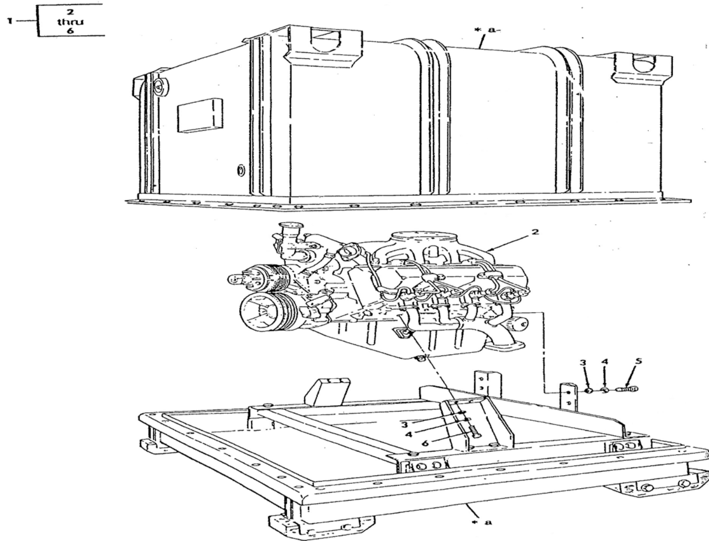
ภาพที่ 1 เครื่องยนต์และเหล็กบรรจุ สป.
