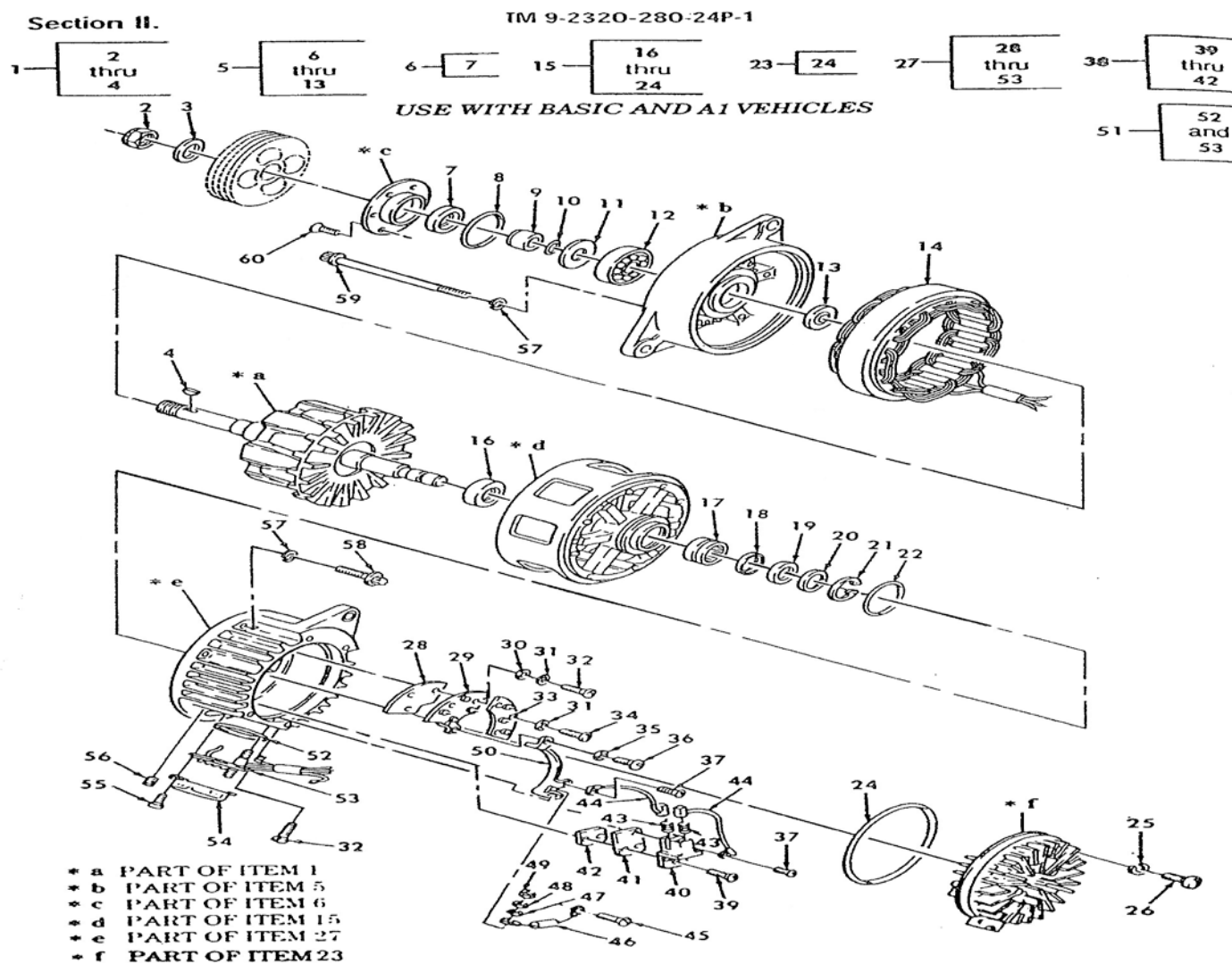
ภาพที่ 40 ชุดเครื่องกำเนิดไฟฟ้า 60/100 และ 200 แอมแปร์
