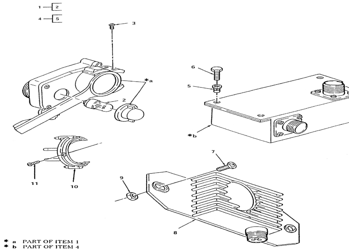
ภาพที่ 47 ชุดไฟเลี้ยว
