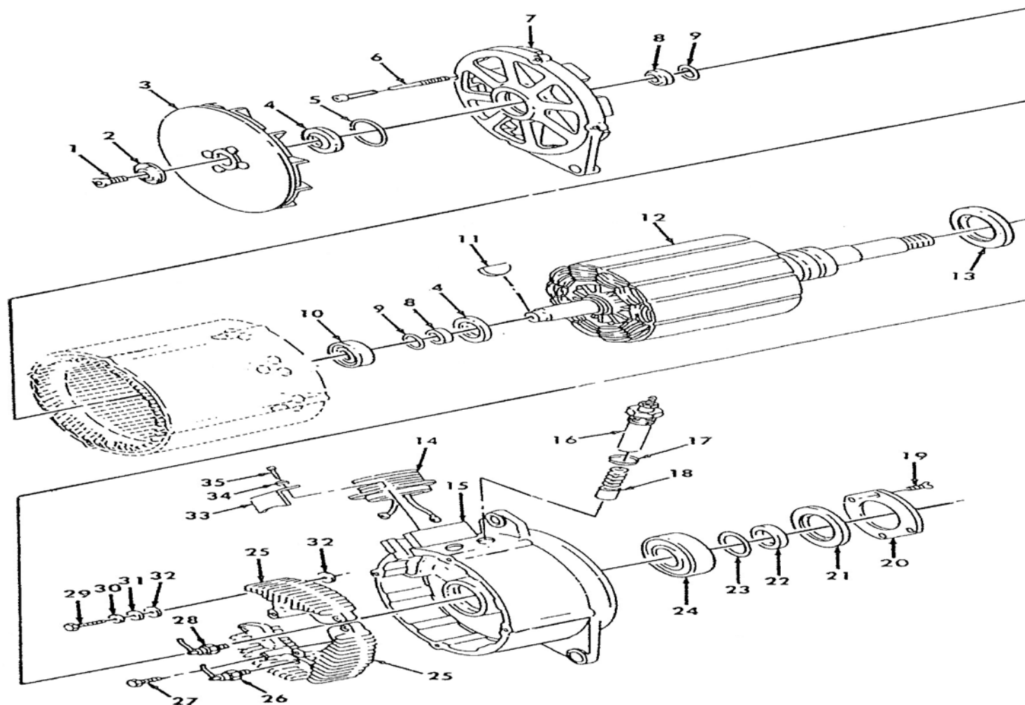
ภาพที่ 41 ชุดเครื่องกำเนิดไฟฟ้า ขนาด 100 แอมแปร์
