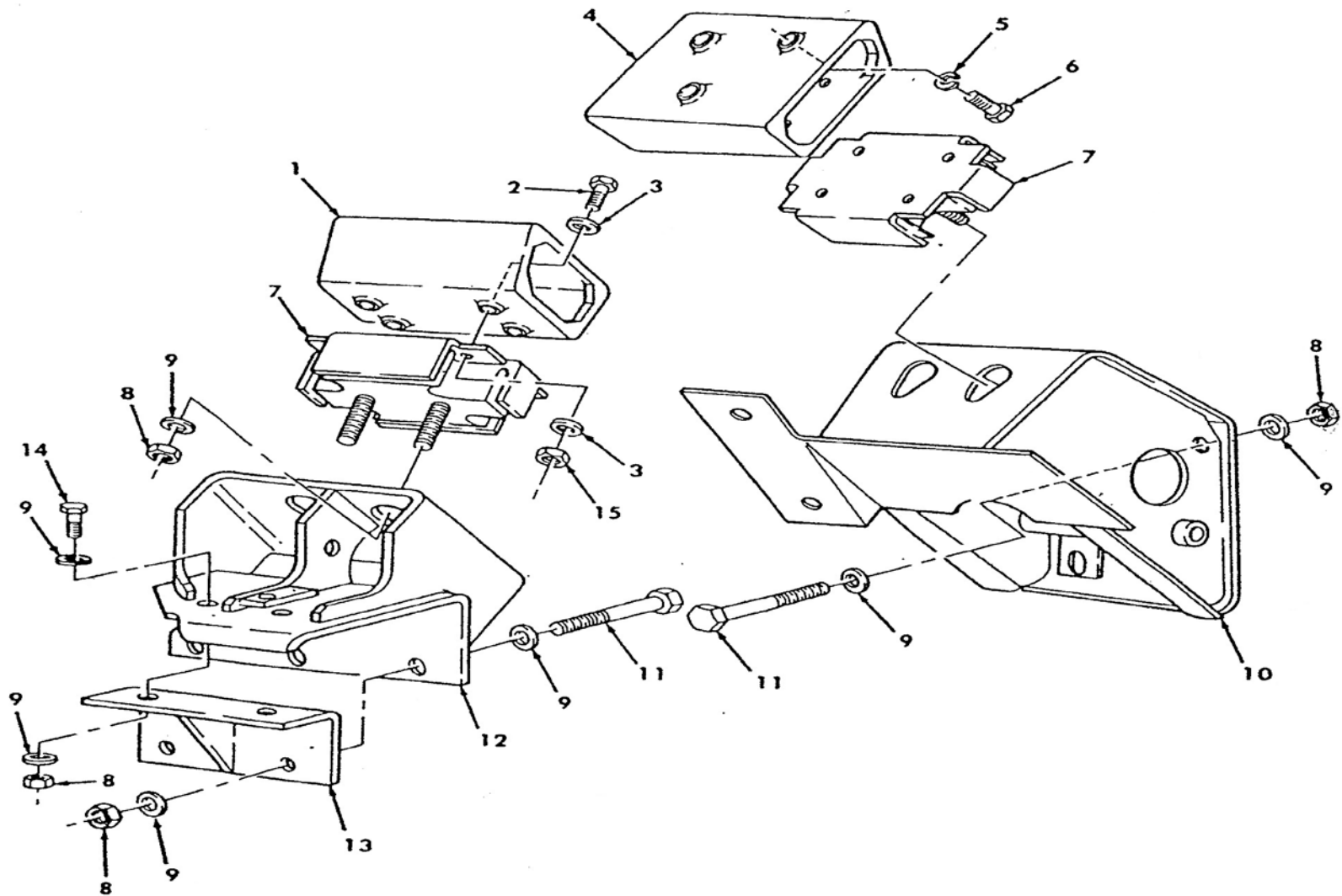
ภาพที่ 2 ชุดแผ่นฐานรองแท่นเครื่องยนต์
