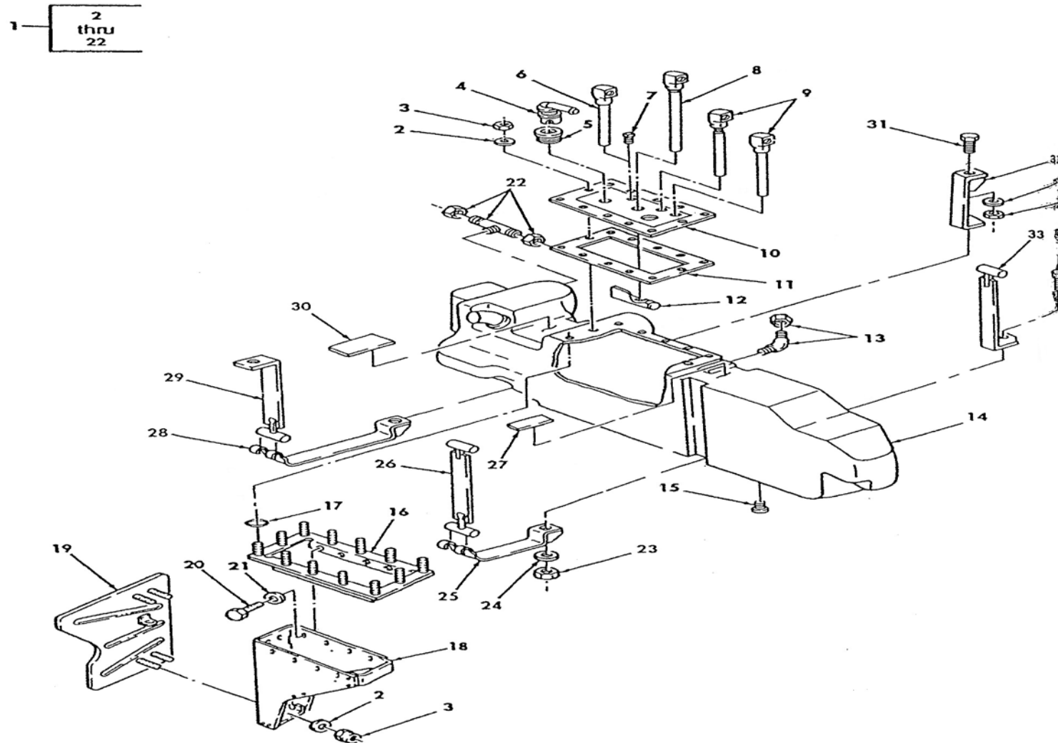
ภาพที่ 14 ชุดถังเชื้อเพลิง
