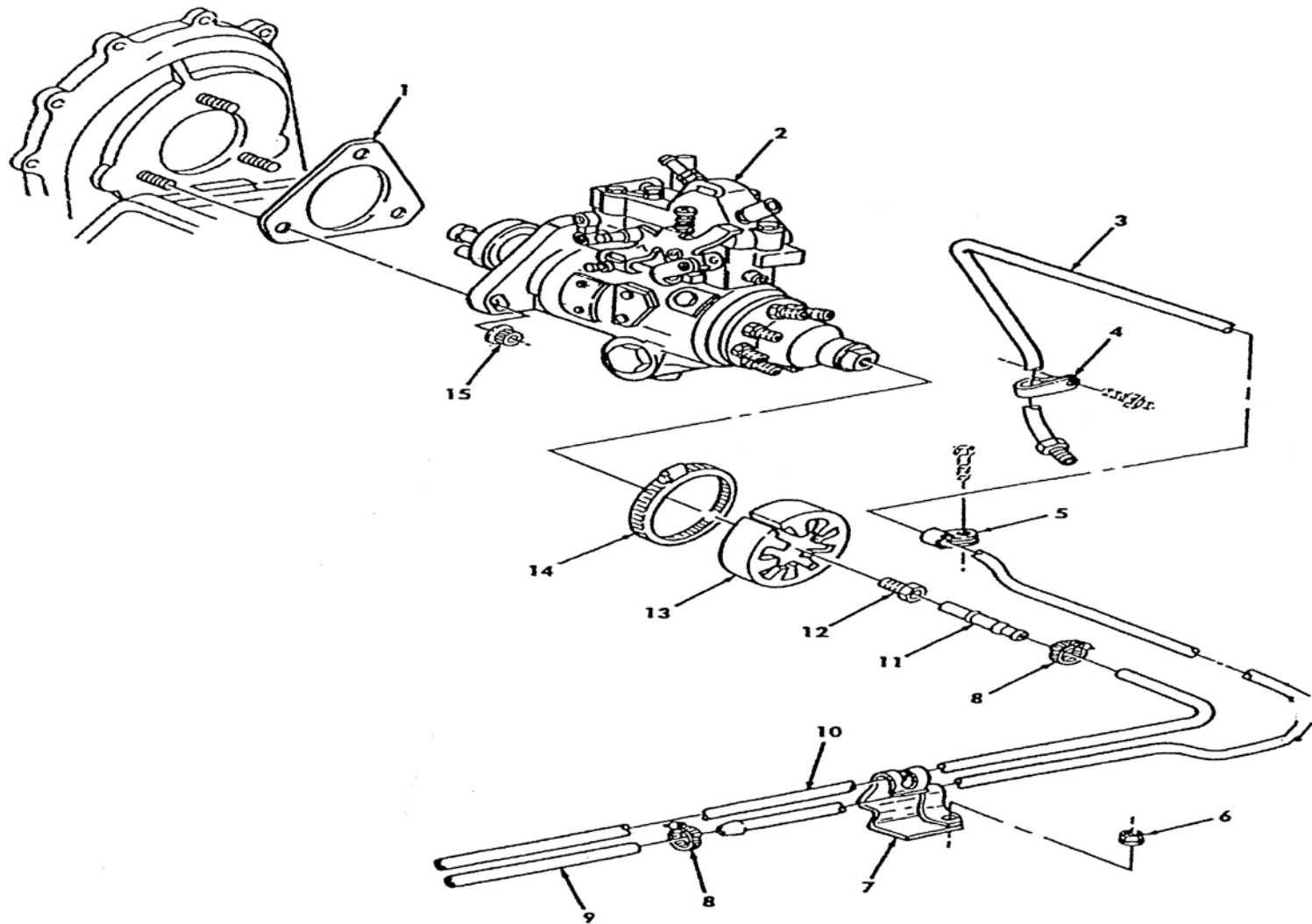
ภาพที่ 10 ชุดปั๊มสูบน้ำเชื้อเพลิง
