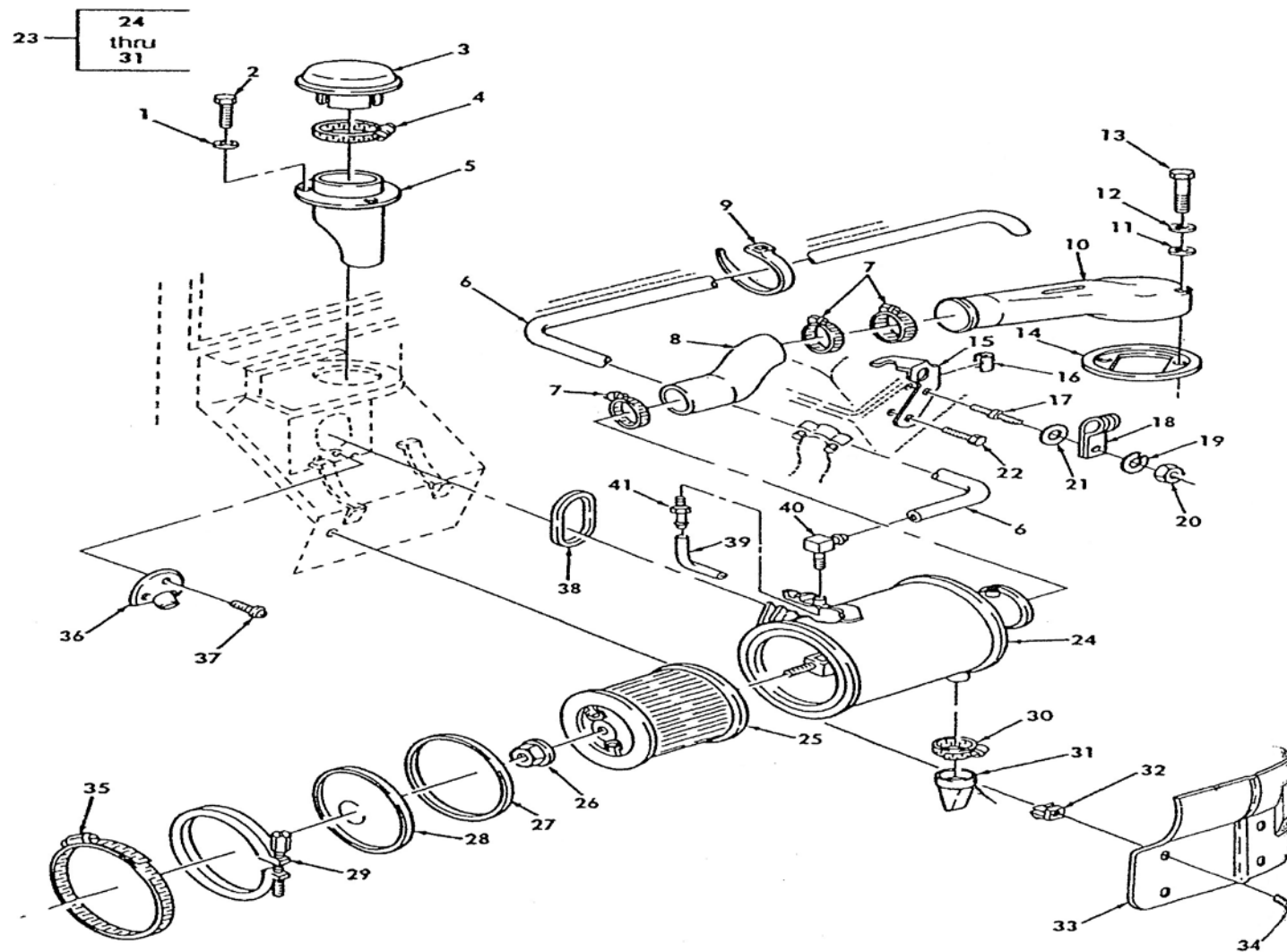
ภาพที่ 11 ชุดกรองอากาศ
