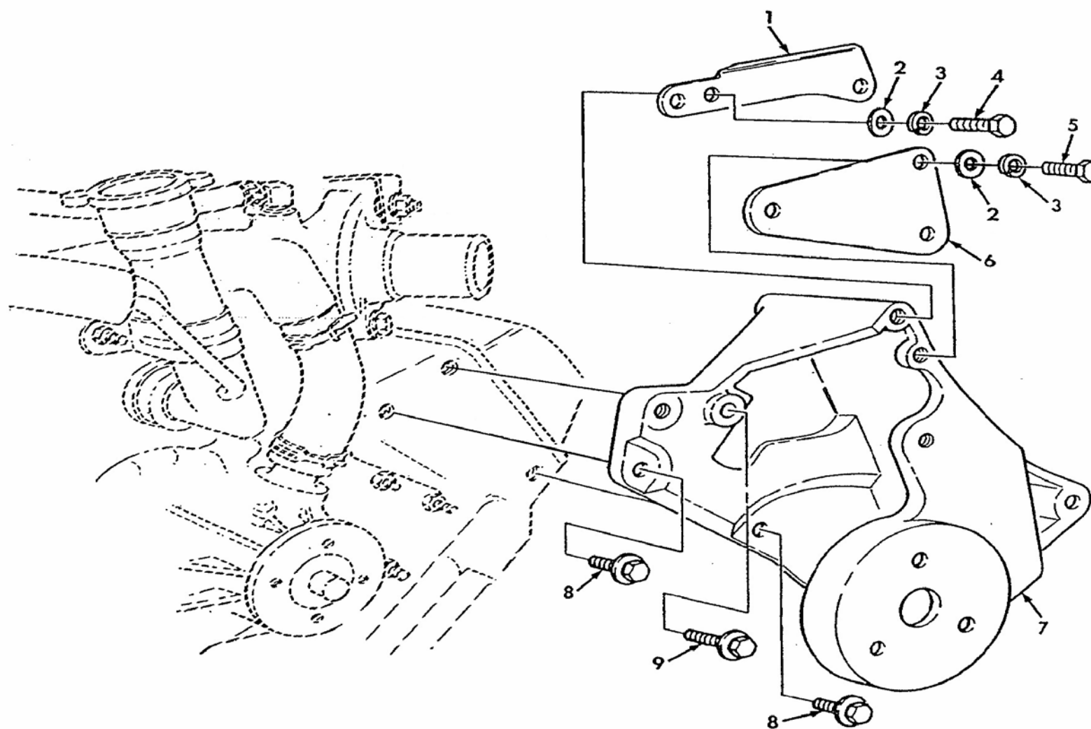
ภาพที่ 33 ชุดแผ่นฐานรองเครื่องกำเนิดไฟฟ้าปั้มบังคับเลี้ยวแบบเพาเวอร์
