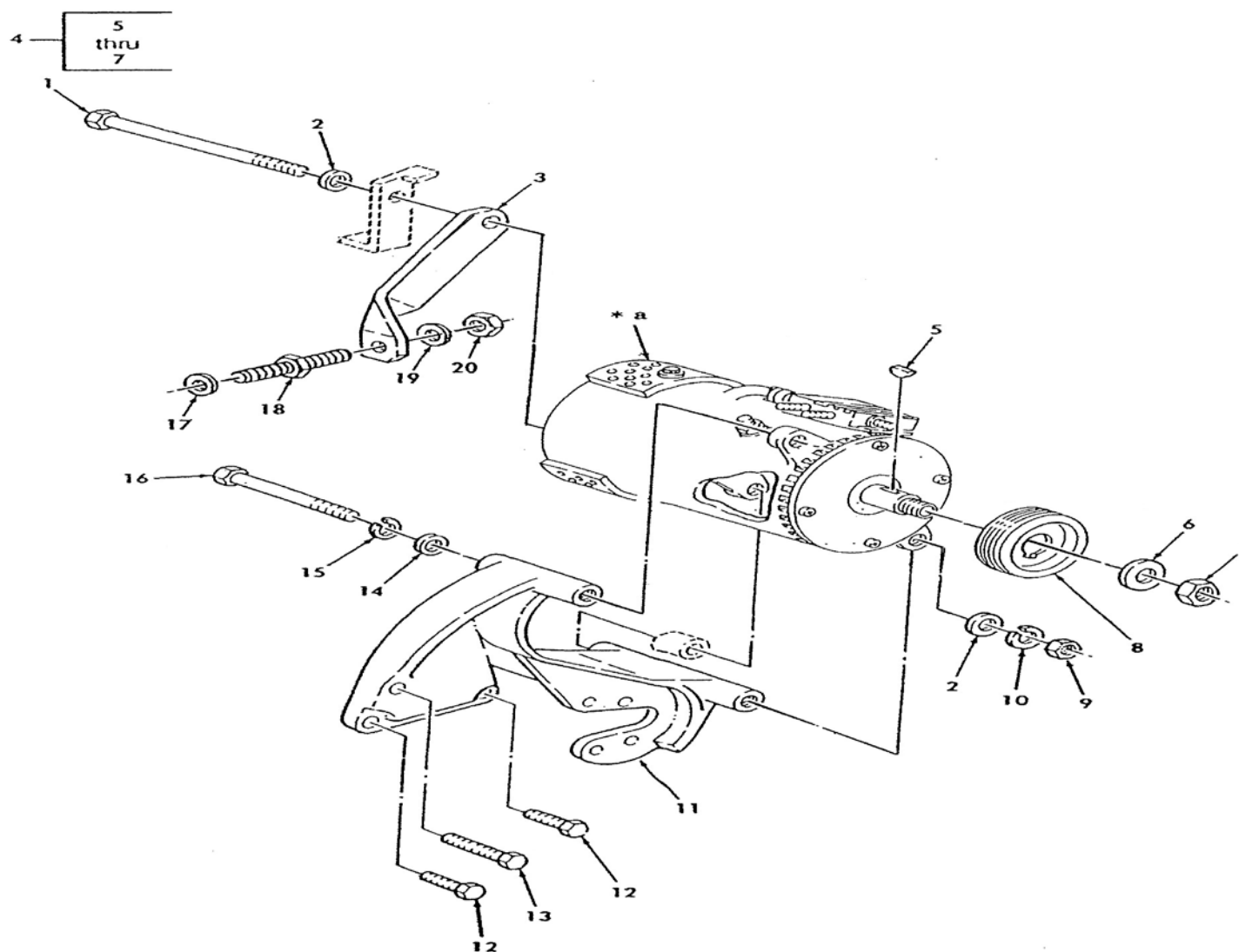
ภาพที่ 32 เครื่องกำเนิดไฟฟ้า 200 แอมแปร์
