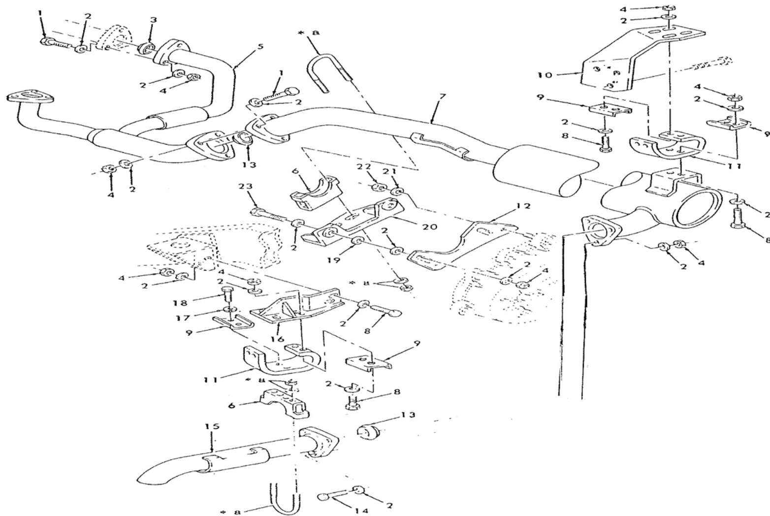
ภาพที่ 18 ชุดท่อไอเสีย
