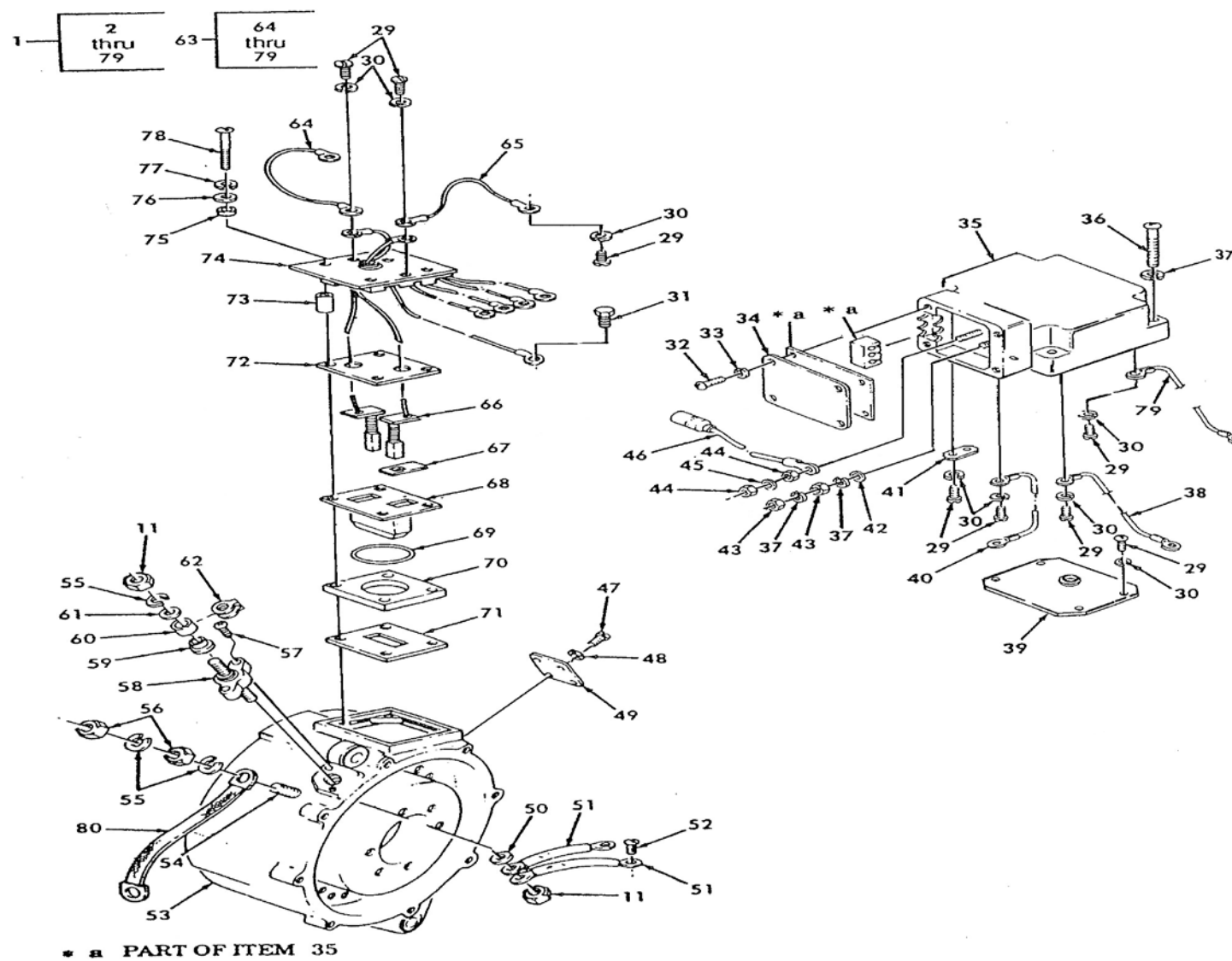
ภาพที่ 35 เครื่องกำเนิดไฟฟ้า ขนาด 200 แอมแปร์ (2)
