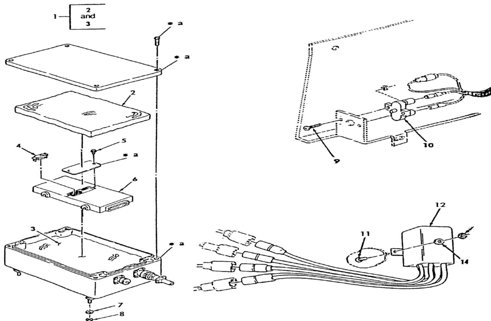
ภาพที่ 48 ชุดควบคุมการทำงานของเกียร์
