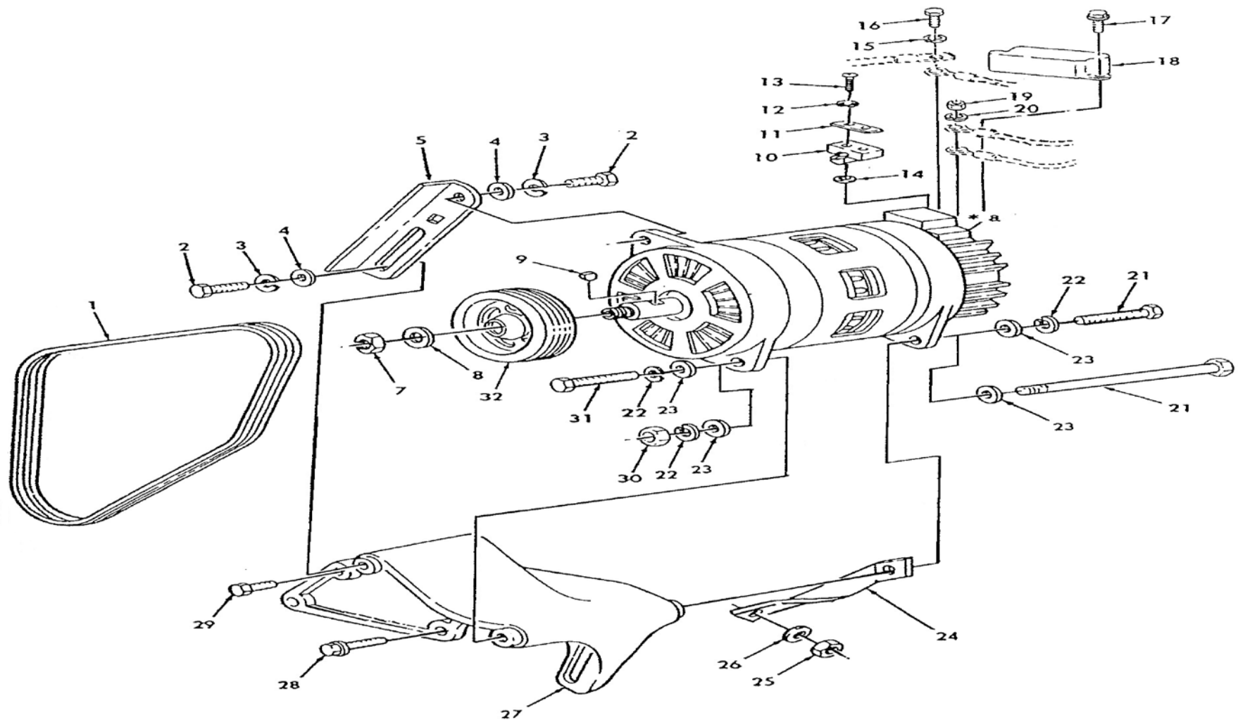
ภาพที่ 28 เครื่องกำเนิดไฟฟ้า 60 แอมแปร์
