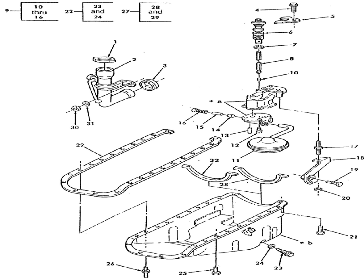
ภาพที่ 4 ชุดอ่างน้ำมันเครื่อง
