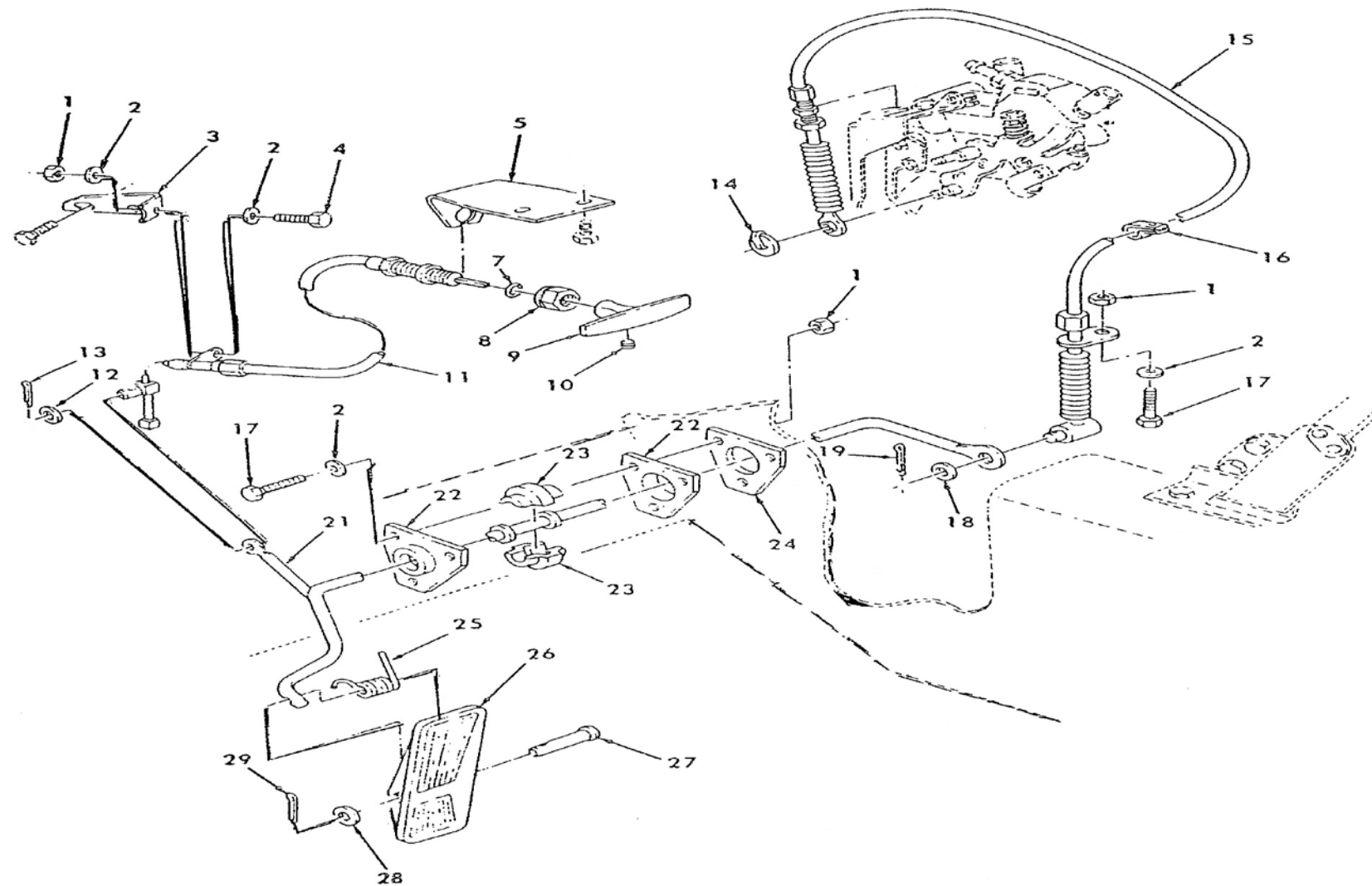
ภาพที่ 17 ชุดคันเร่ง
