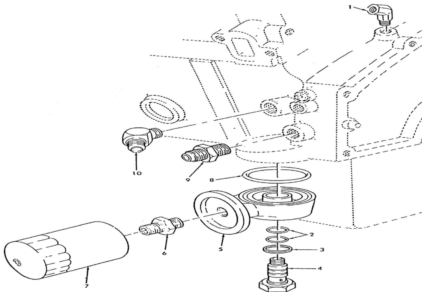
ภาพที่ 6 ชุดกรองน้ำมันเครื่อง
