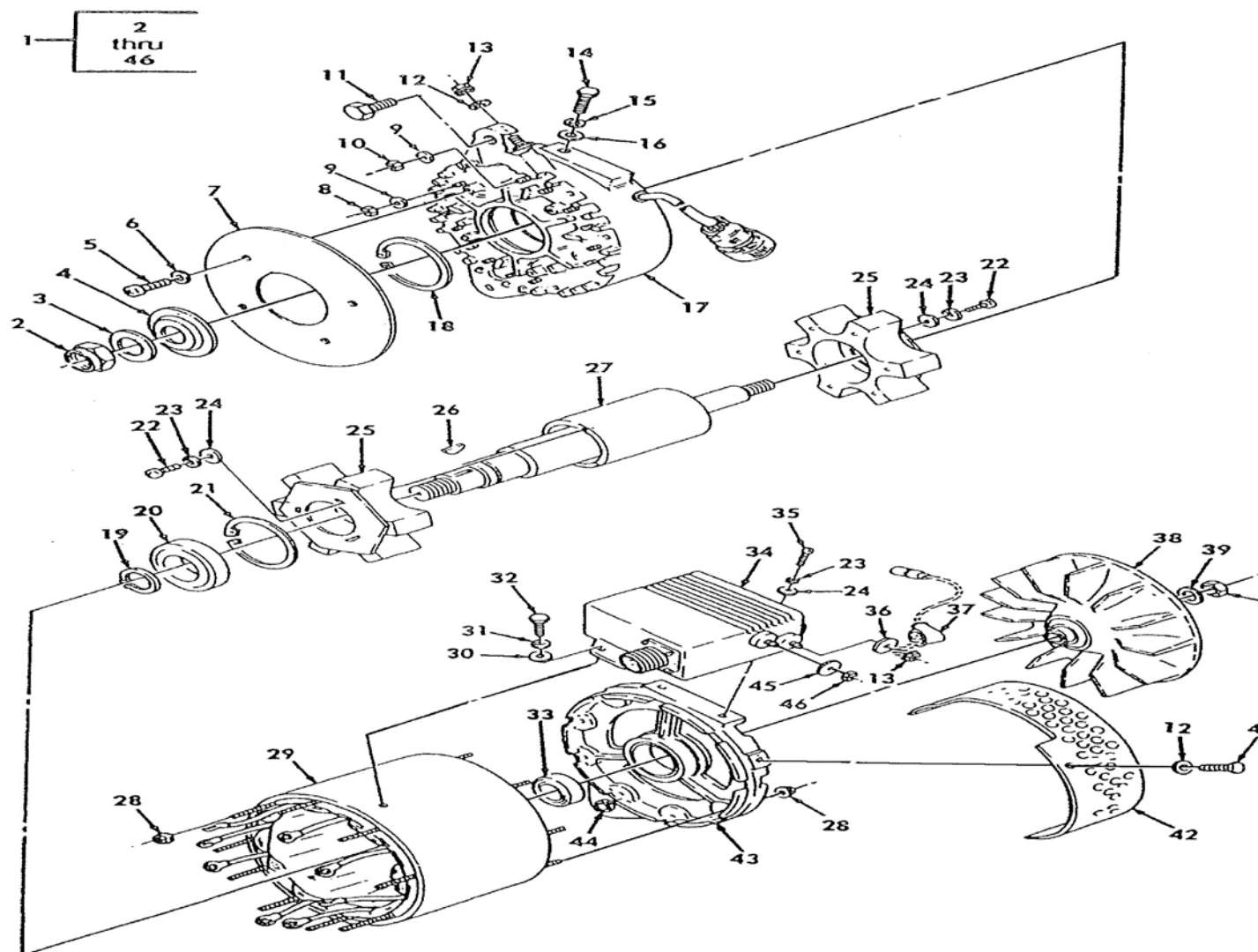
ภาพที่ 42 ชุดเครื่องกำเนิดไฟฟ้า ขนาด 100 แอมแปร์
