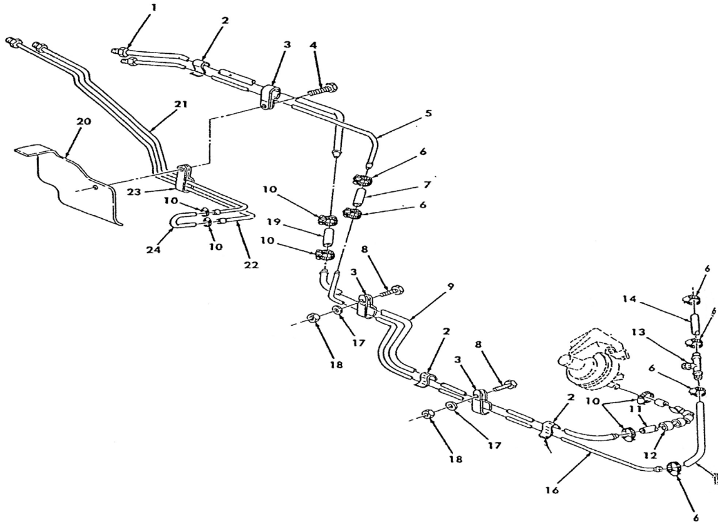
ภาพที่ 12 ชุดท่อเชื้อเพลิง
