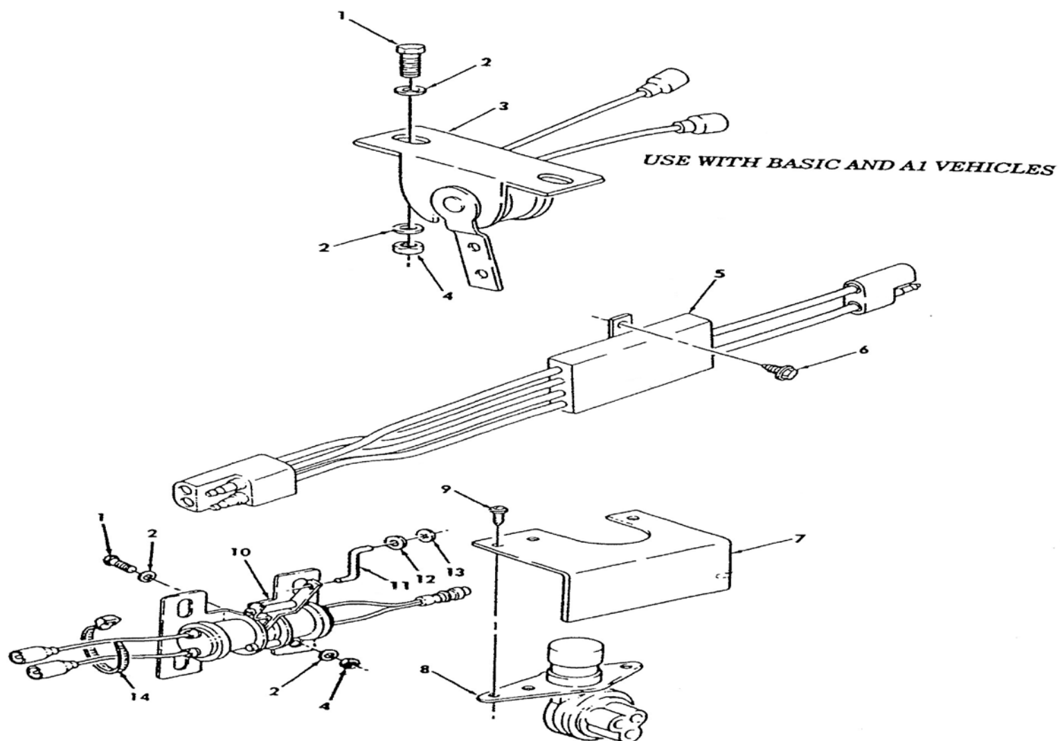
ภาพที่ 49 ชุดสวิตช์ไฟหยุดรถและสวิตช์ไฟสูง-ต่ำ
