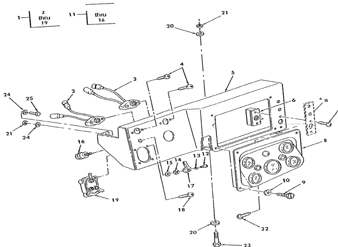
ภาพที่ 45 ชุดฐานยึดแผงเครื่องวัด
