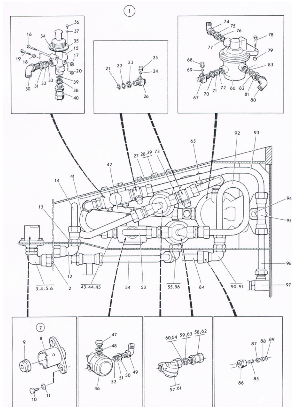
ภาพที่ 13 ชุดเบรกกลมครบชุด
