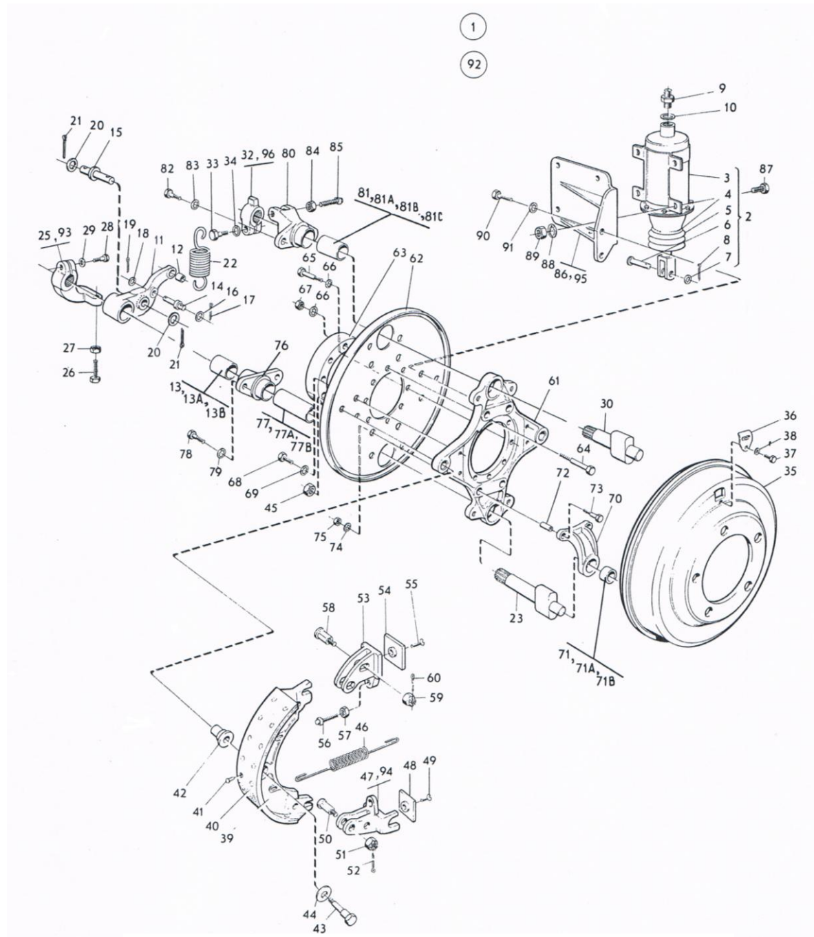
ภาพที่ 25 เบรกหลังด้านซ้ายครบชุด
