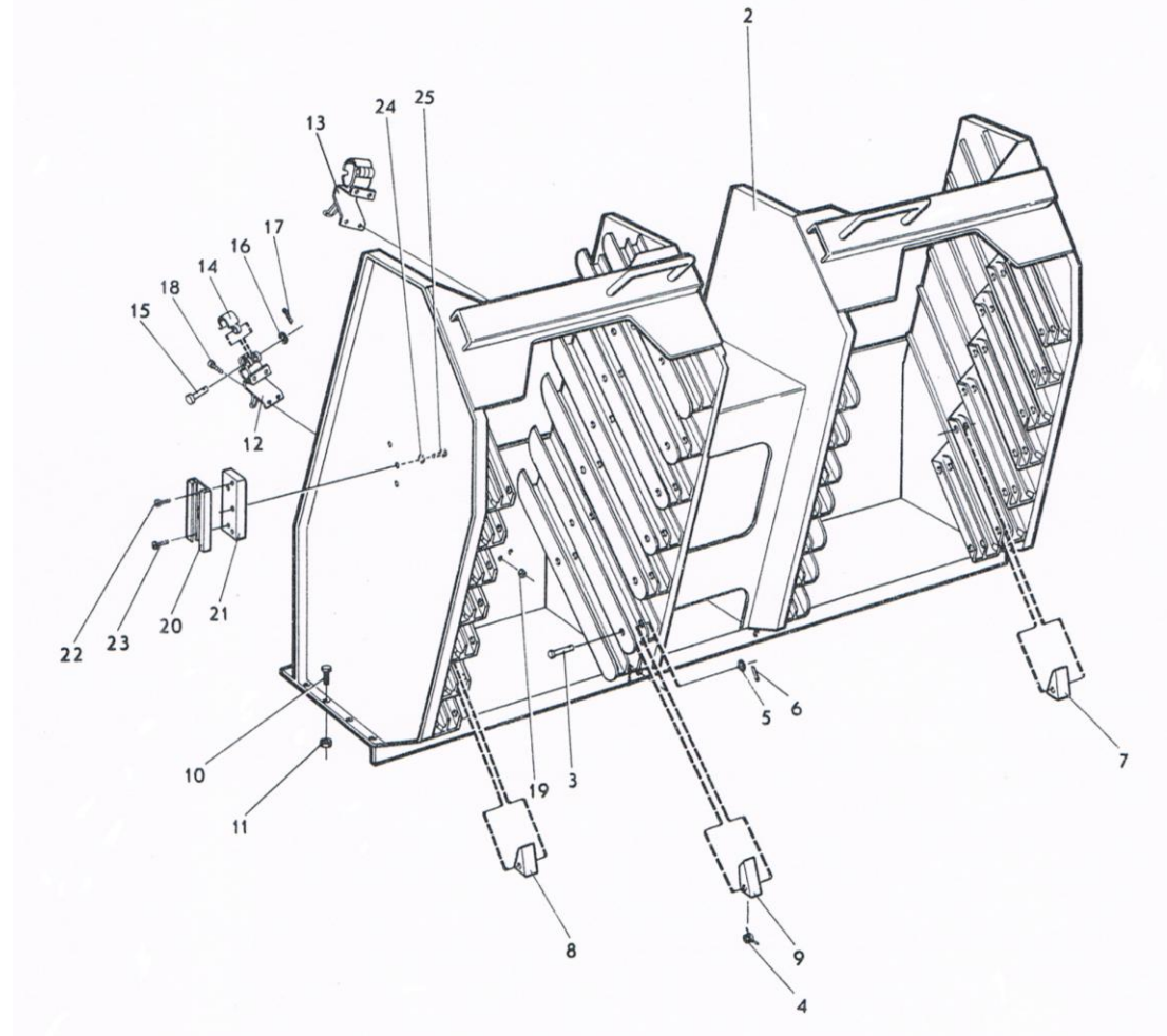
ภาพที่ 4 ร่างเก็บกระสุนครบชุด
