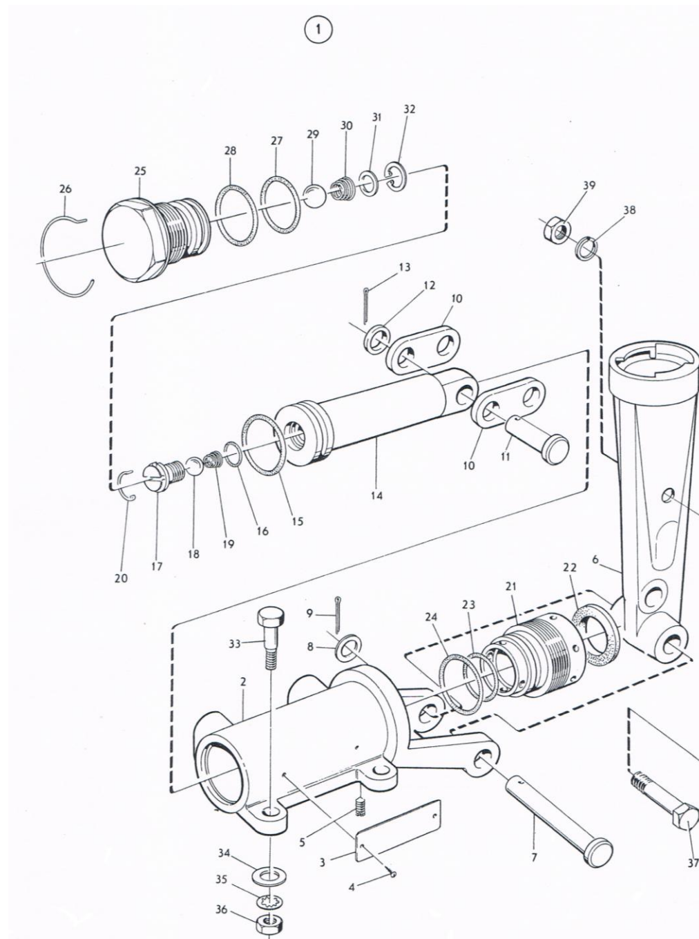
ภาพที่ 11 ชุดปั๊มครบชุด
