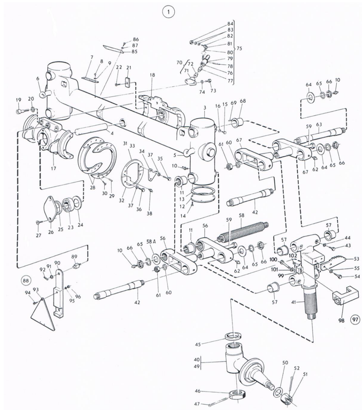
ภาพที่ 24 ชุดแกนเพลาลังครบชุด
