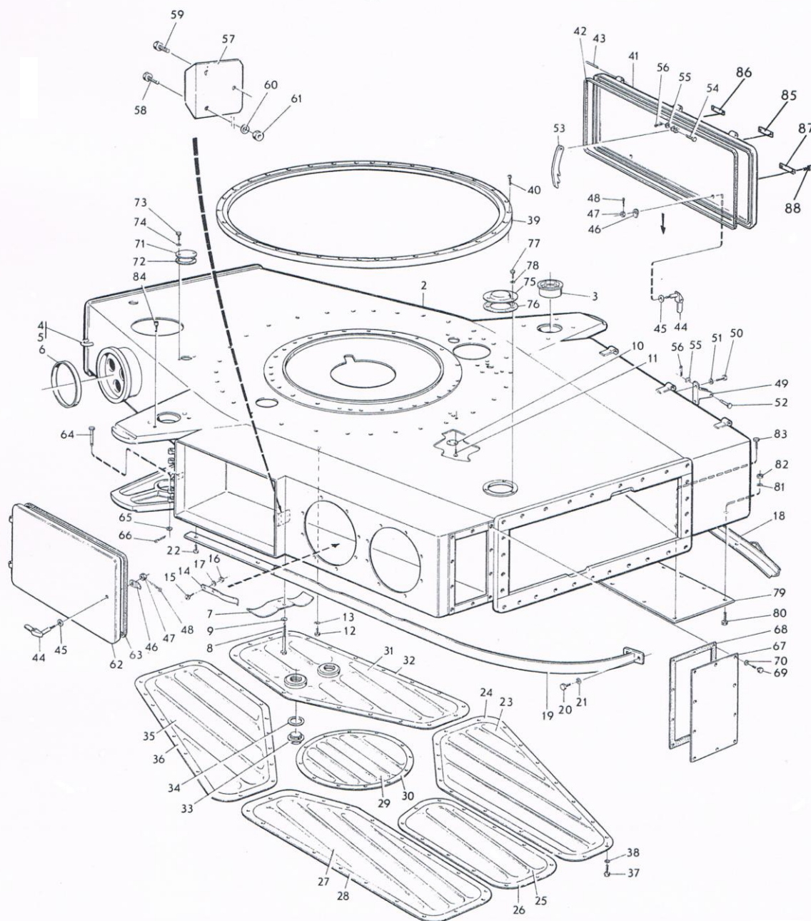
ภาพที่ 7 ชุดแครงกลางครบชุด
