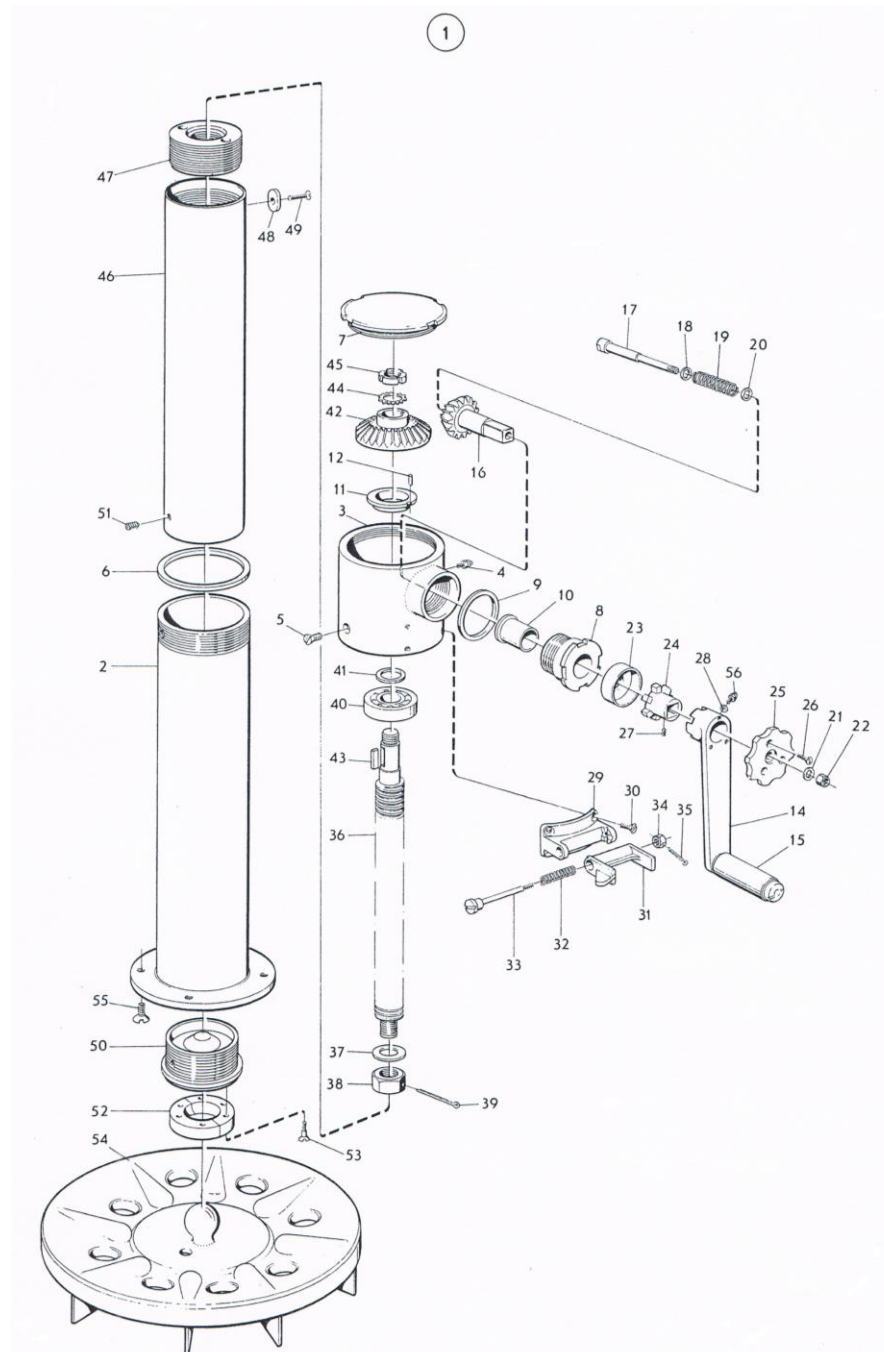
ภาพที่ 18 ชุดปรับระดับฐานปืนครบชุด
