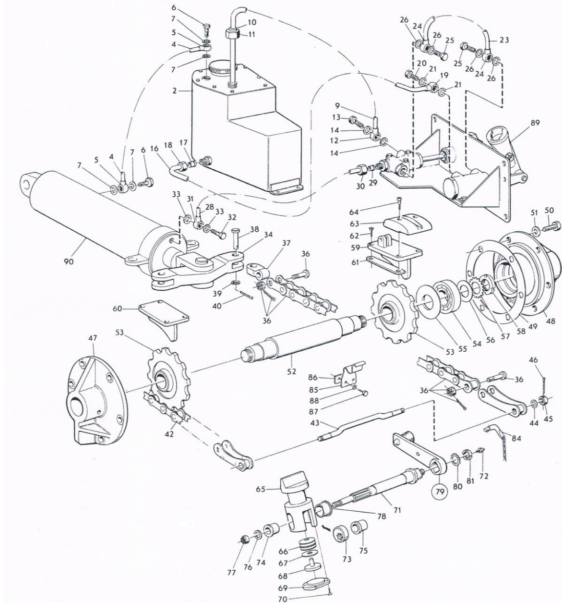
ภาพที่ 15 ชุดเฟืองยกเพลาลัง
