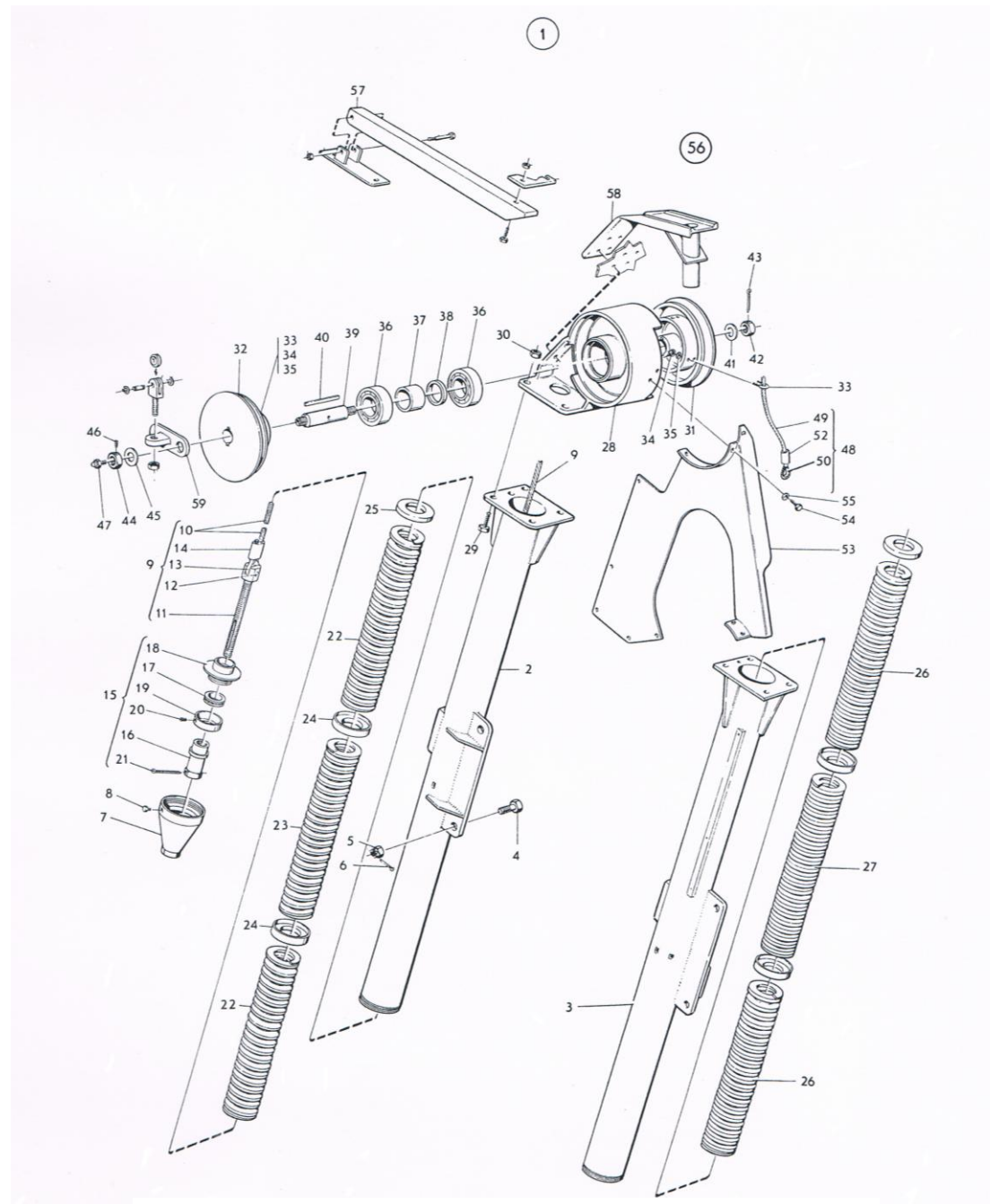
ภาพที่ 6 ชุดเครื่องช่วยทางสูงครบชุด
