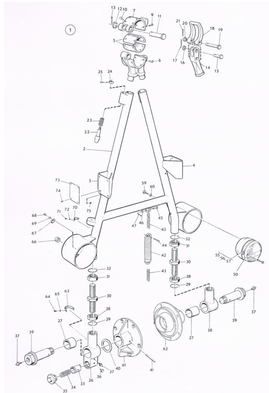
ภาพที่ 16 ชุดขายึดปีนครบชุด
