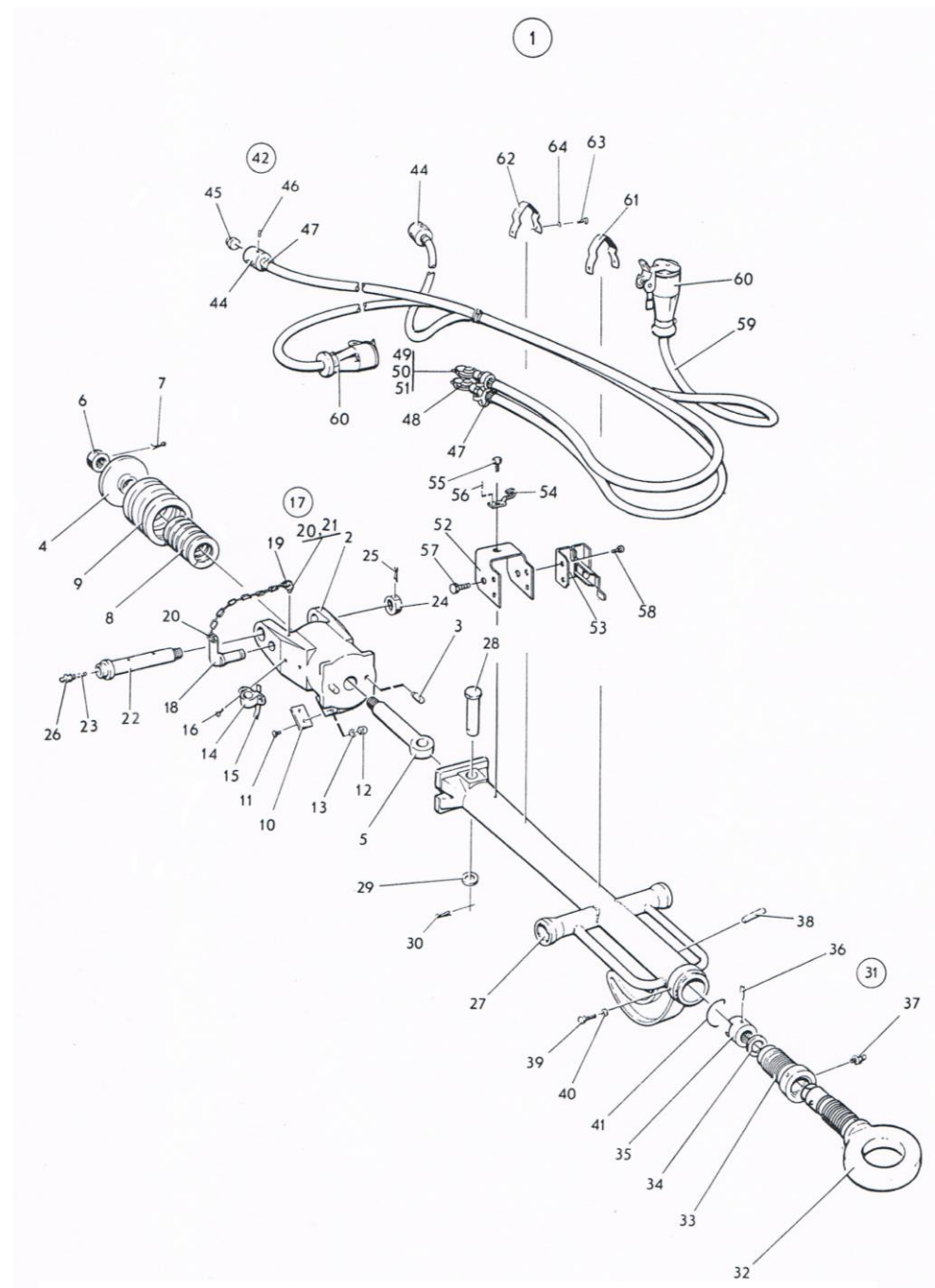
ภาพที่ 23 ห่วงลากจูงครบชุด
