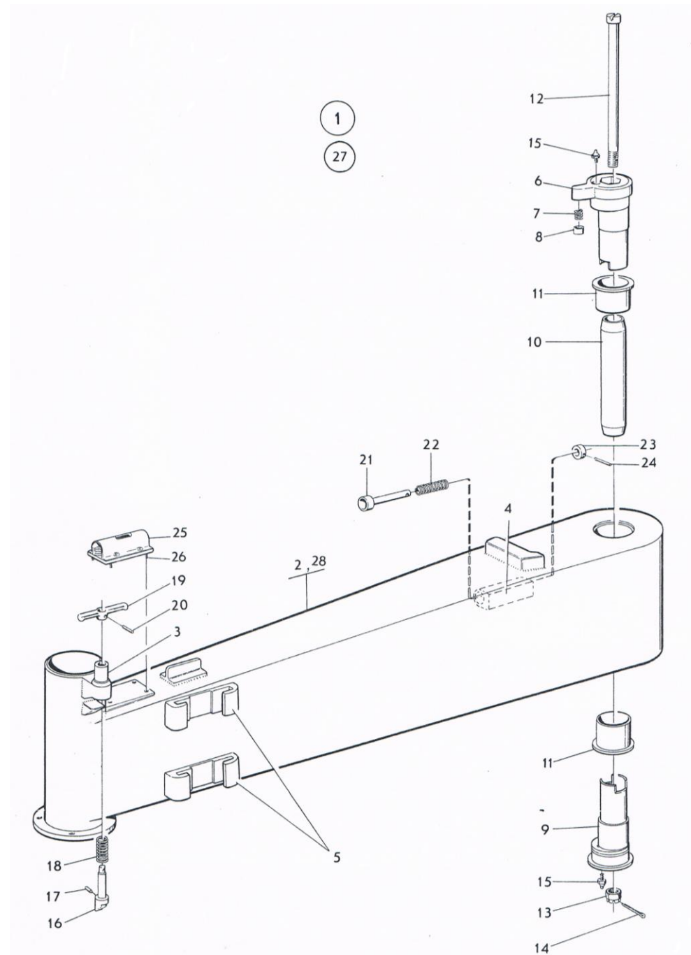
ภาพที่ 17 ชุดปั๊มภายนอกด้านซ้ายครบชุด
