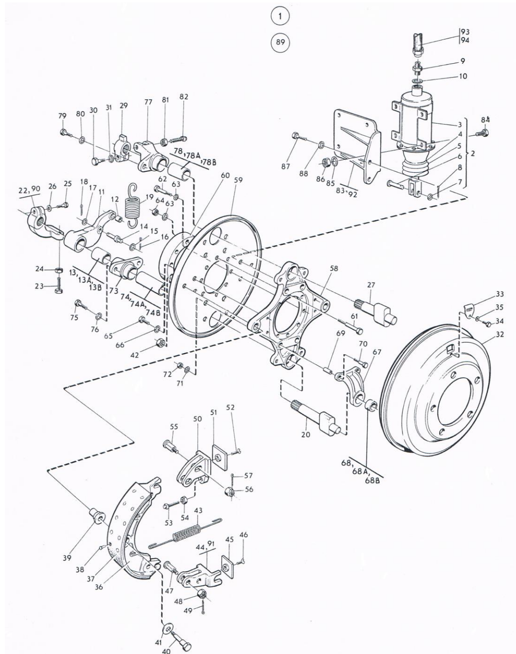
ภาพที่ 21 เบรกด้านหน้าซ้ายครบชุด
