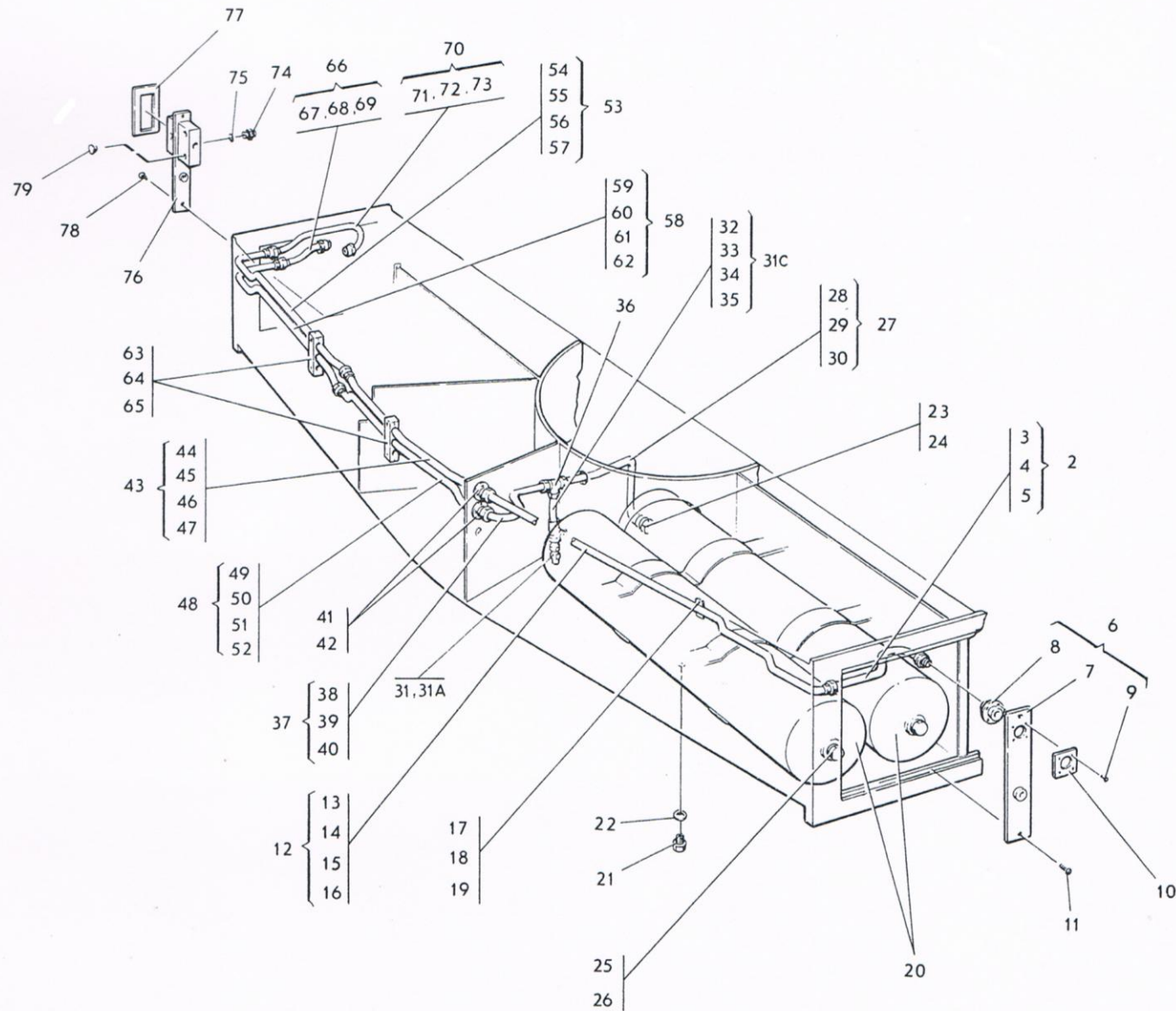
ภาพที่ 8 เบรกลมครบชุด
