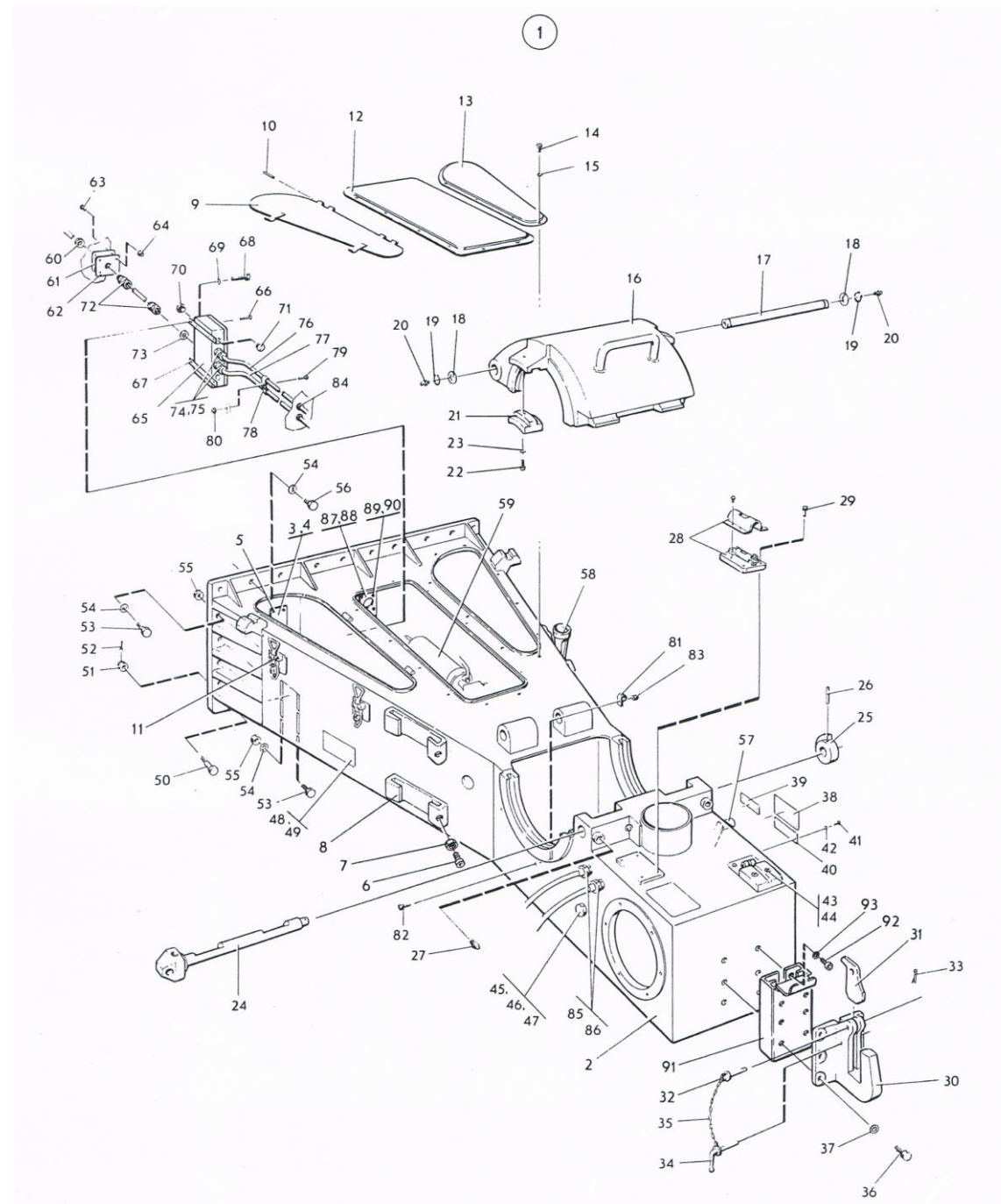
ภาพที่ 14 แทนปีนด้านหลังครบชุด
