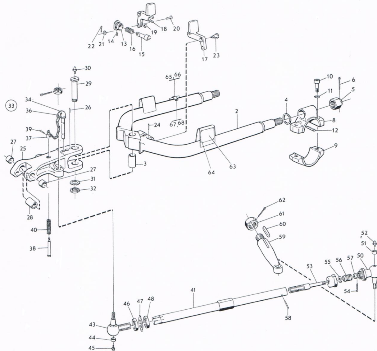
ภาพที่ 20 เฟืองบังคับเลี้ยวครบชุด
