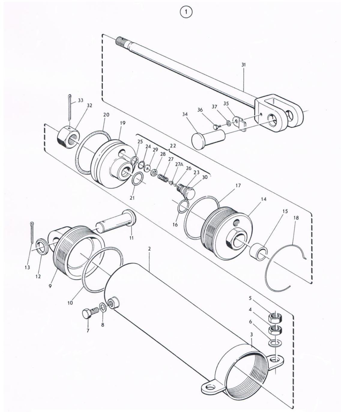
ภาพที่ 12 ชุดกระบอกไฮดรอลิค
