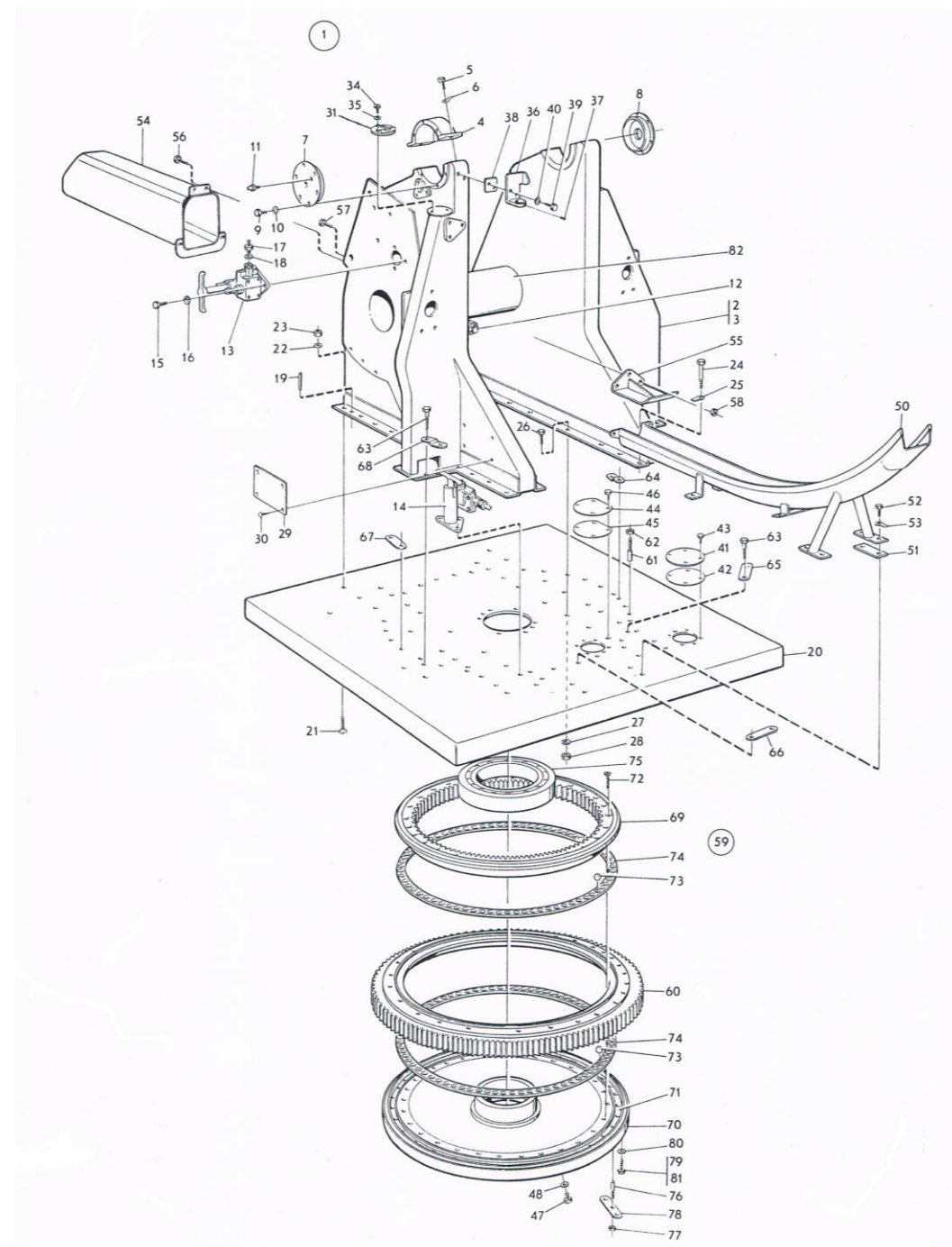
ภาพที่ 1 ชุดเรือนติดตั้ง
