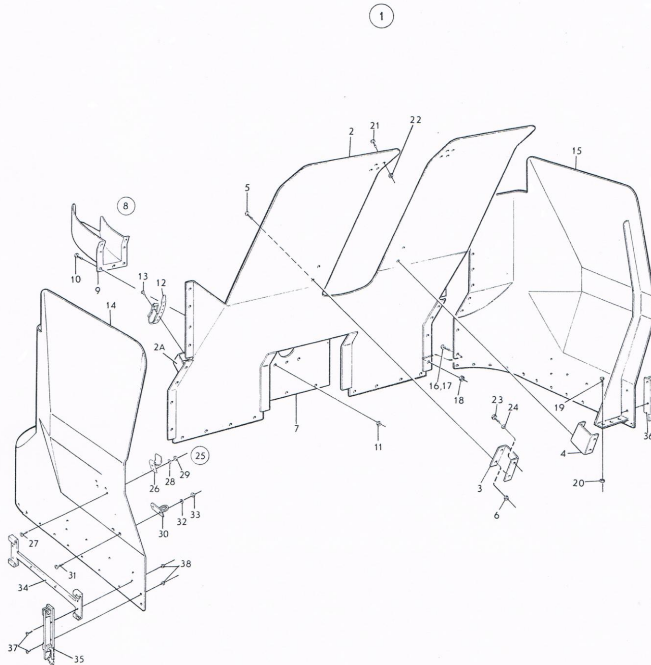
ภาพที่ 5 โถ่ปั่นครบชุด
