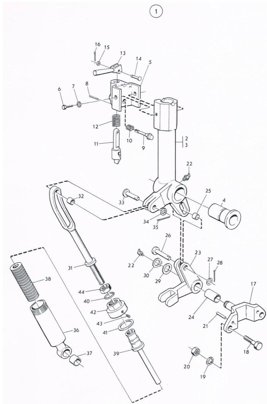
ภาพที่ 26 ชุดเบรกมือ
