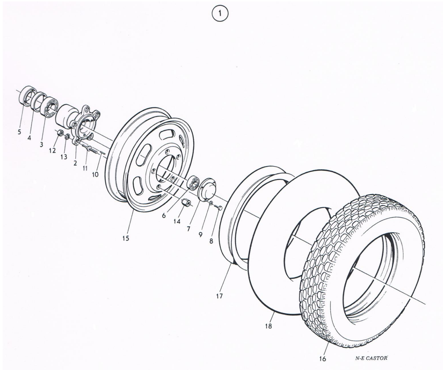
ภาพที่ 22 ล้อและกะทะล้อ
