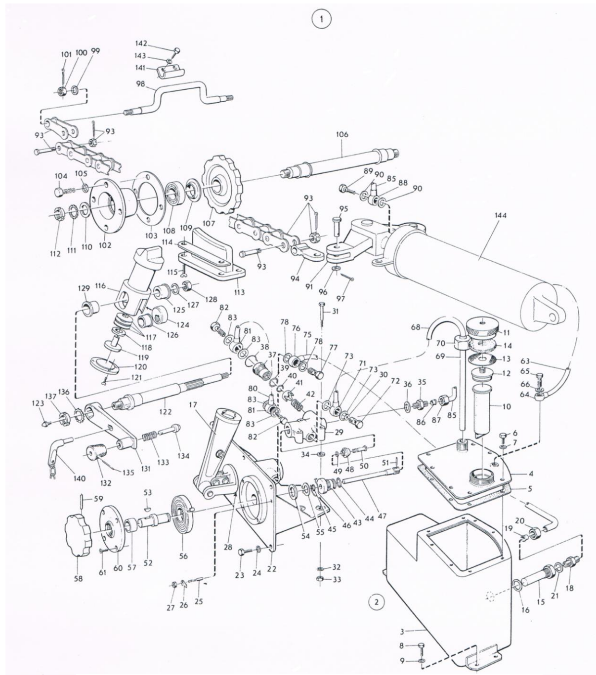
ภาพที่ 10 ชุดเฟืองยกเพลาด้านหน้า
