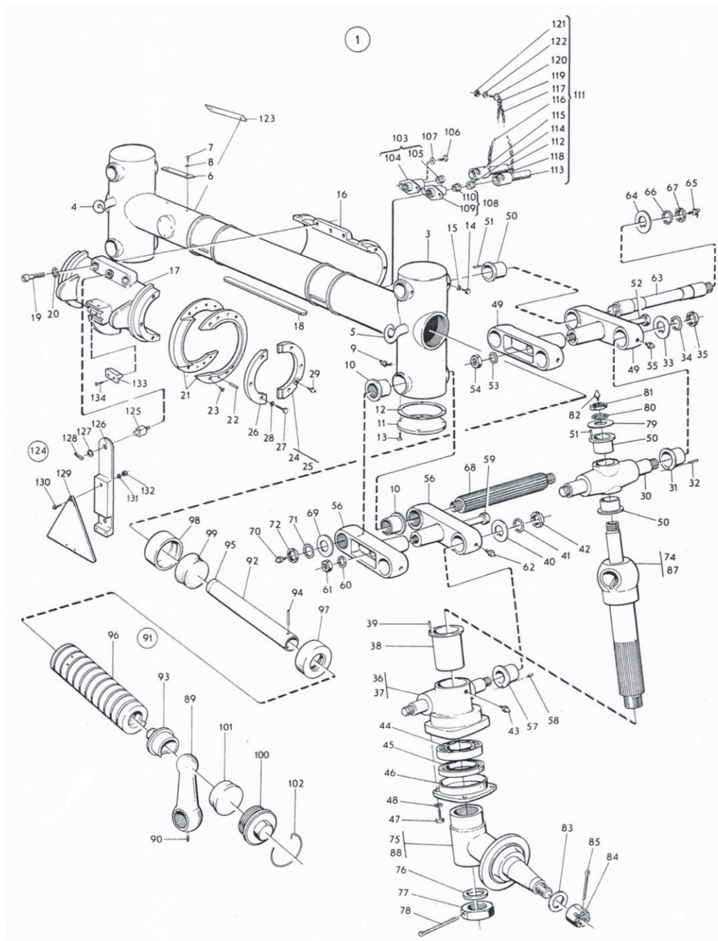
ภาพที่ 19 ฐานปืนด้านหน้าครบชุด
