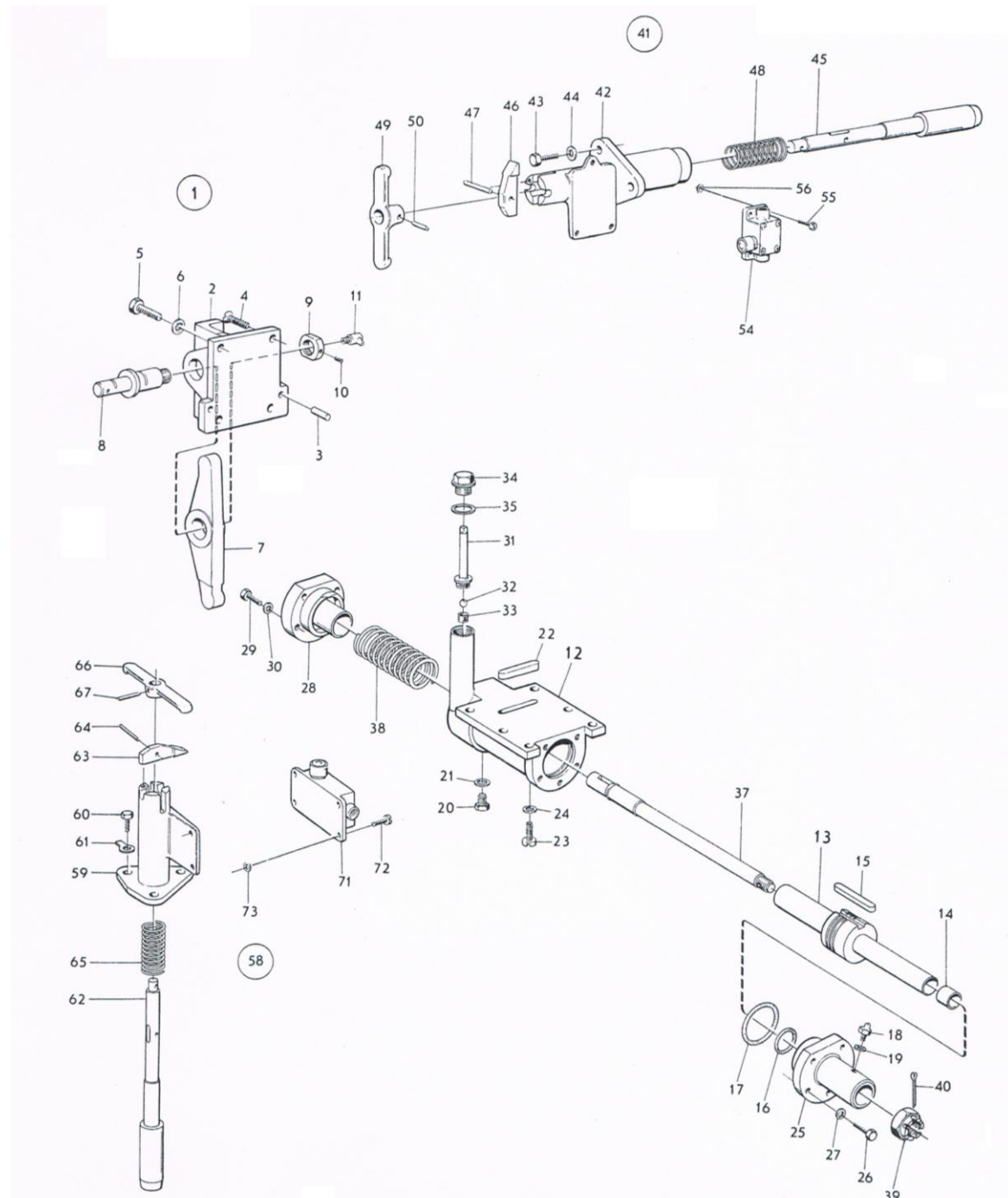
ภาพที่ 2 ชุดจำกัดมุมทางสูงครบชุด
