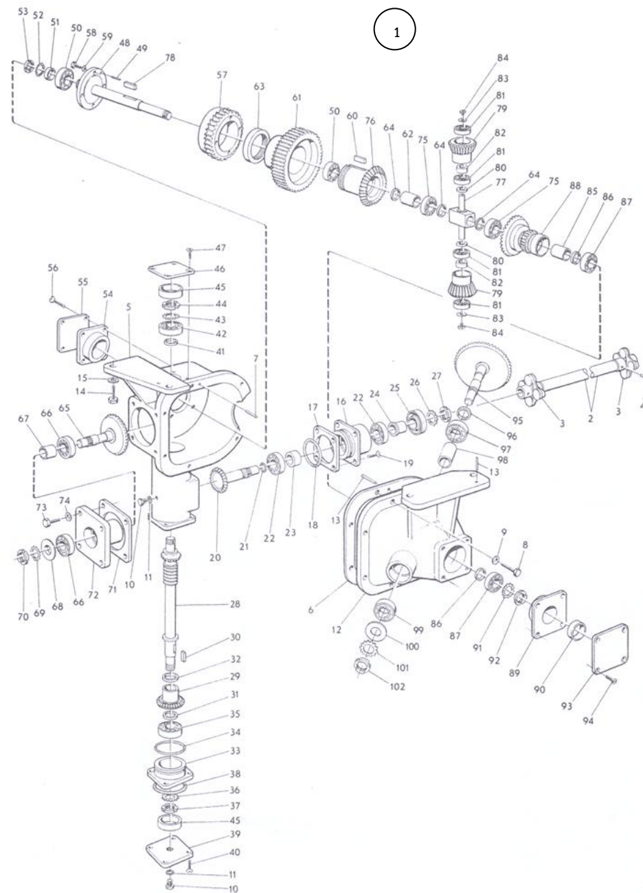
ภาพที่ 73 ชุดตั้งค่าเฟืองทดทางสูง
