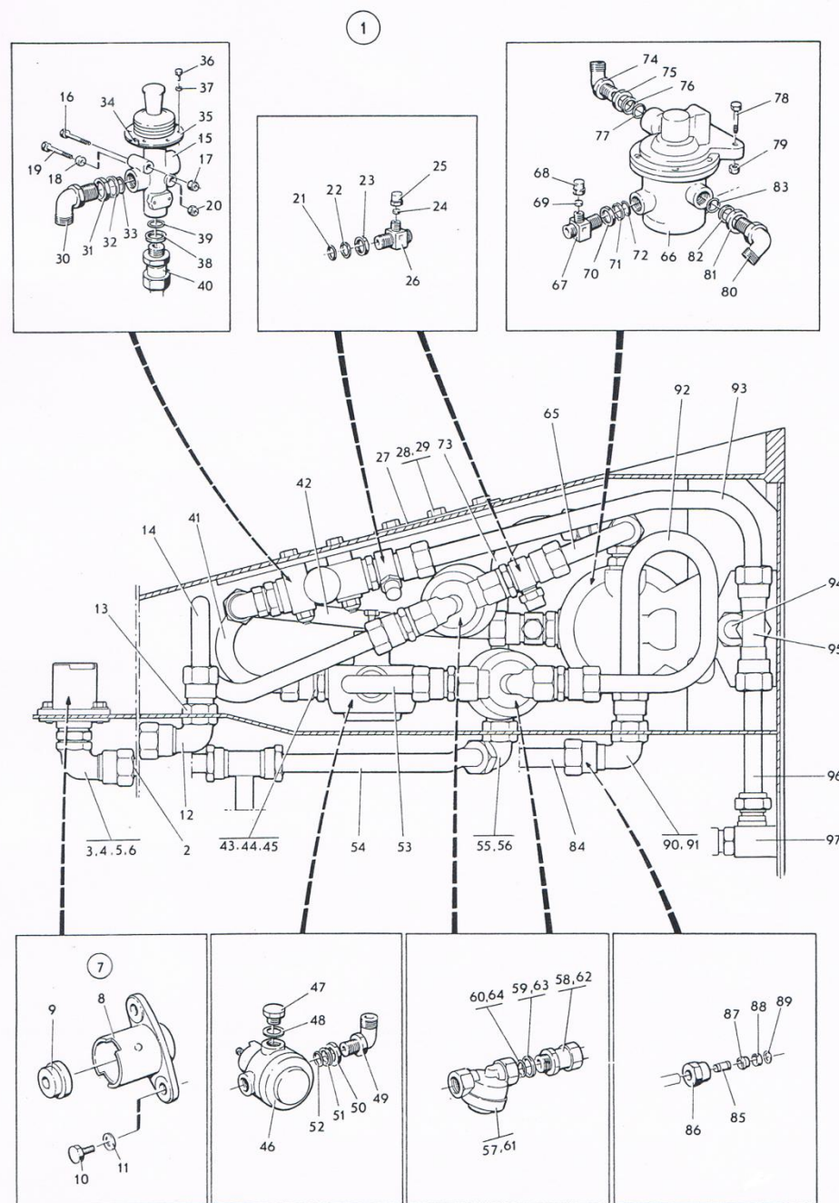
ภาพที่ 31 เบรกลมครบชุด
