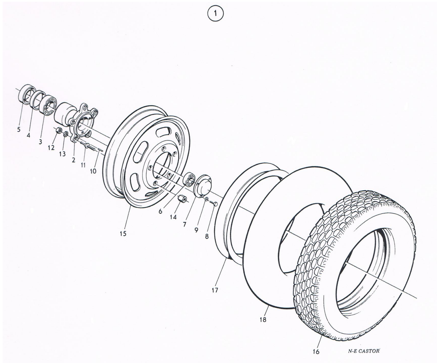
ภาพที่ 40 ล้อและกะทะล้อ
