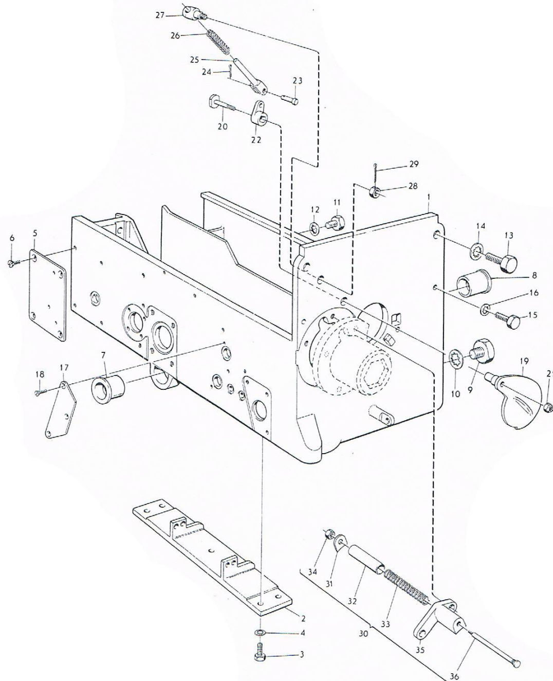
ภาพที่ 6 เครื่องป้อนกระสุนอัตโนมัติครบชุด
