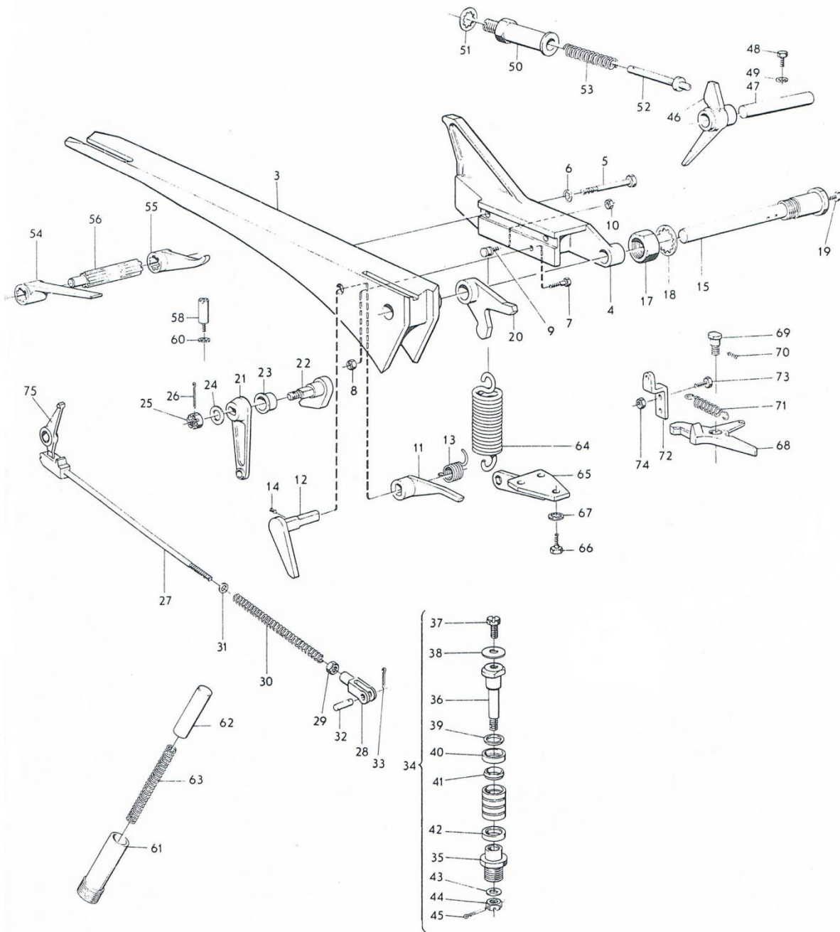
ภาพที่ 9 ถาดป้อนกระสุนครบชุด
