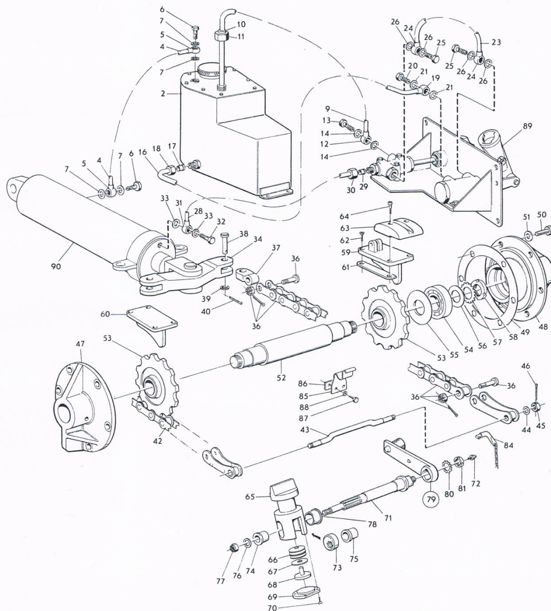
ภาพที่ 33 เฟืองยกเพลาลัง
