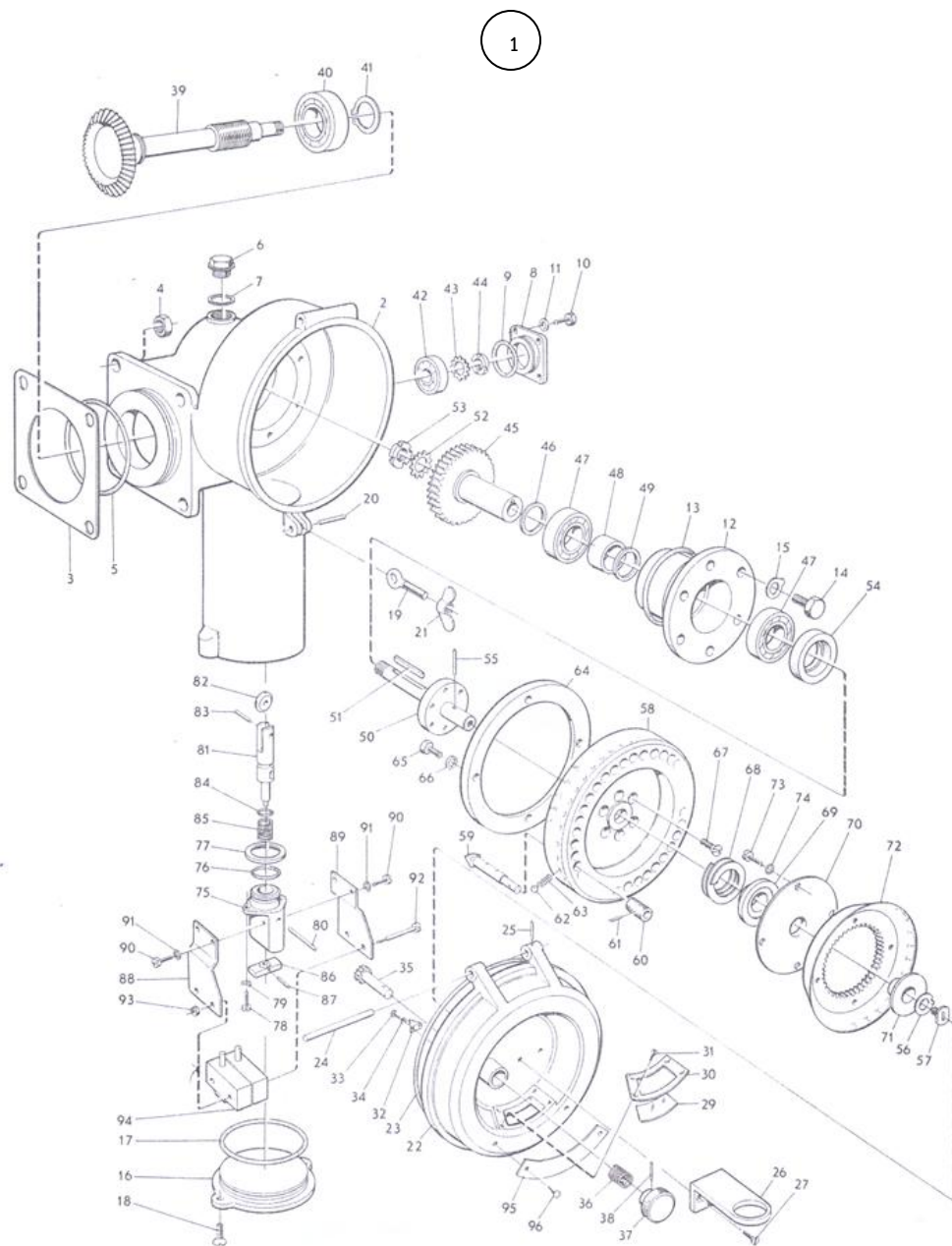
ภาพที่ 77 เครื่องตั้งเขตจำกัดการยิงทางทิศ
