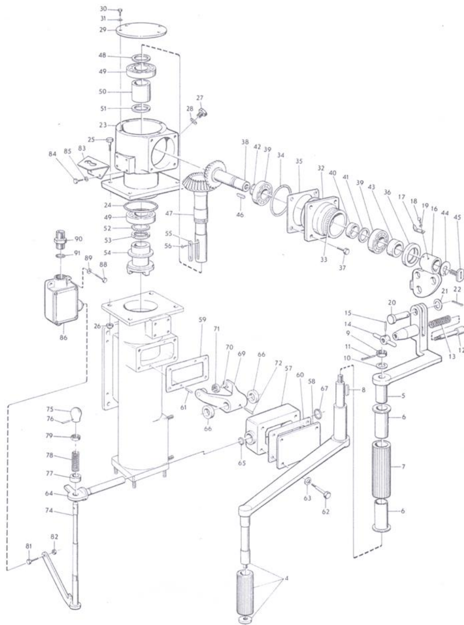
ภาพที่ 65 เฟืองให้มุมทางทิศรอบชุด
