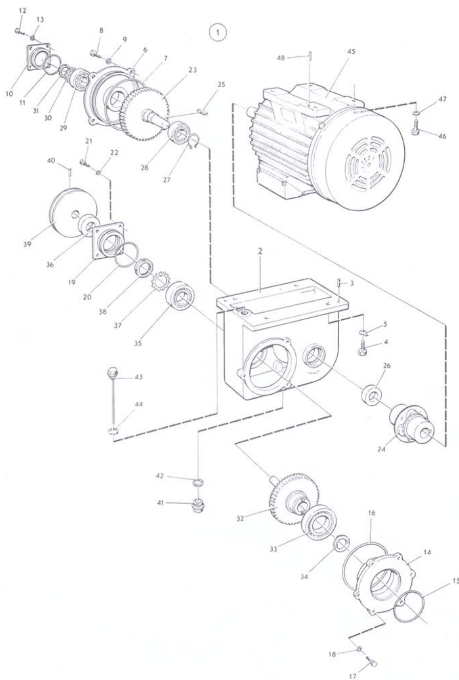
ภาพที่ 56 ป้อนเกียร์และมอเตอร์
