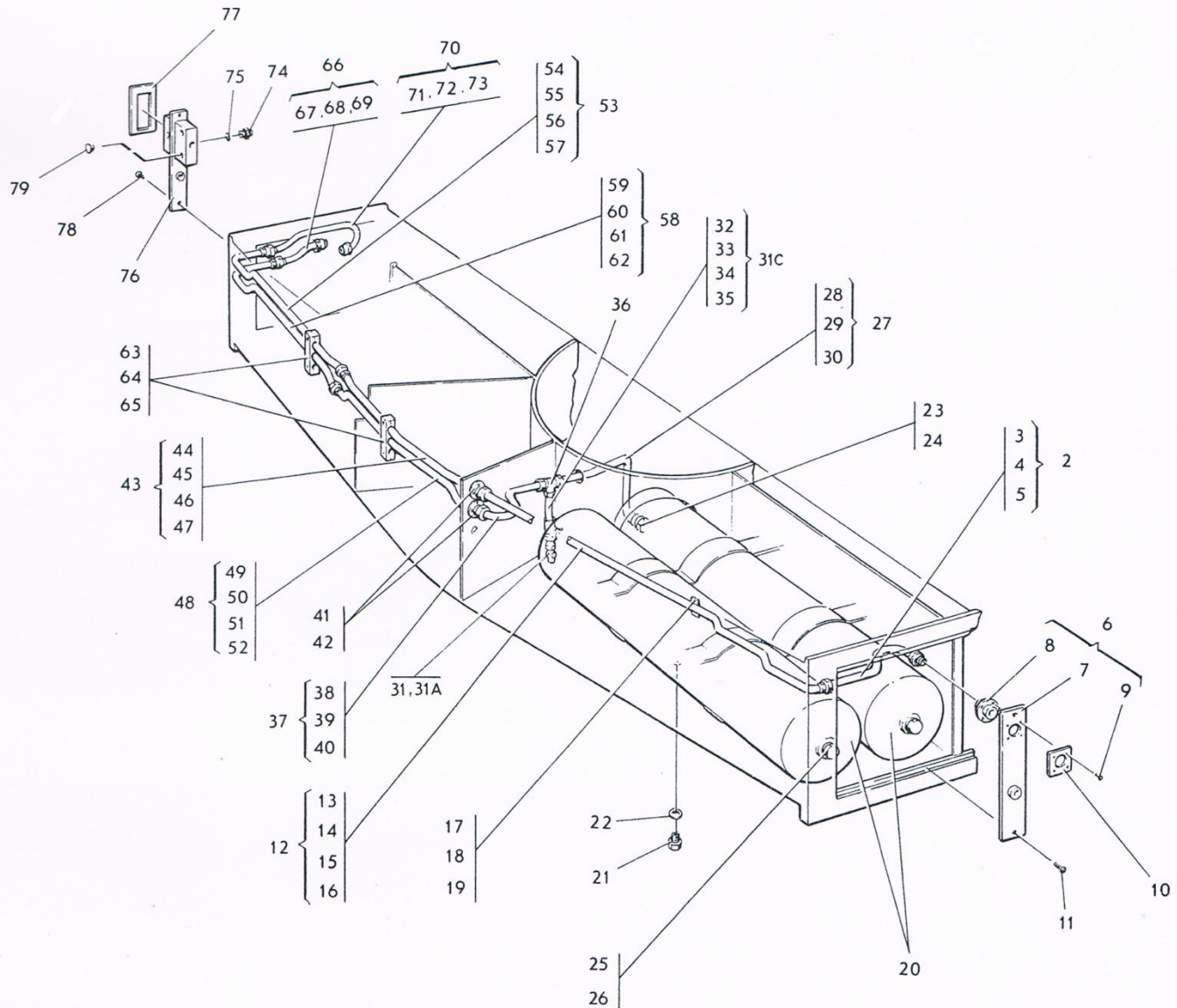
ภาพที่ 26 เบรกลมครบชุด
