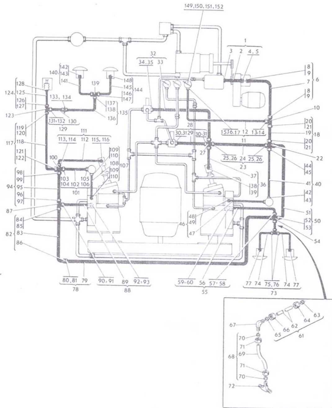
ภาพที่ 61 ท่อไฮดรอลิคครบชุด
