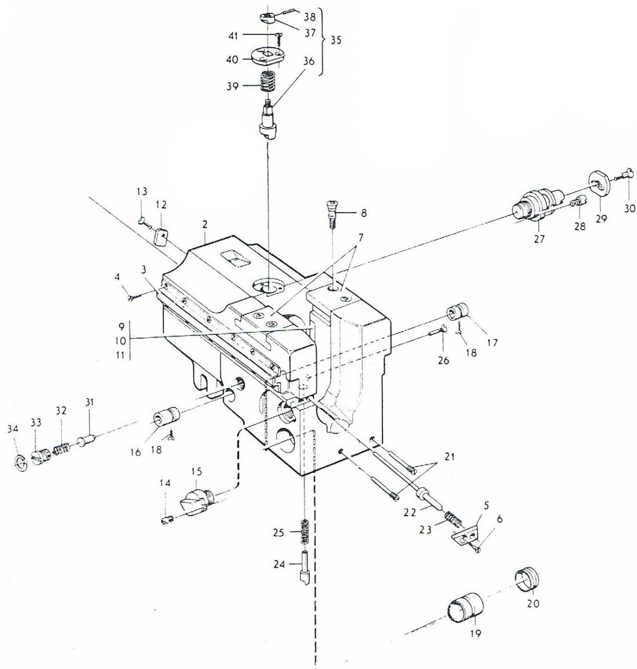
ภาพที่ 3 เรือนเครื่องปิดท้ายครบชุด
