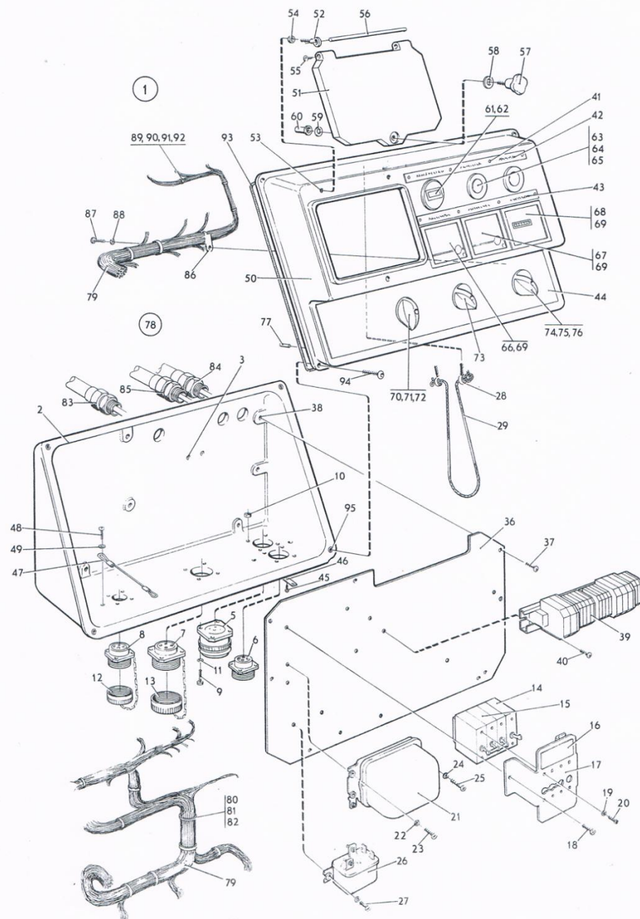
ภาพที่ 83 แผงควบคุมครบชุด, แผงเครื่องควบคุมครบชุด
