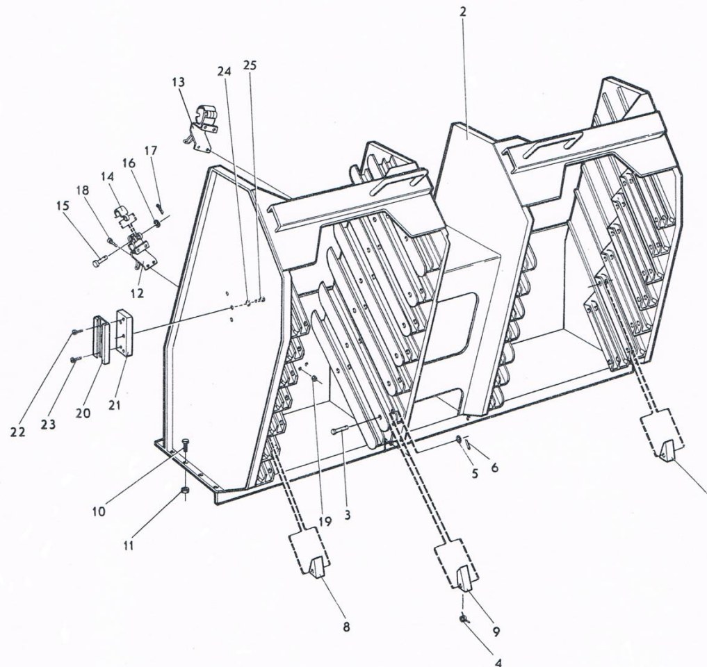
ภาพที่ 22 ร่างเก็บกระสุนครบชุด
