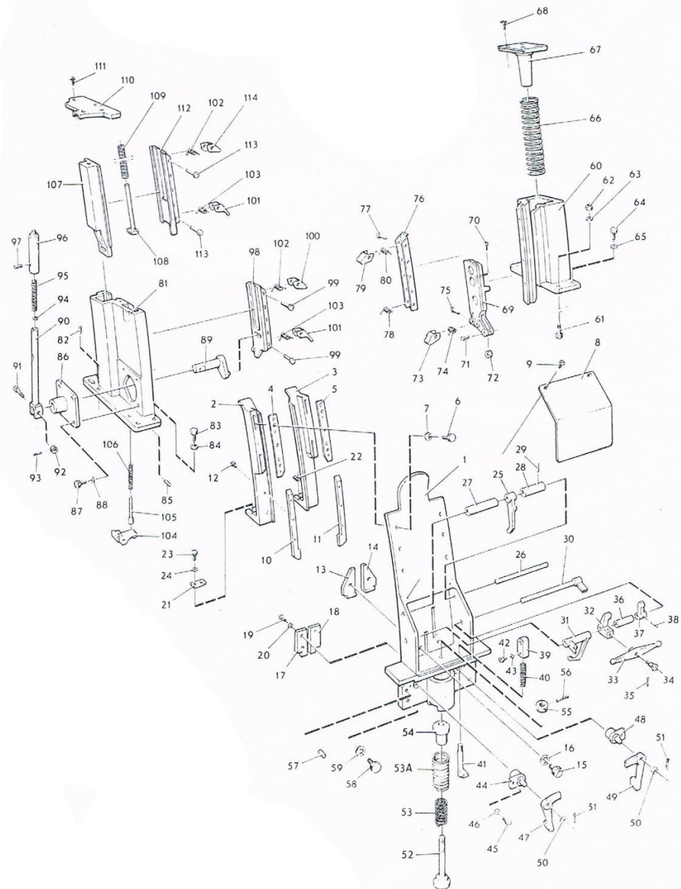
ภาพที่ 12 แผ่นนำกระสุนครบชุด
