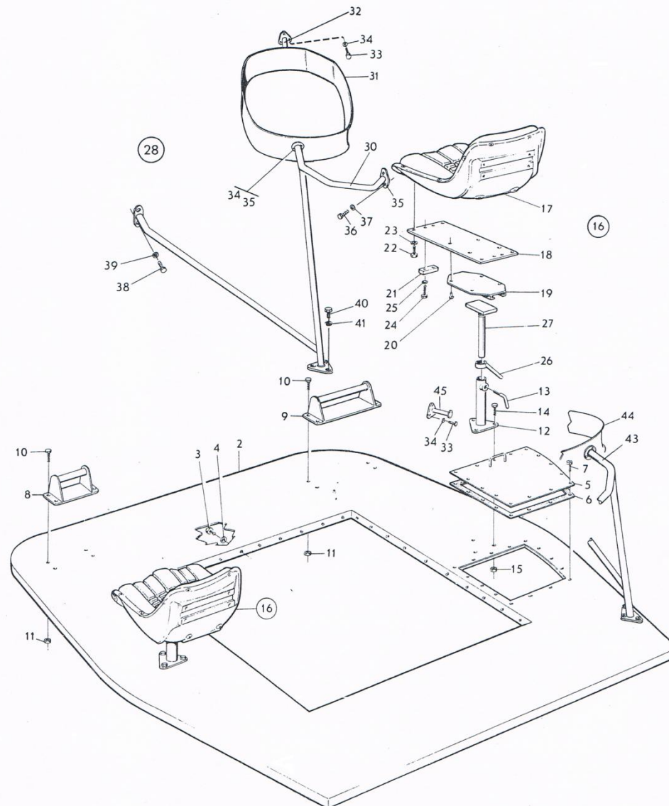
ภาพที่ 21 ฐานปีนครบชุด
