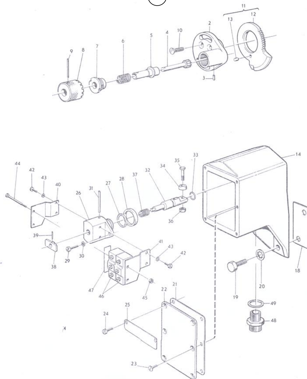
ภาพที่ 78 เครื่องตั้งเขตจำกัดการยิงทางสูง
