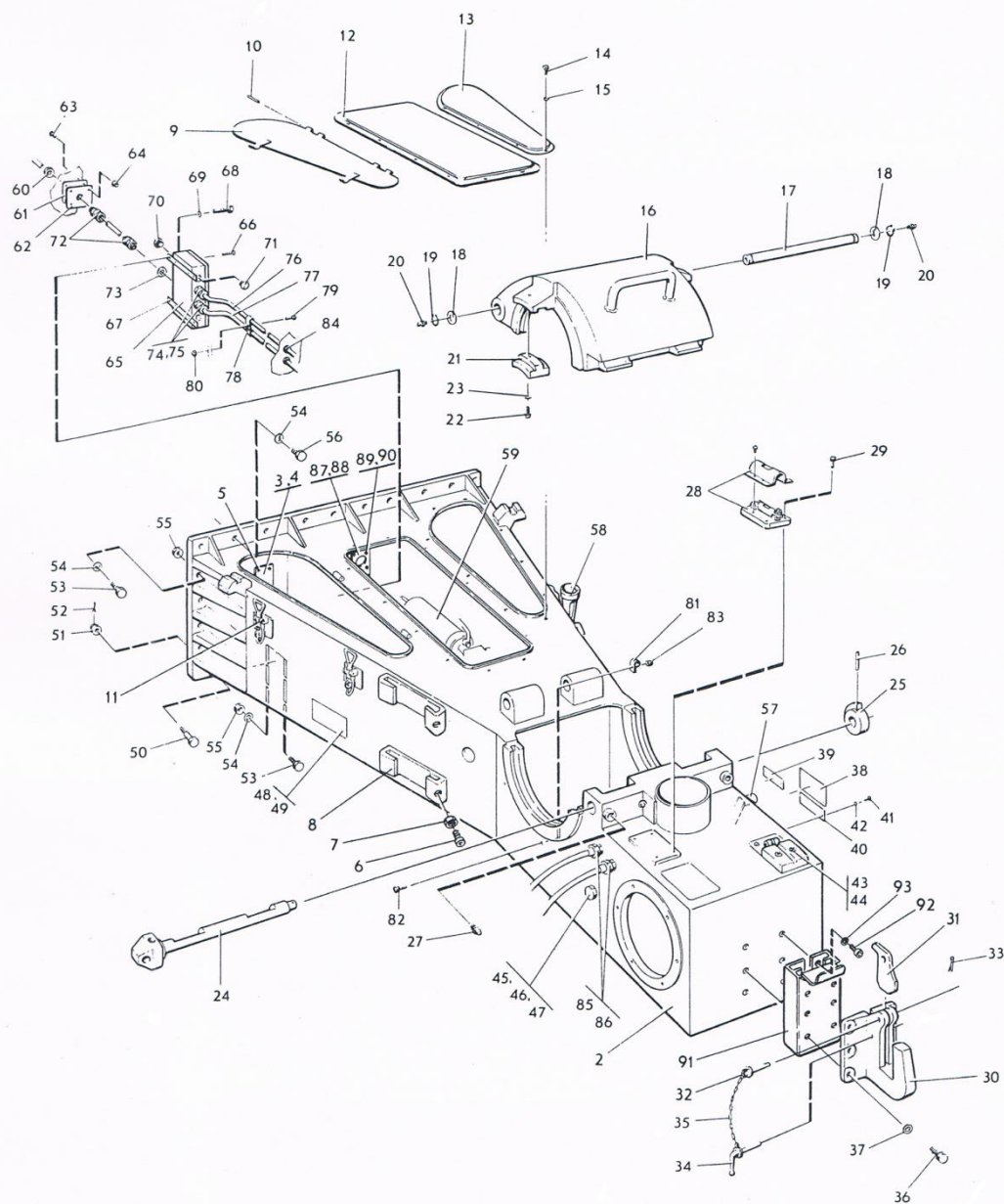
ภาพที่ 32 แท่นป็นด้านหลังกบชุด
