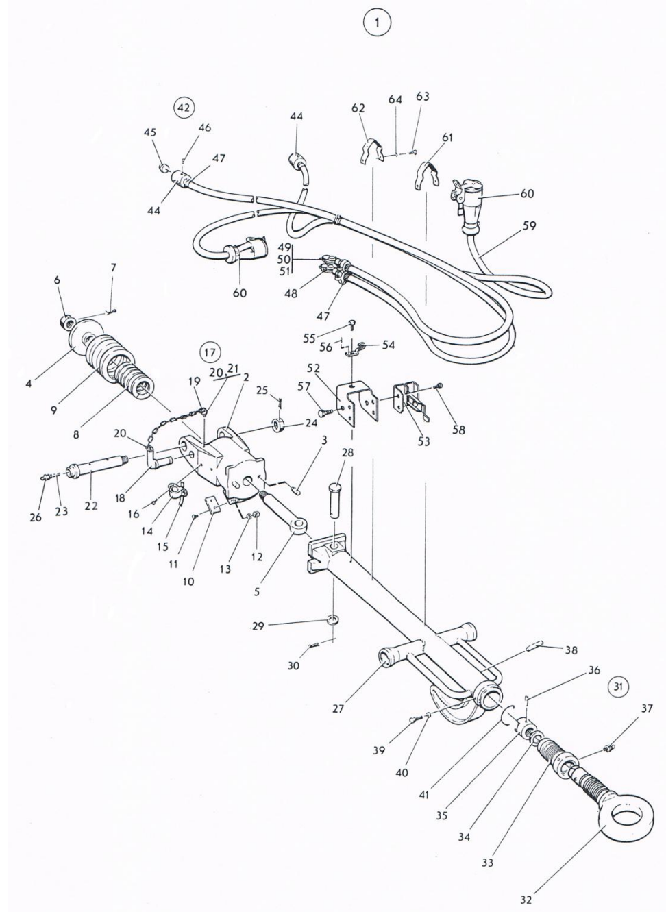
ภาพที่ 41 ห่วงลากจูงครบชุด
