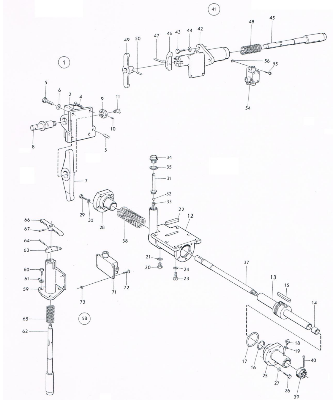
ภาพที่ 20 ชุดจํักัดมุมทางสูง
