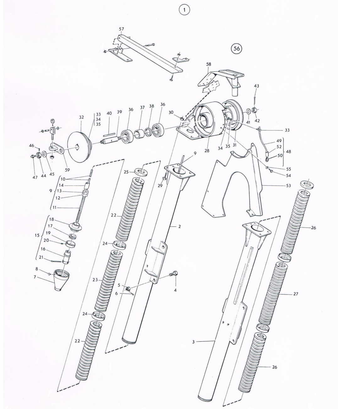
ภาพที่ 24 เครื่องช่วยทางสูงครบชุด
