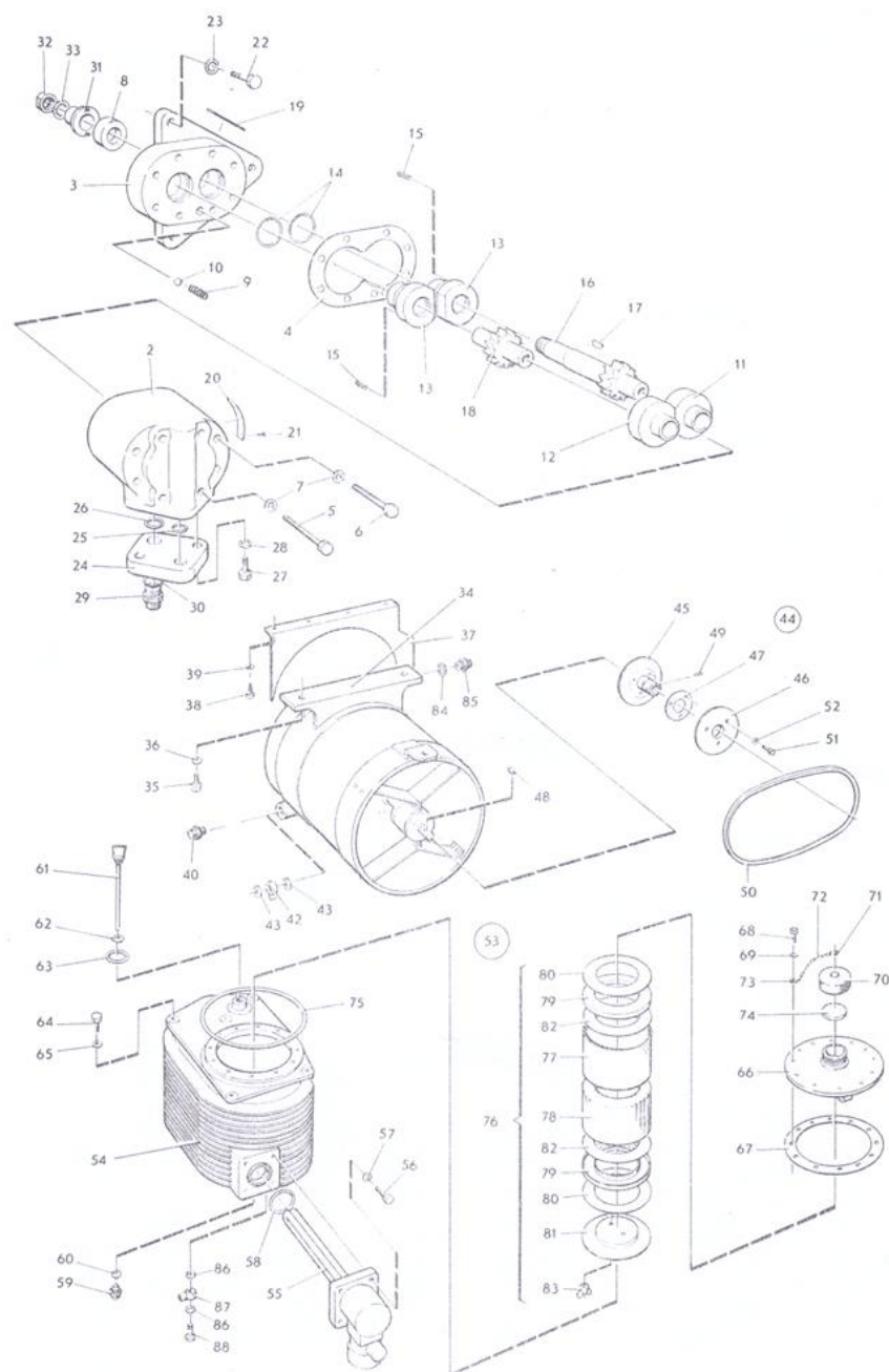
ภาพที่ 60 ป้อนน้ำมัน เครื่องระบายความร้อนและถังน้ำมันเครื่อง, พู่เล่ย์, ถังน้ำมันเครื่องพร้อมไส้กรอง
