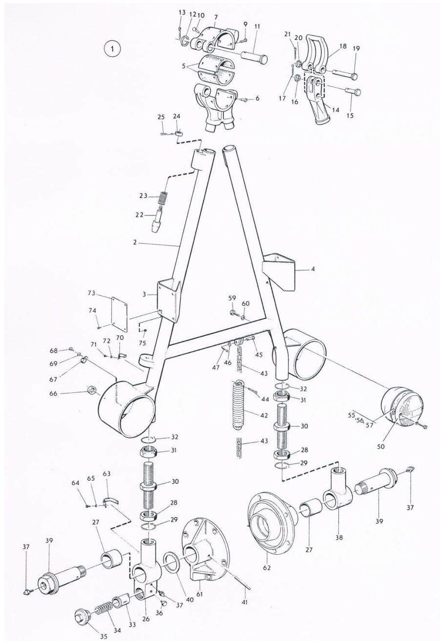
ภาพที่ 34 แขนยึดปีนครบชุด
