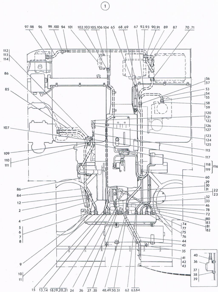
ภาพที่ 50 ส่วนติดตั้งระบบไฟฟ้า
