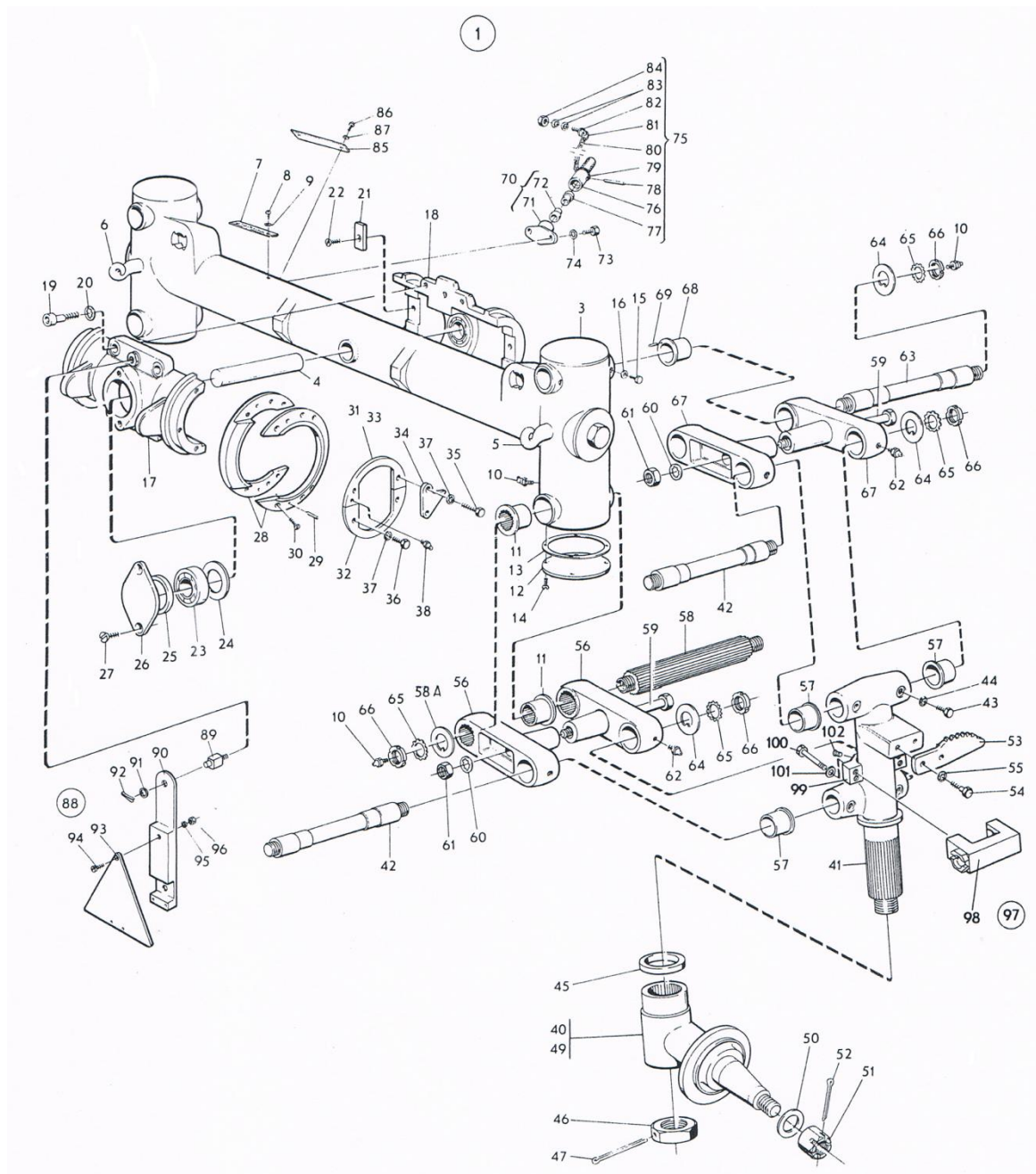
ภาพที่ 42 แกนเพลาลังครบชุด
