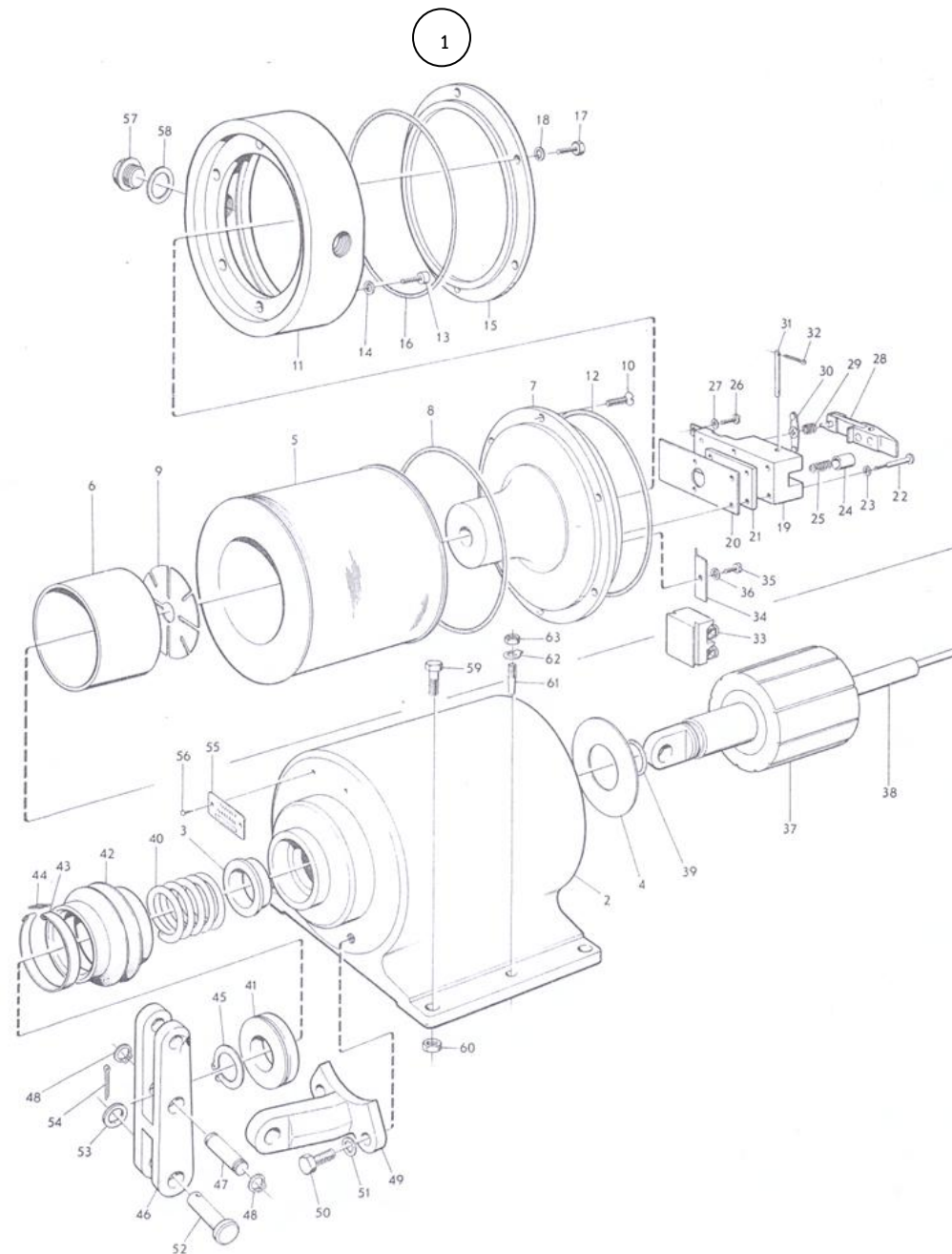
ภาพที่ 76 เครื่องลั่นไกด้วยแม่เหล็กไฟฟ้า
