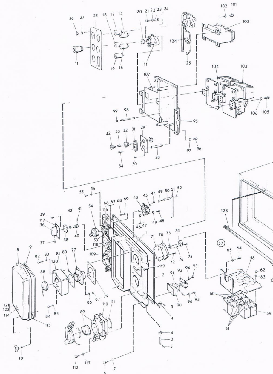
ภาพที่ 47 กล่องจ่ายไฟ, แทนยี่ห้อรีเลย์ครบชุด
