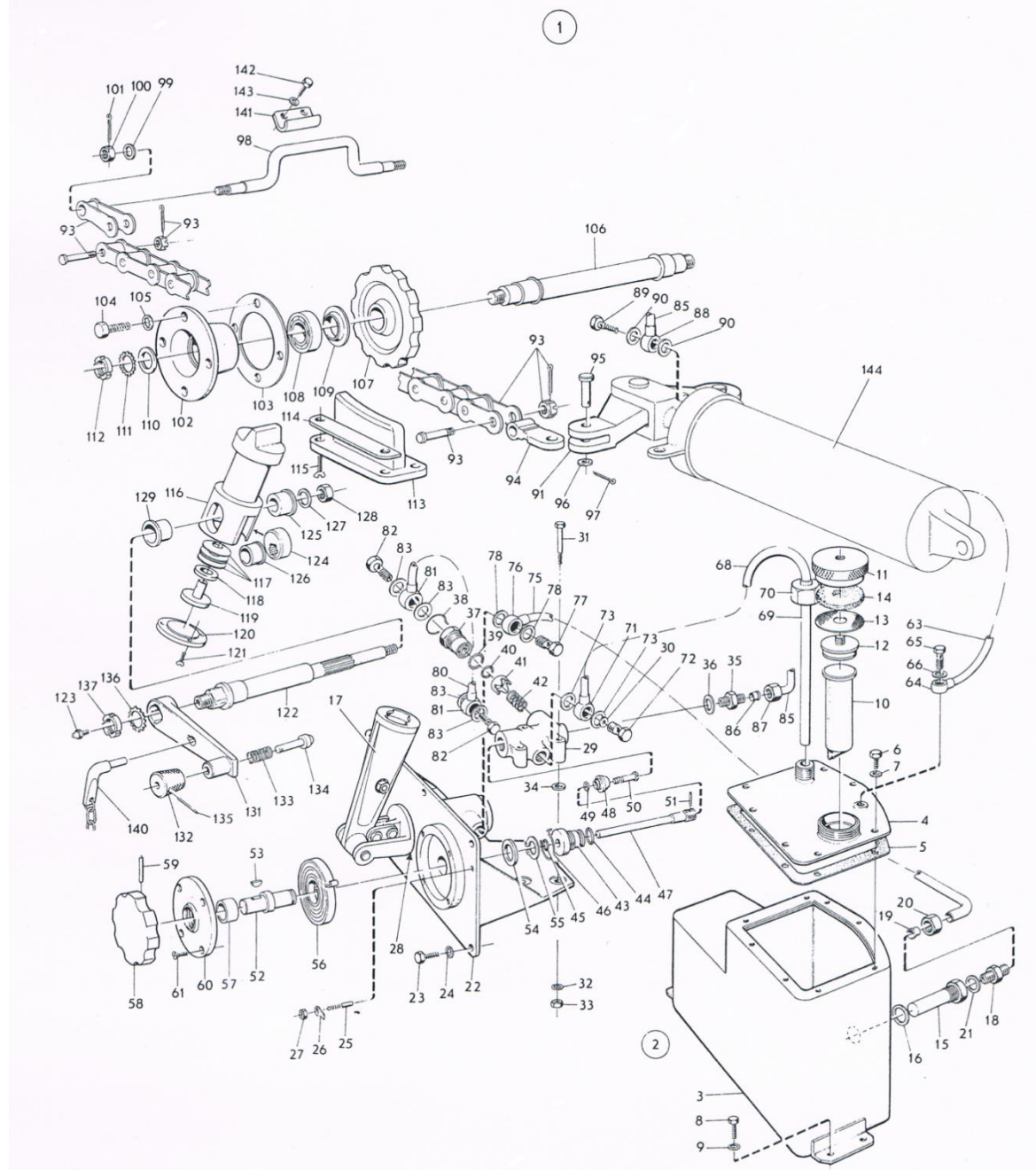
ภาพที่ 28 เฟืองยกเพลาด้านหน้าครบชุด
