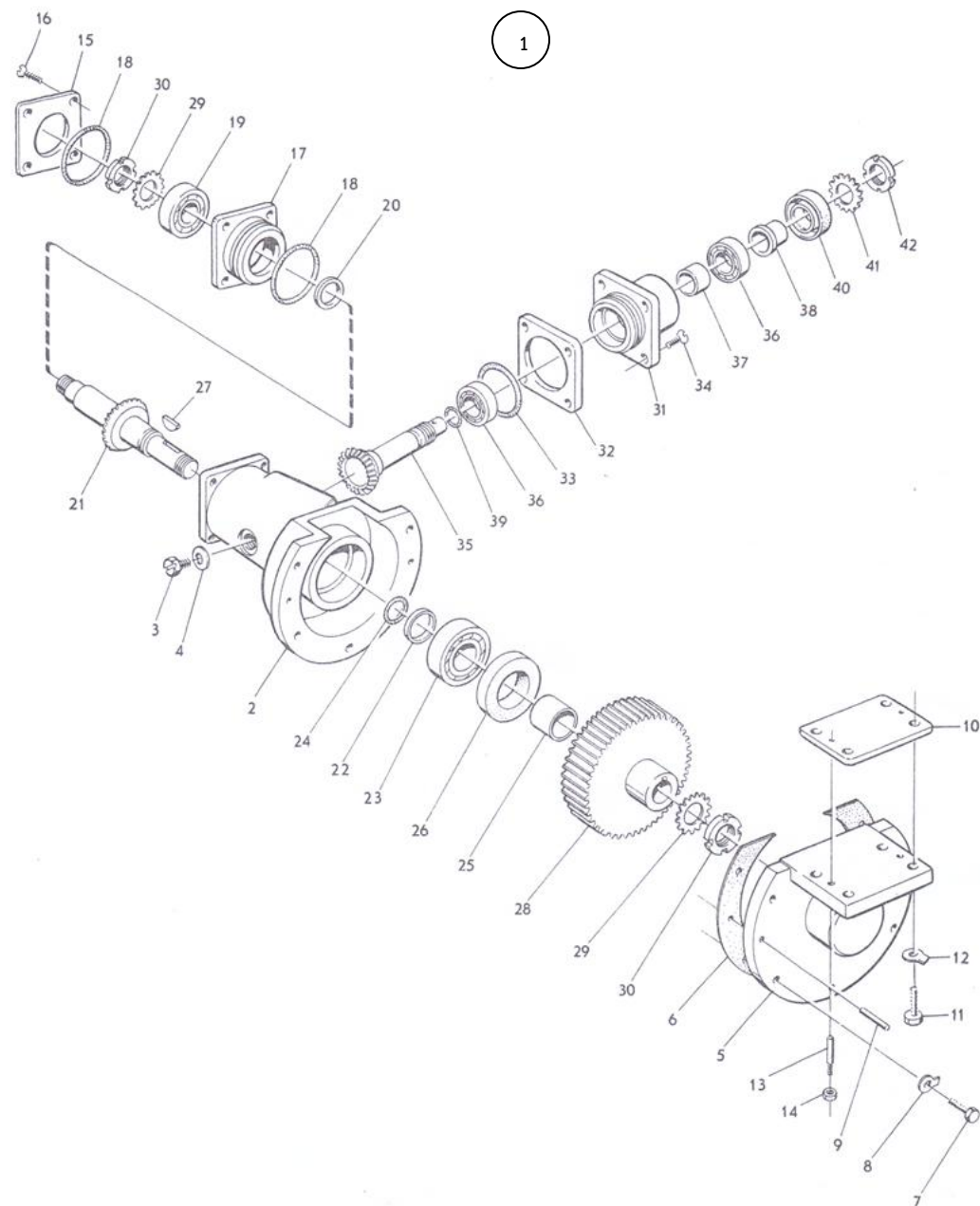
ภาพที่ 72 ชุดตั้งค่าเฟืองทดทางทิศ
