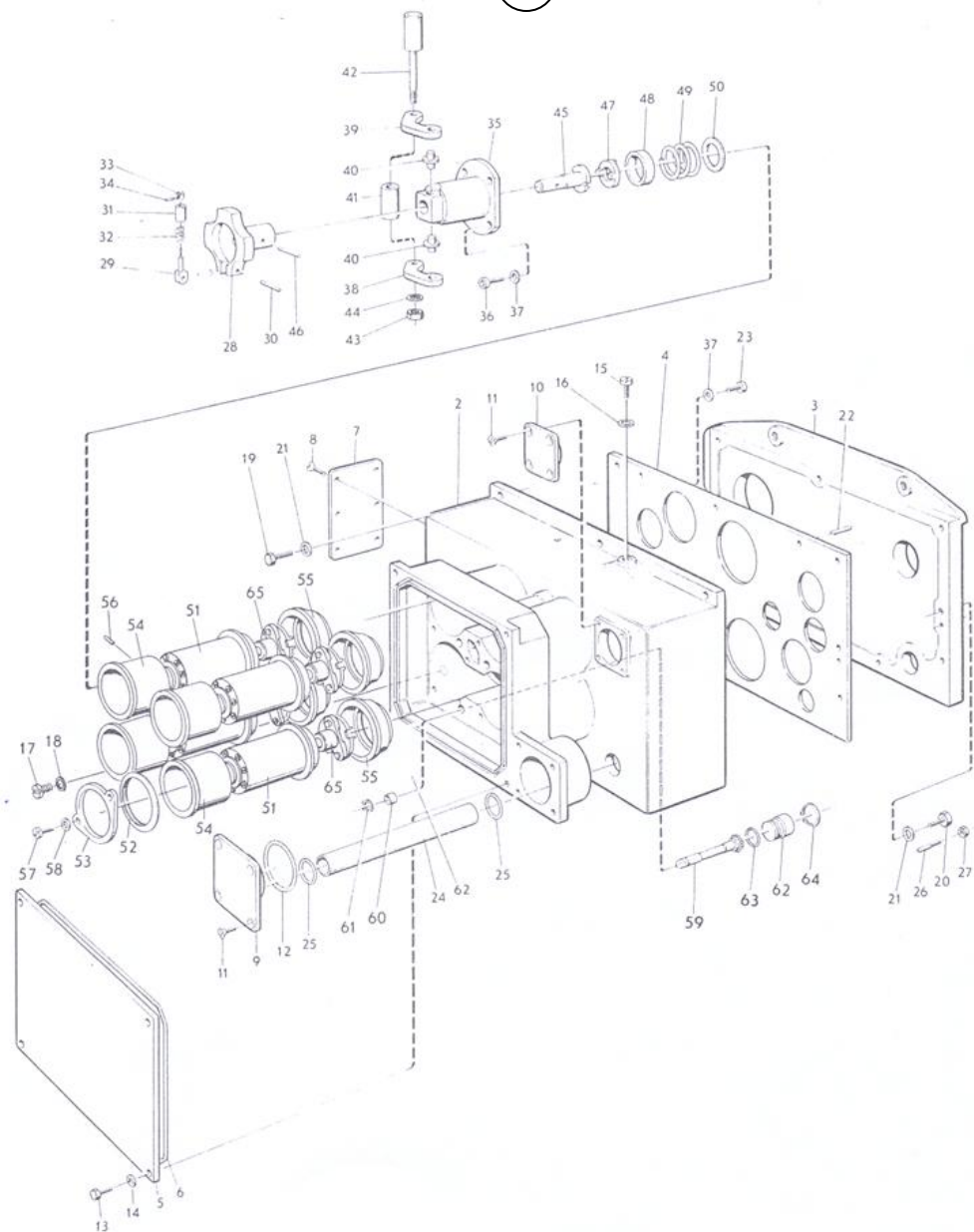
ภาพที่ 71 กล่องตั้งค่าครบชุด
