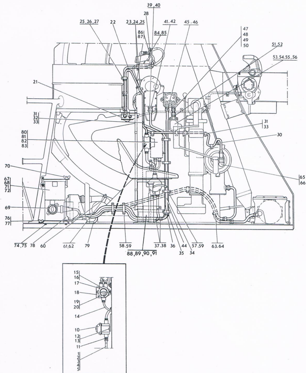
ภาพที่ 51 ส่วนติดตั้งระบบไฟฟ้า
