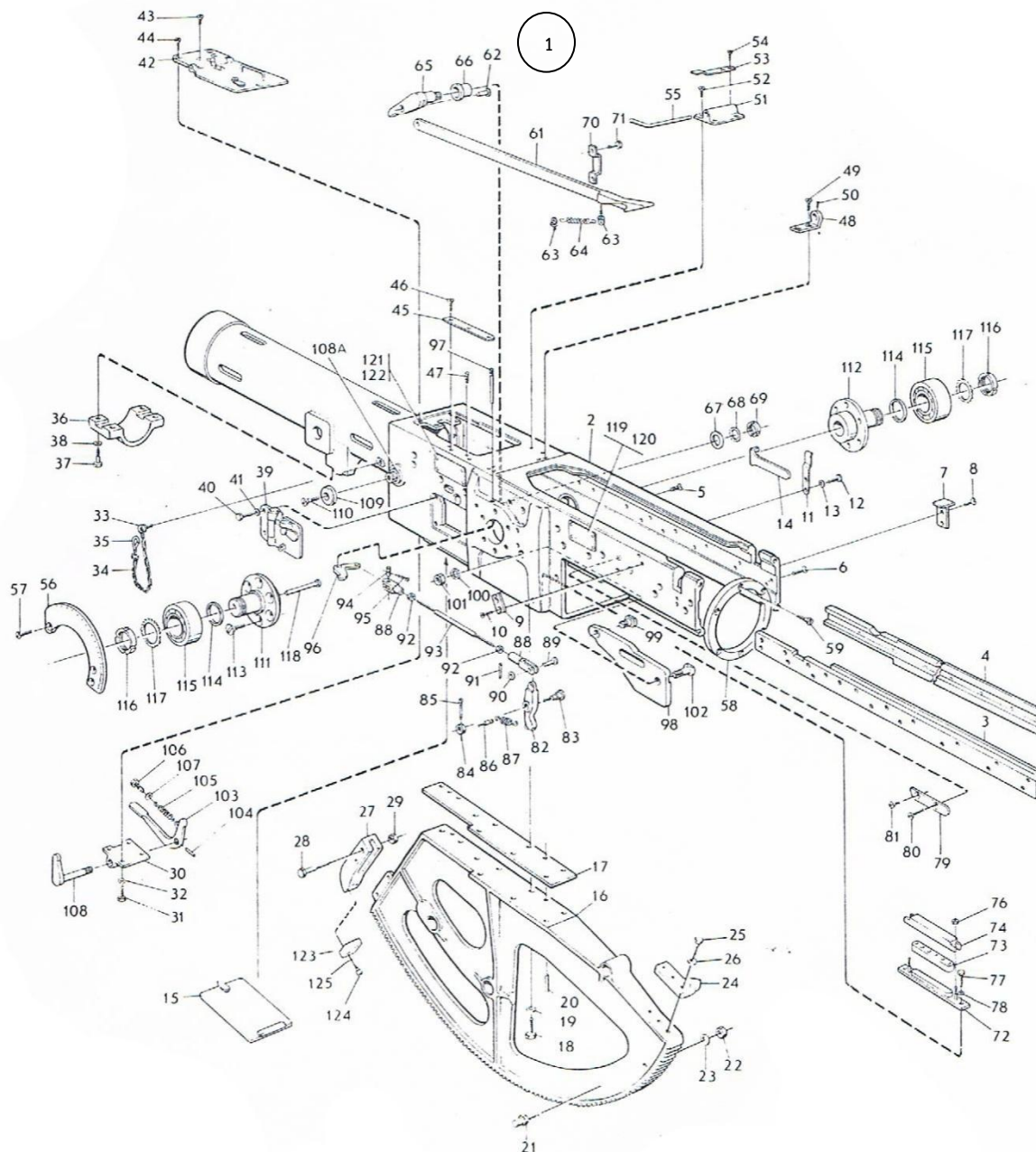
ภาพที่ 14 ชุดเรือนเครื่องปิดท้าย
