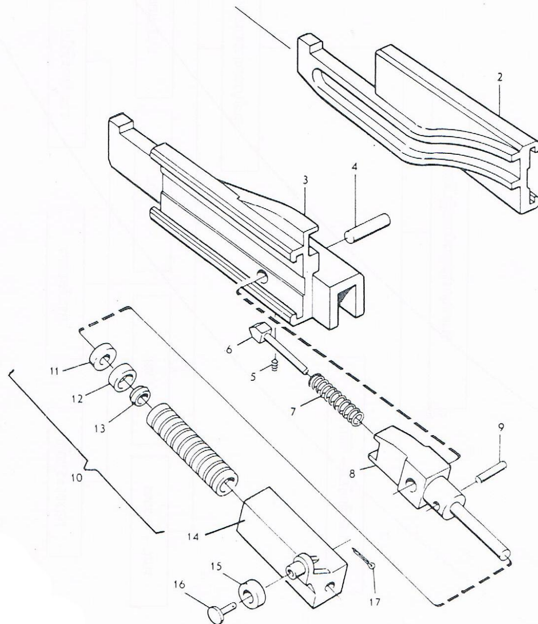
ภาพที่ 5 ลาดบังคับขึ้นนกรบชุด
