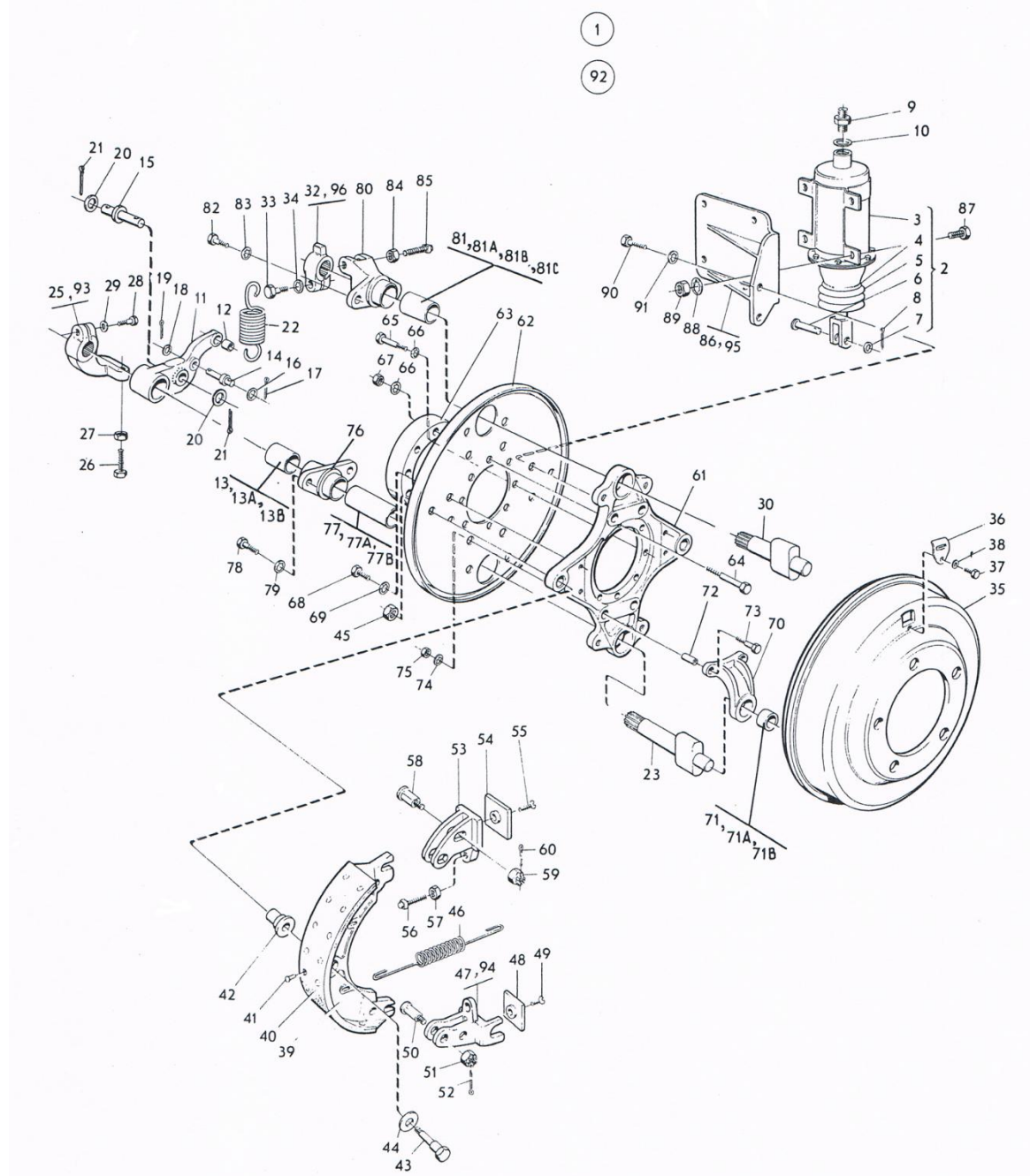
ภาพที่ 43 เบรกหลังด้านซ้ายครบชุด
