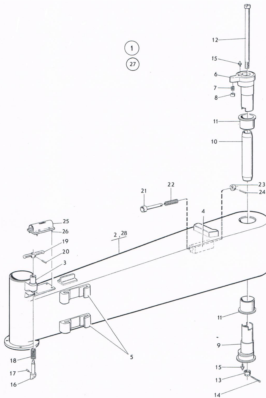
ภาพที่ 35 ชุดไทป์นภายนอกด้านซ้าย
