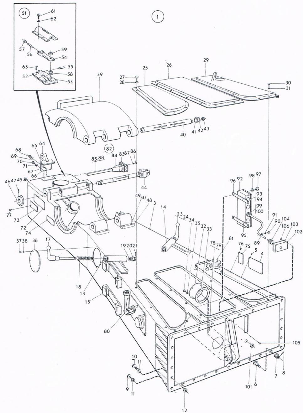
ภาพที่ 27 ฐานปีนด้านหน้าครบชุด
