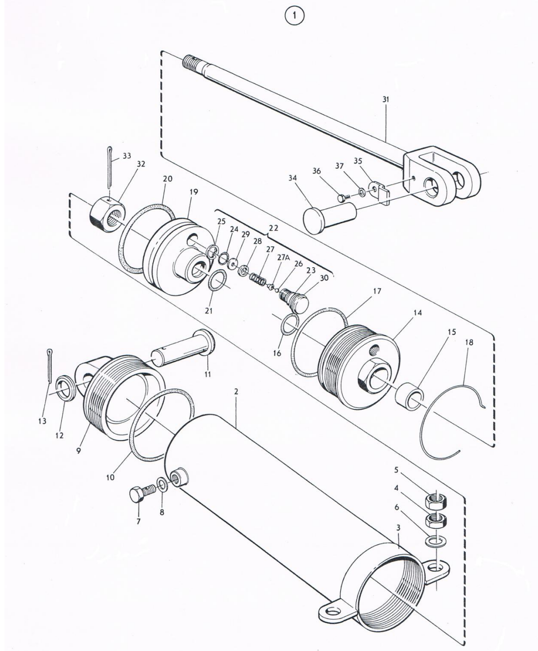
ภาพที่ 30 กระบอกไฮดรอลิค
