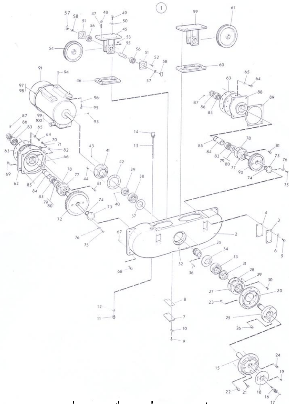
ภาพที่ 53 เครื่องเปลี่ยนความเร็ว
