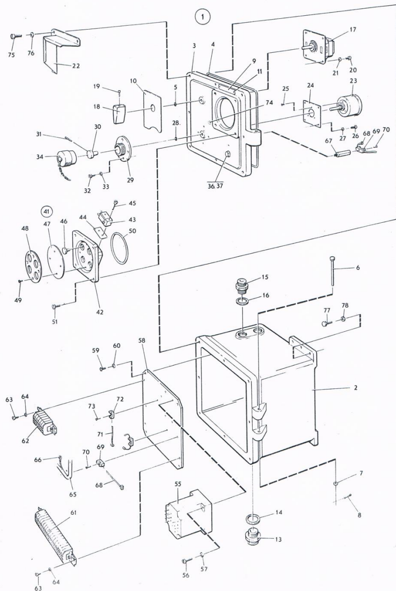
ภาพที่ 45 ชุดสตาร์ทและกล่องสวิตช์
