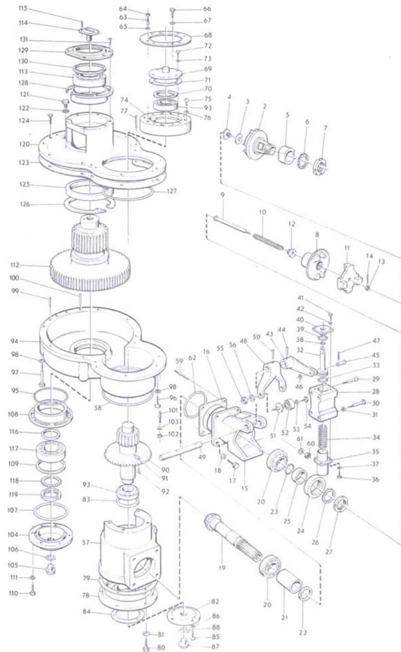
ภาพที่ 67 เฟืองให้มุมทางทิศ
