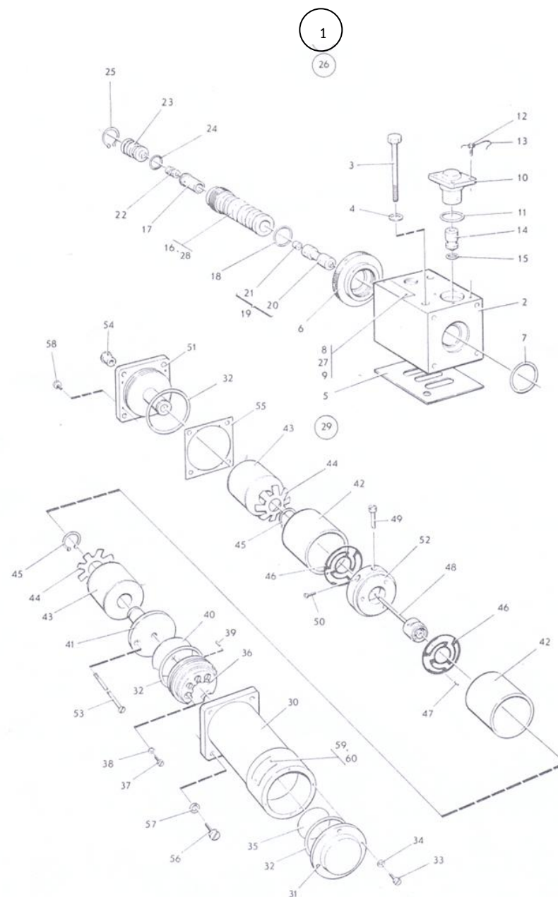
ภาพที่ 55 เครื่องเปลี่ยนความเร็วด้วยไฮดรอลิก, วาล์วนำทางสูงครบชุด, วาล์วนำทางทิศครบชุด
