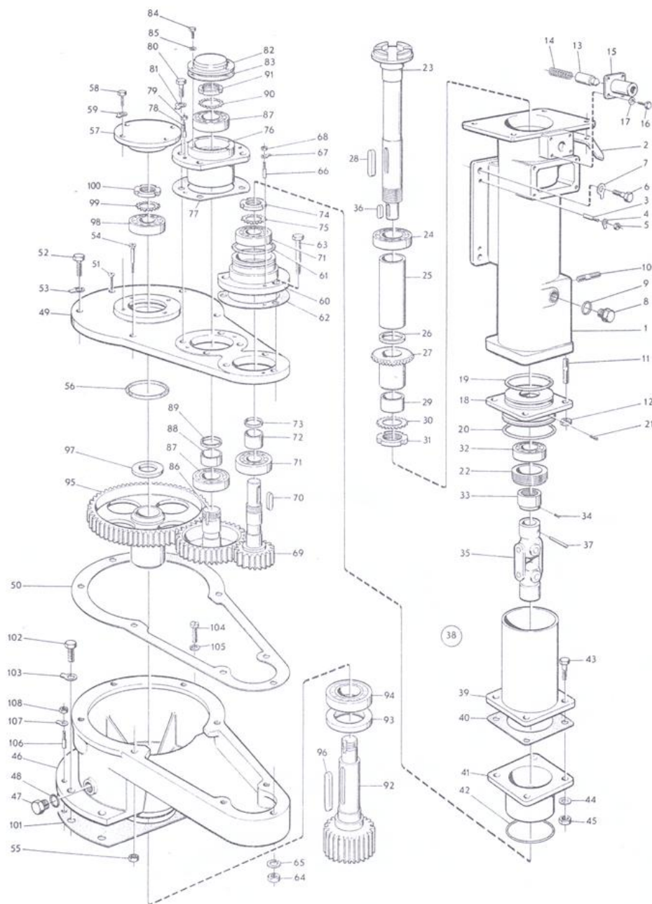
ภาพที่ 66 ควมมือหมุนให้มุมทางทิศครบชุด, ชุดเฟืองให้มุมทางทิศ ส่วนล่าง
