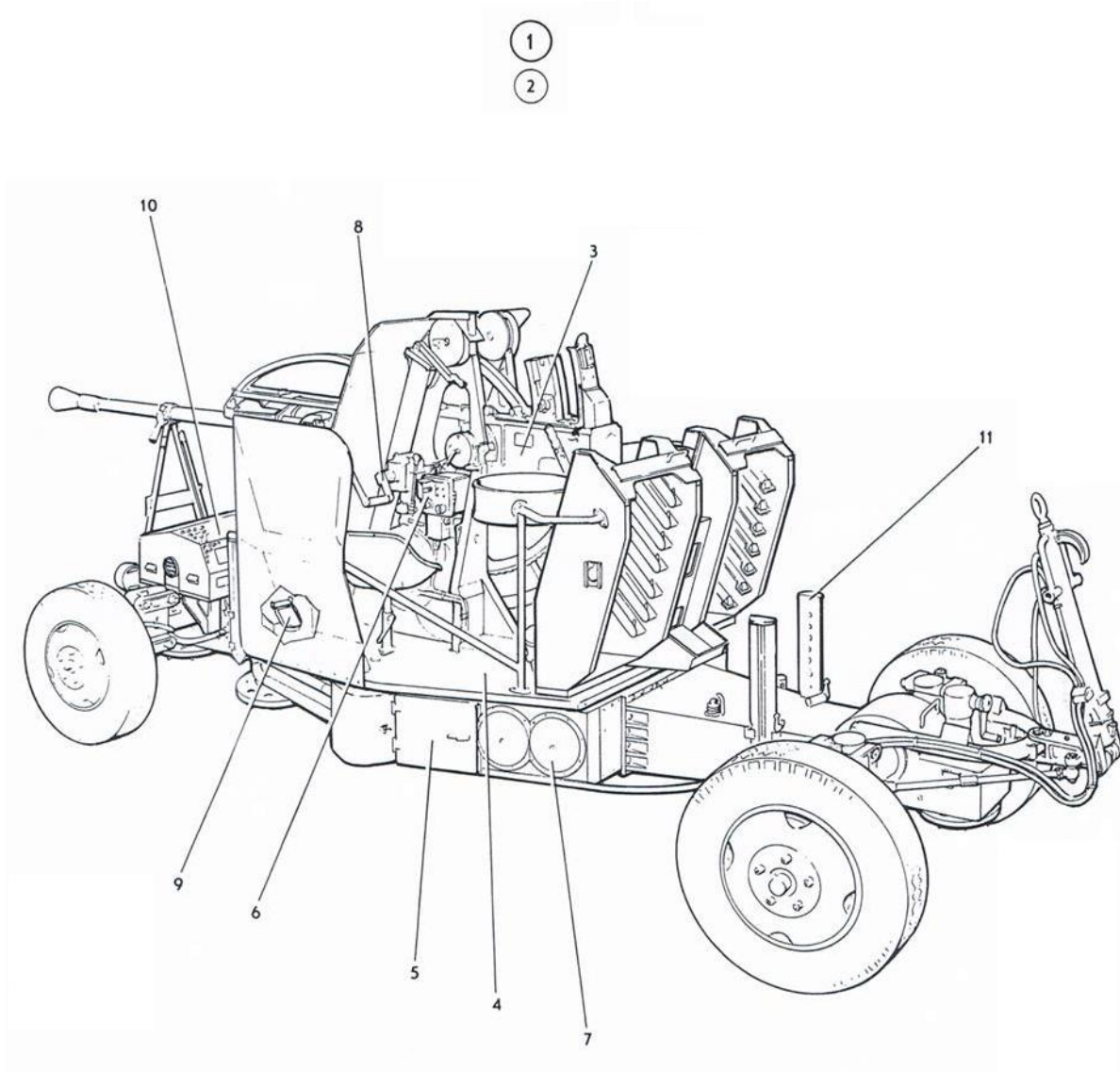
ภาพที่ 1 ส่วนตัวปีนครบชุด
