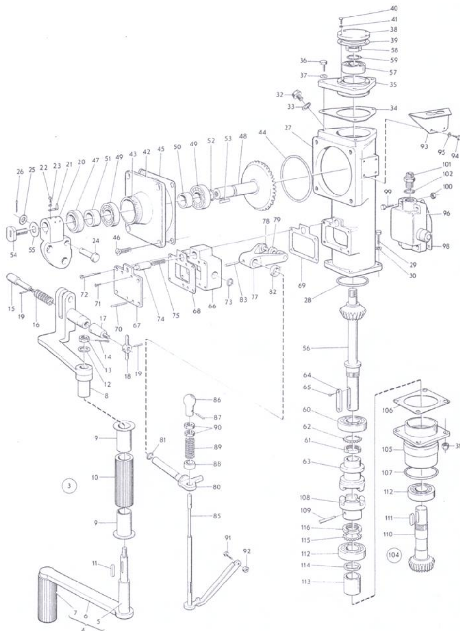
ภาพที่ 64 ชุดเฟืองให้มุมทางสูง, ชุดเฟืองให้มุมทางสูง ส่วนบน, ควมมือหมุน
