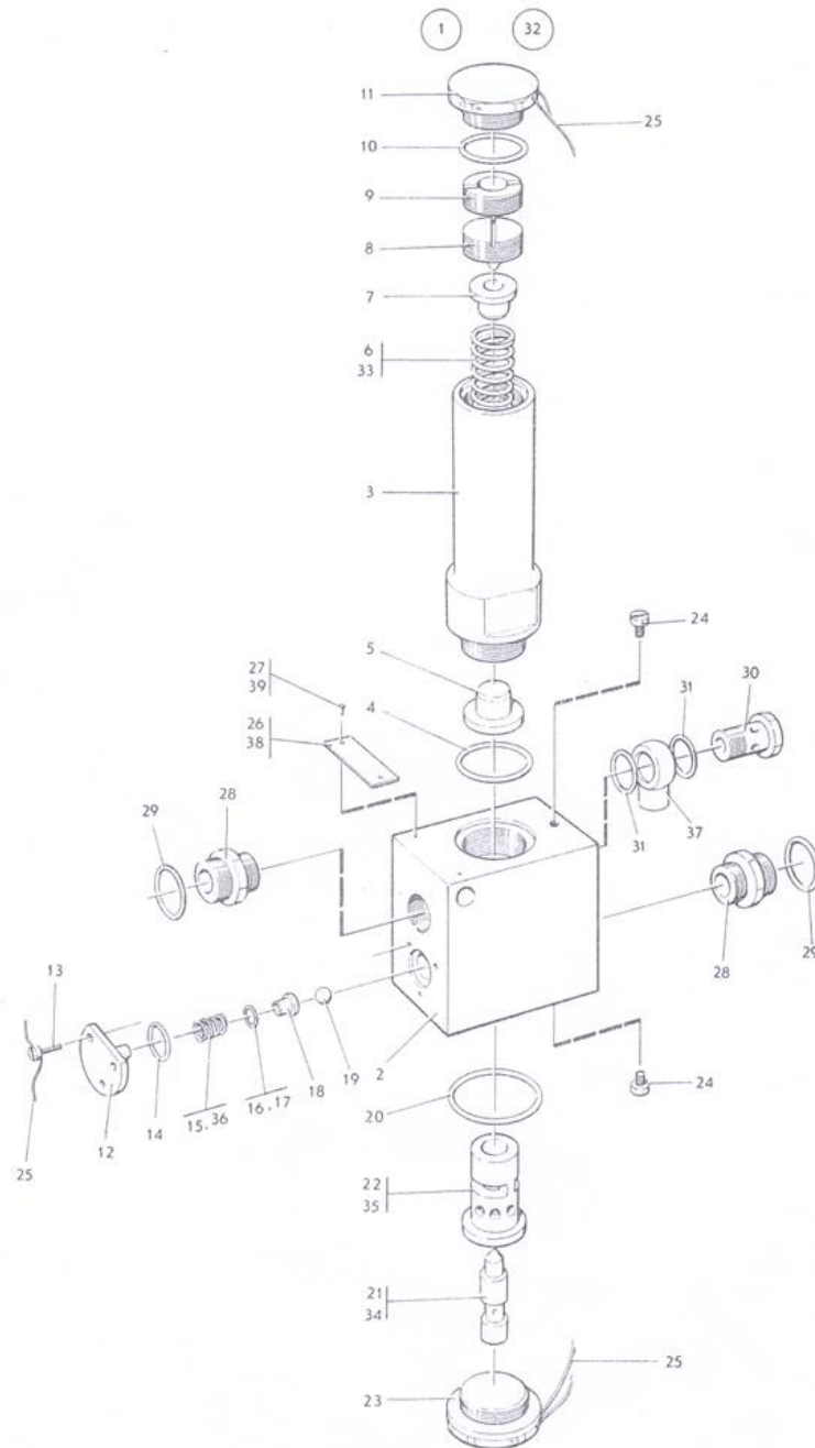
ภาพที่ 57 วาล์วลดและวาล์วบายพาส, วาล์วลด
