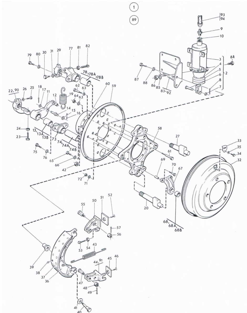
ภาพที่ 39 เบรกด้านหน้าซ้ายครบชุด
