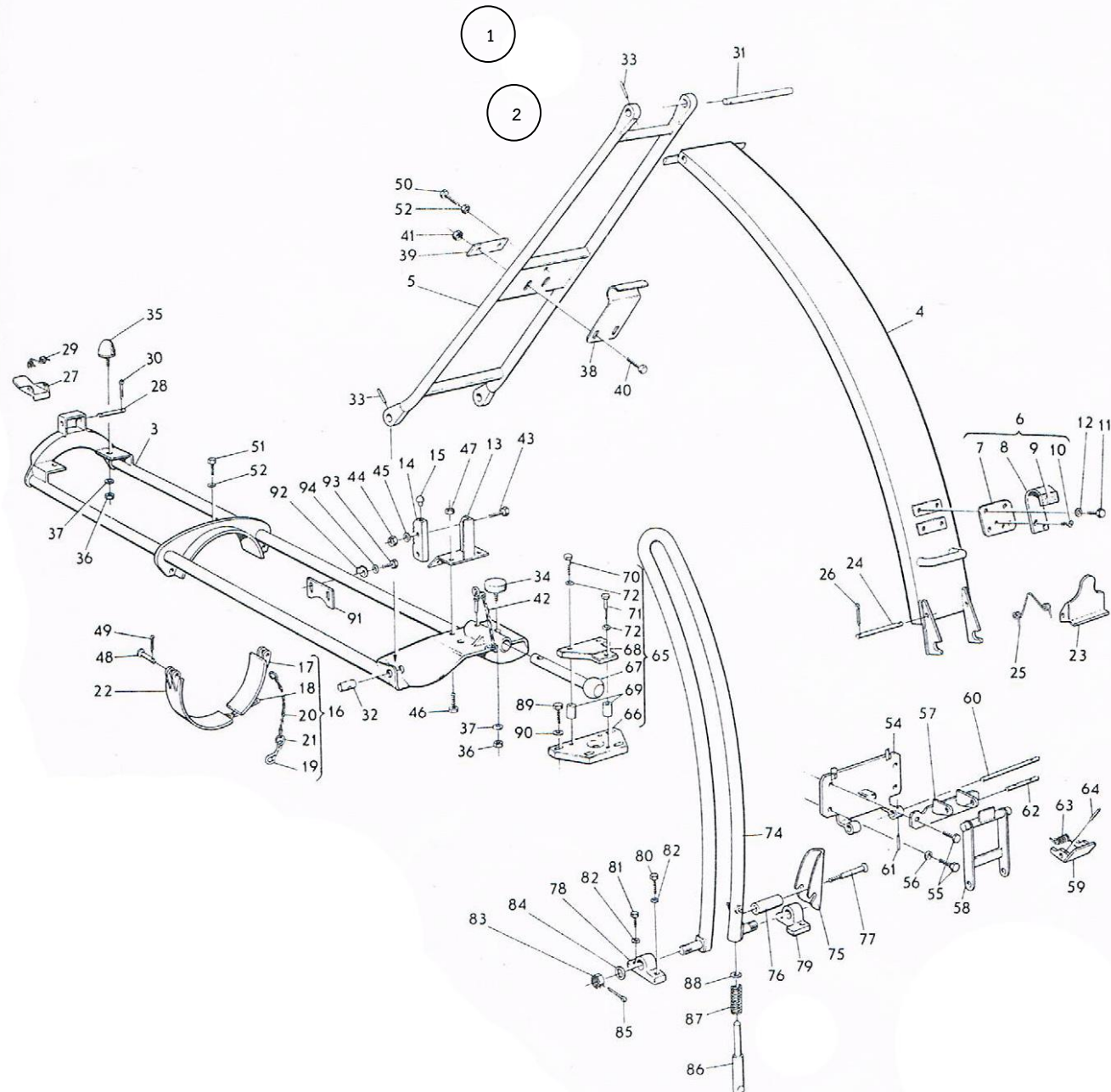
ภาพที่ 13 รายนํากระสุนครบชุด
