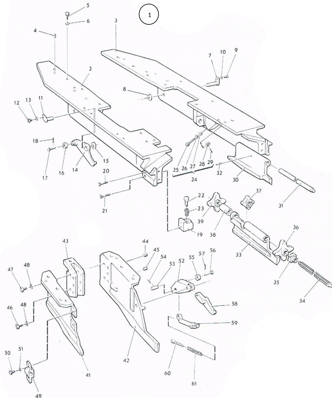
ภาพที่ 11 เครื่องป้อนกระสุนครบชุด
