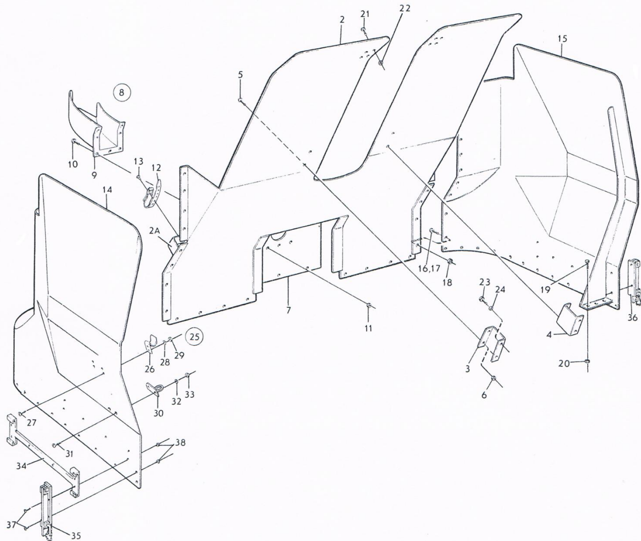
ภาพที่ 23 โล่ป็นครบชุด
