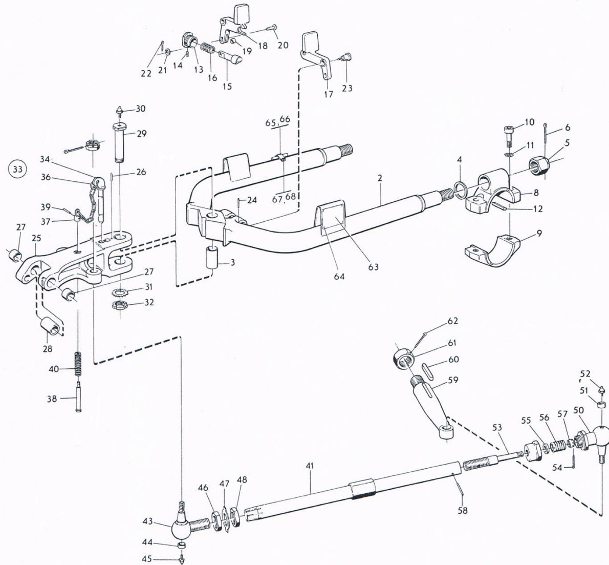
ภาพที่ 38 เฟืองบังคับเลี้ยวครบชุด
