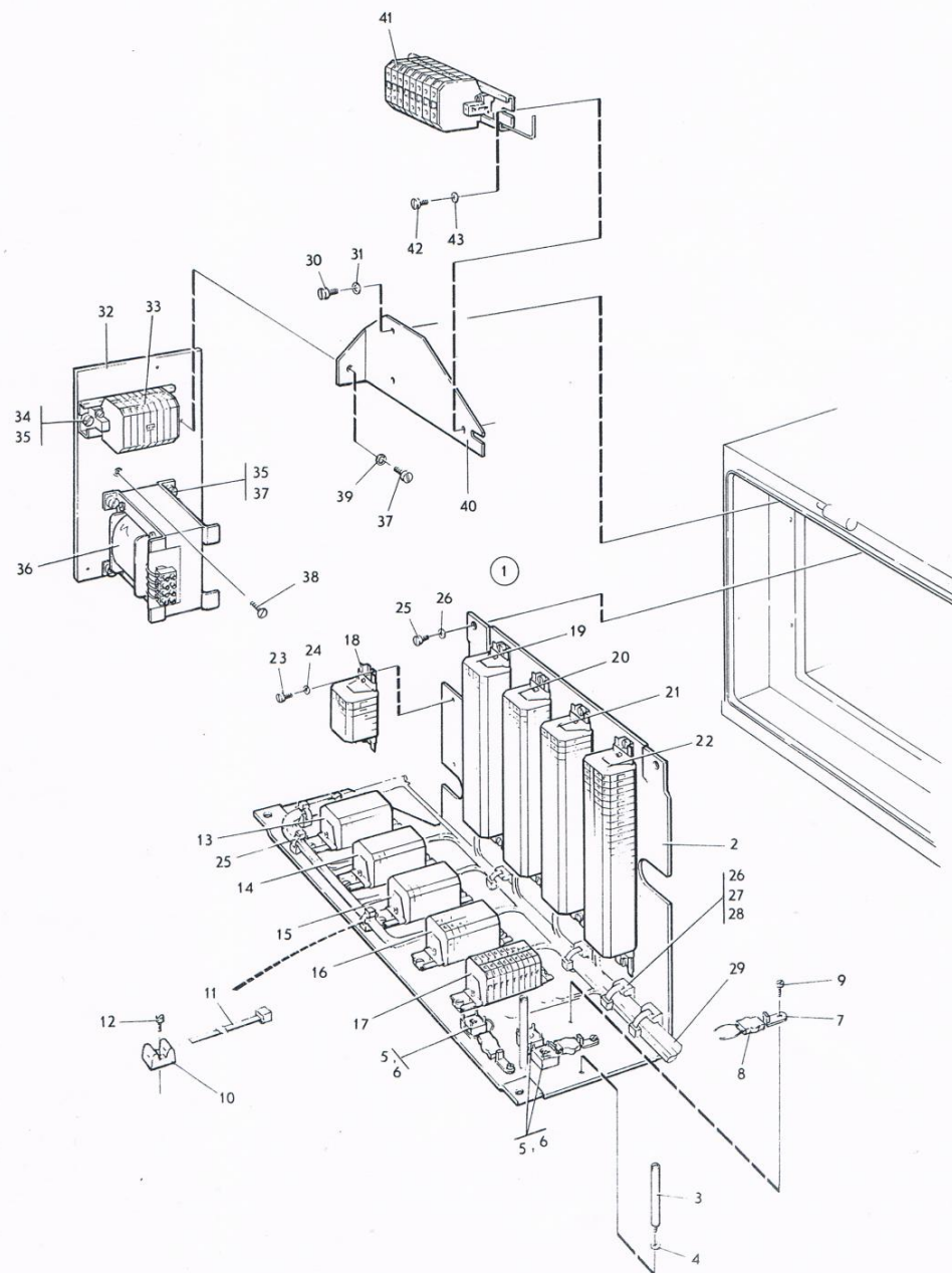
ภาพที่ 48 กล่องจ่ายไฟ, แผงรวมหัวสายไฟครบชุด, หัวรวมสายไฟครบชุด
