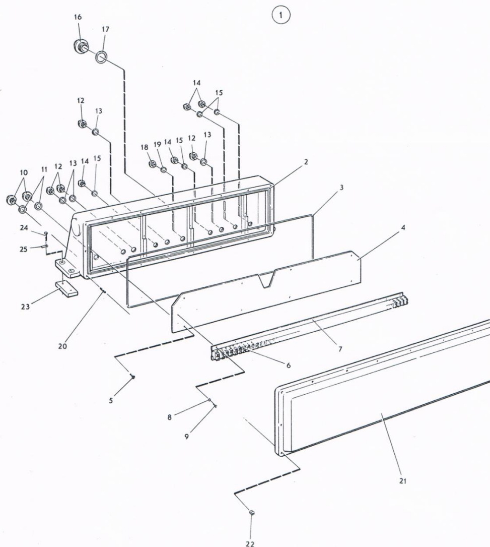
ภาพที่ 49 กล่องรวมหัวต่อสายไฟครบชุด
