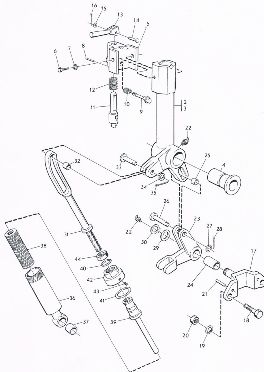
ภาพที่ 44 เบรกมือ
