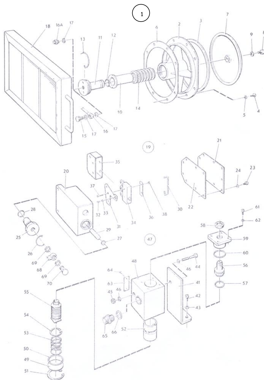
ภาพที่ 59 เทอร์โมสแตทและสวิตช์วาล์วลม, สวิตช์, เทอร์โมสแตท
