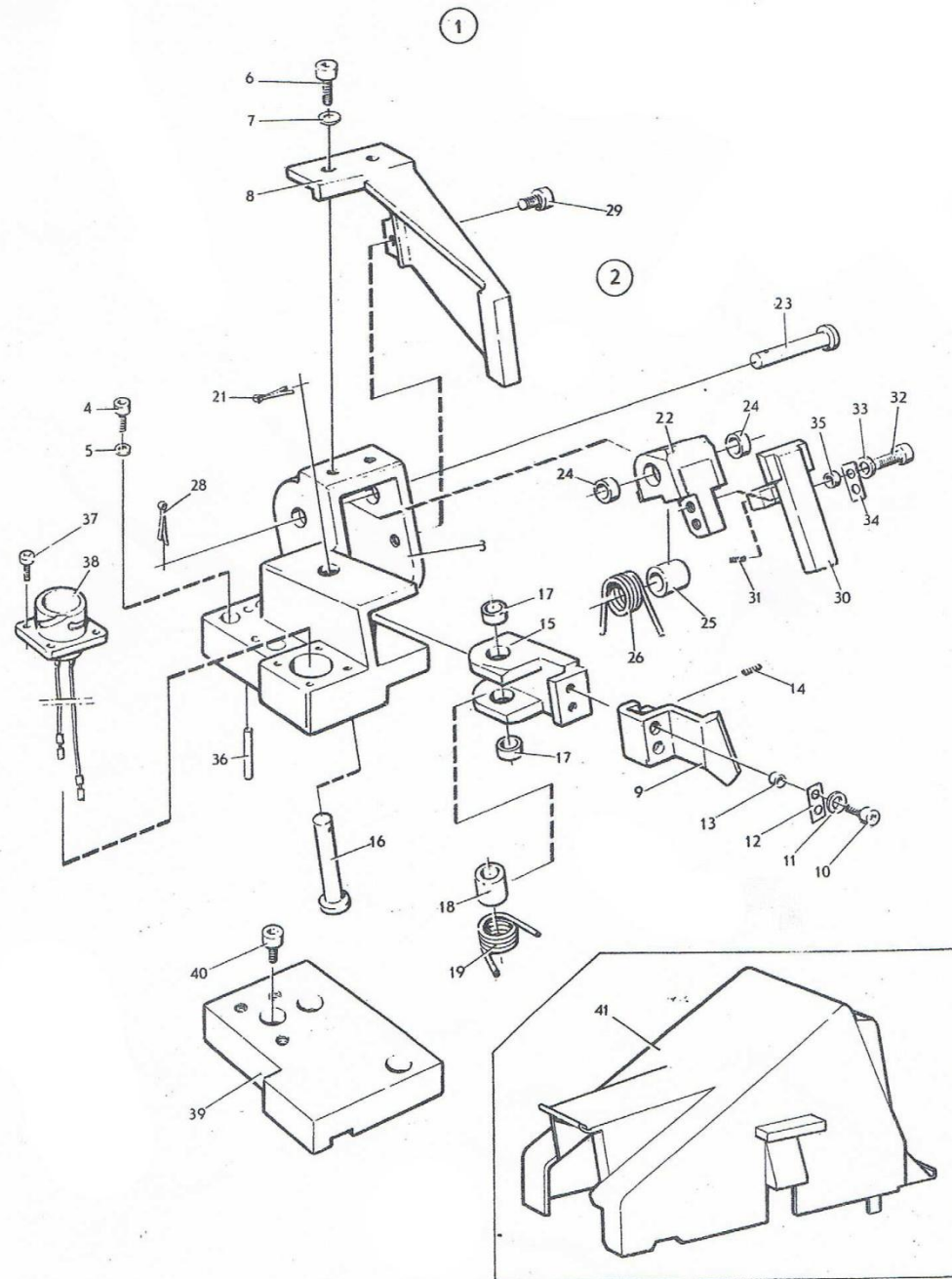
ภาพที่ 17 เครื่องตั้งขนวนวีทีครบชุด
