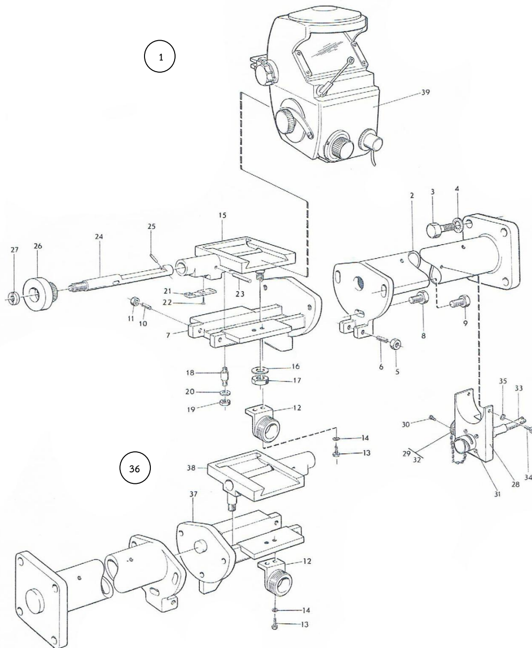
ภาพที่ 18 ฐานยึดกล้องเล็งด้านซ้ายครบชุด
