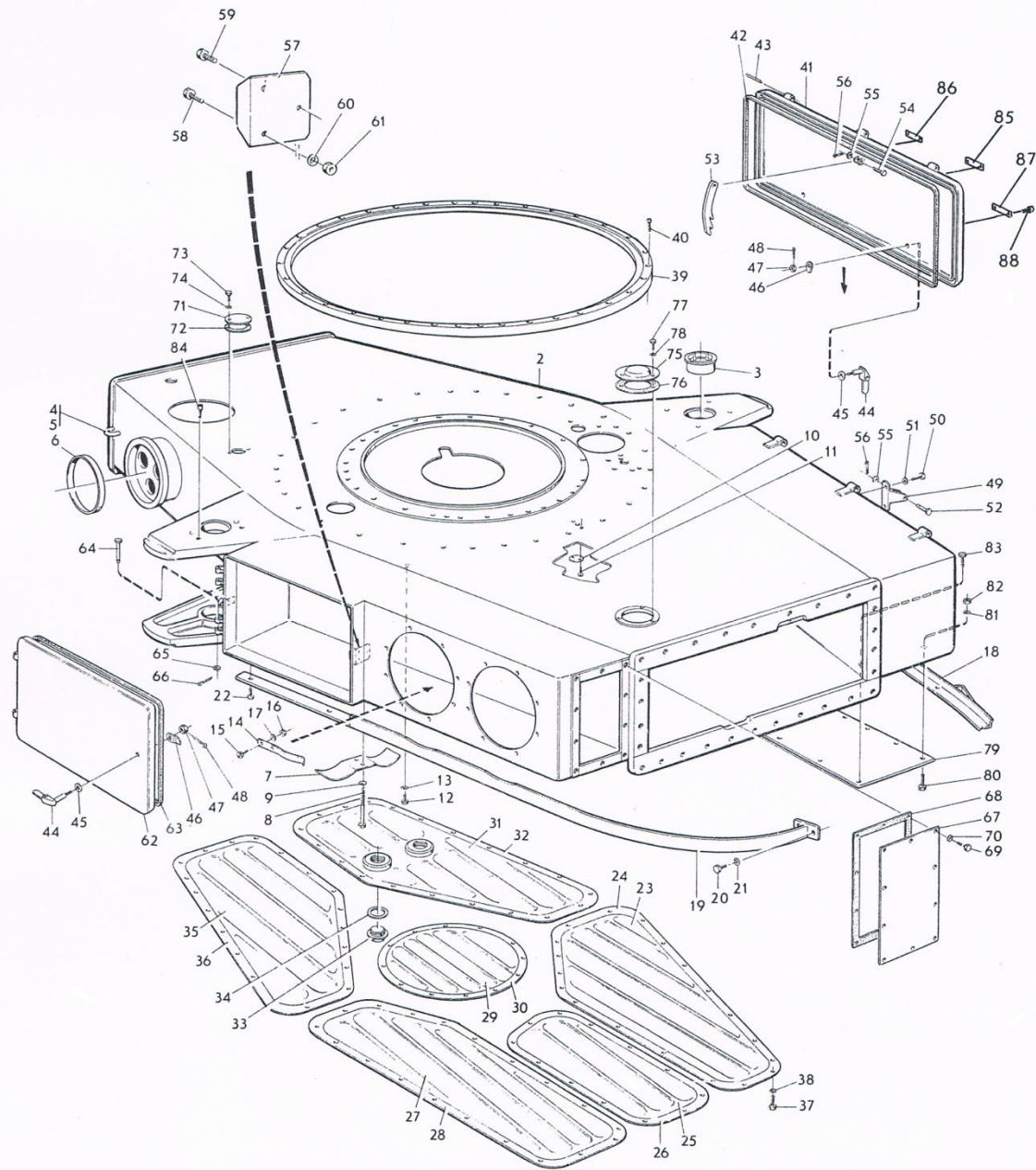
ภาพที่ 25 แคร่กลางครบชุด
