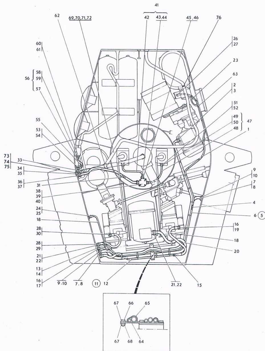
ภาพที่ 52 ส่วนติดตั้งระบบไฟฟ้า
