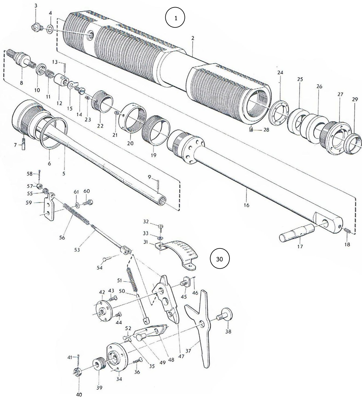
ภาพที่ 16 เครื่องรับแรงสะท้อนถอยหลัง
