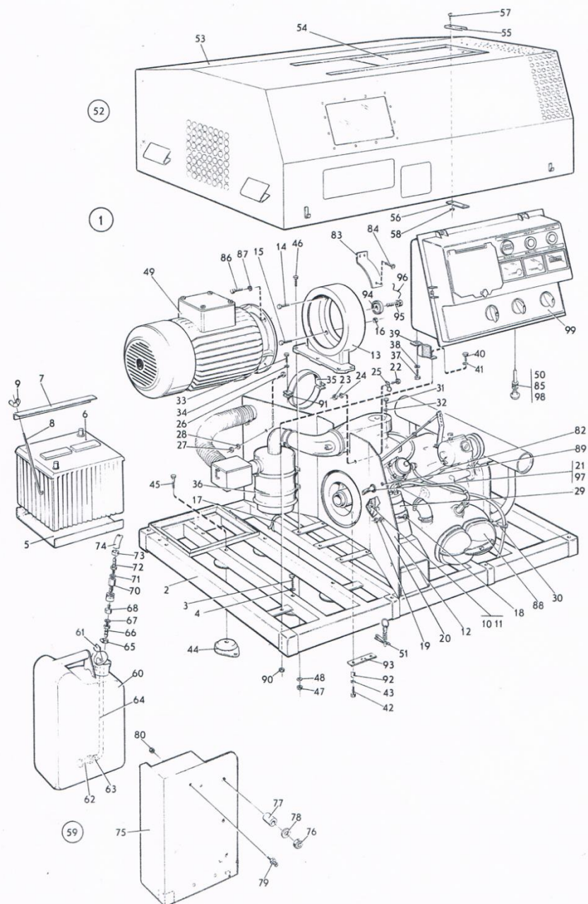
ภาพที่ 82 ฝาครอบเครื่องปั๊มนไฟครบชุด, ชุดแทนบยัด, ถังเชื้อเพลิงครบชุด
