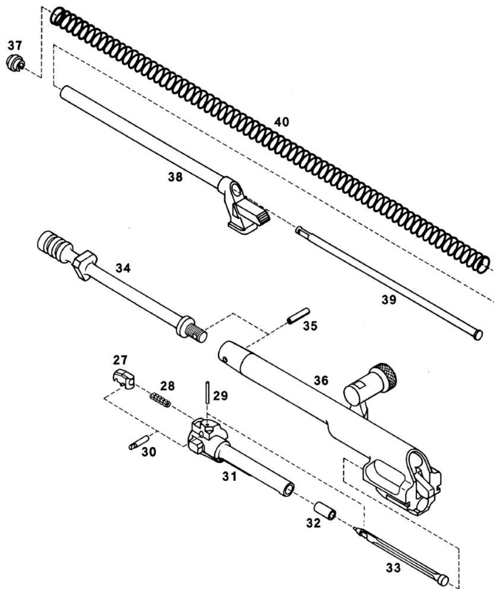
ภาพที่ 5 ส่วนเคลื่อนถอย
