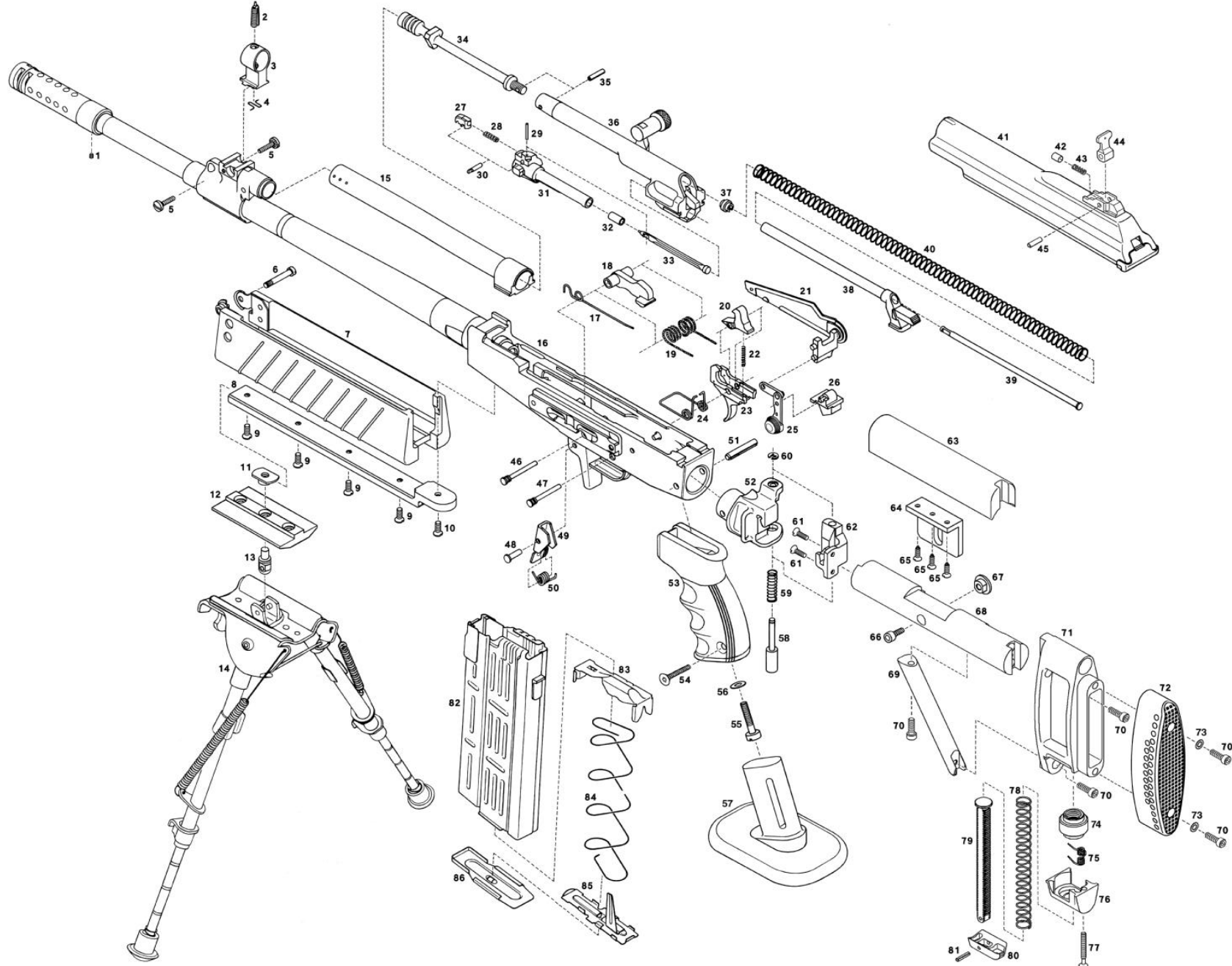
ภาพที่ 1 ปืนชুমยิงกาลิล ขนาด 7.62X51 มม.
