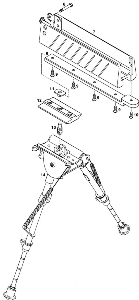
ภาพที่ 6 ชุดประกับรองมือและขาทราย
