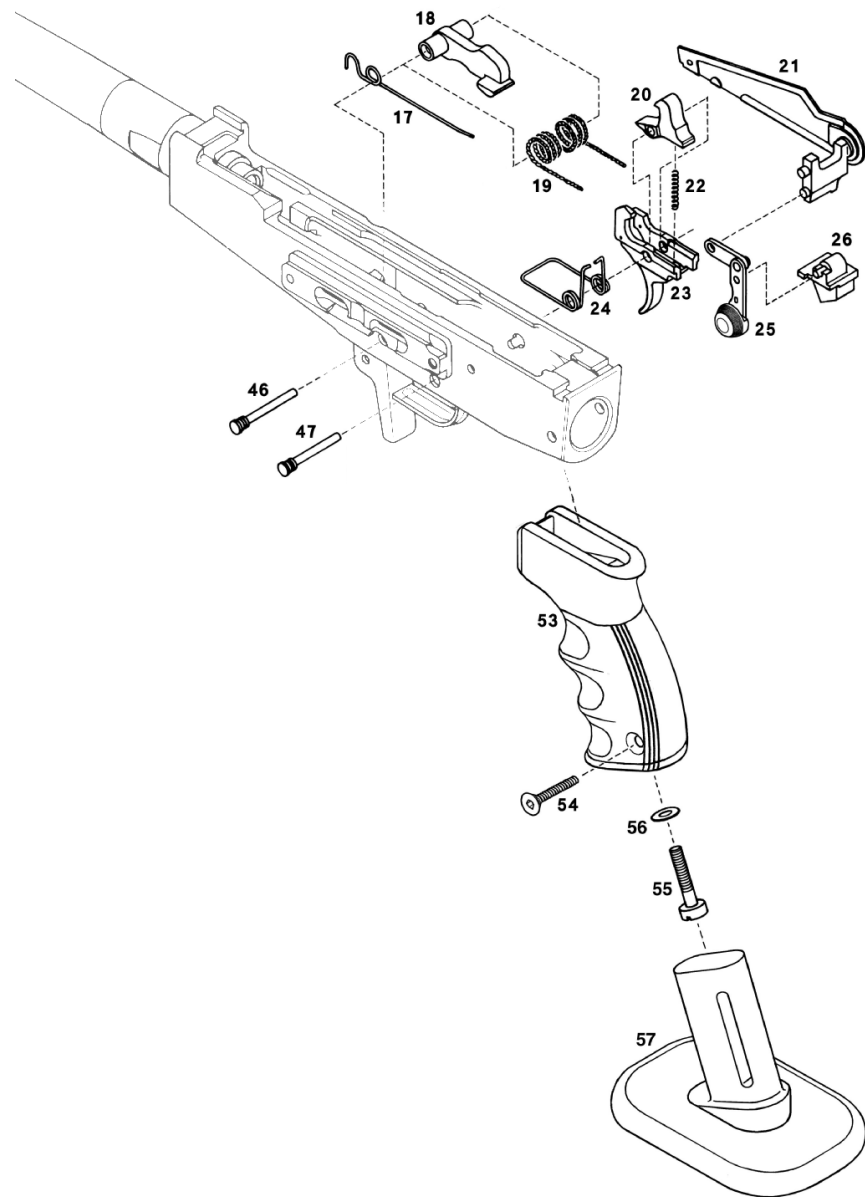
ภาพที่ 4 ด้ามปืนและห้ามไก
