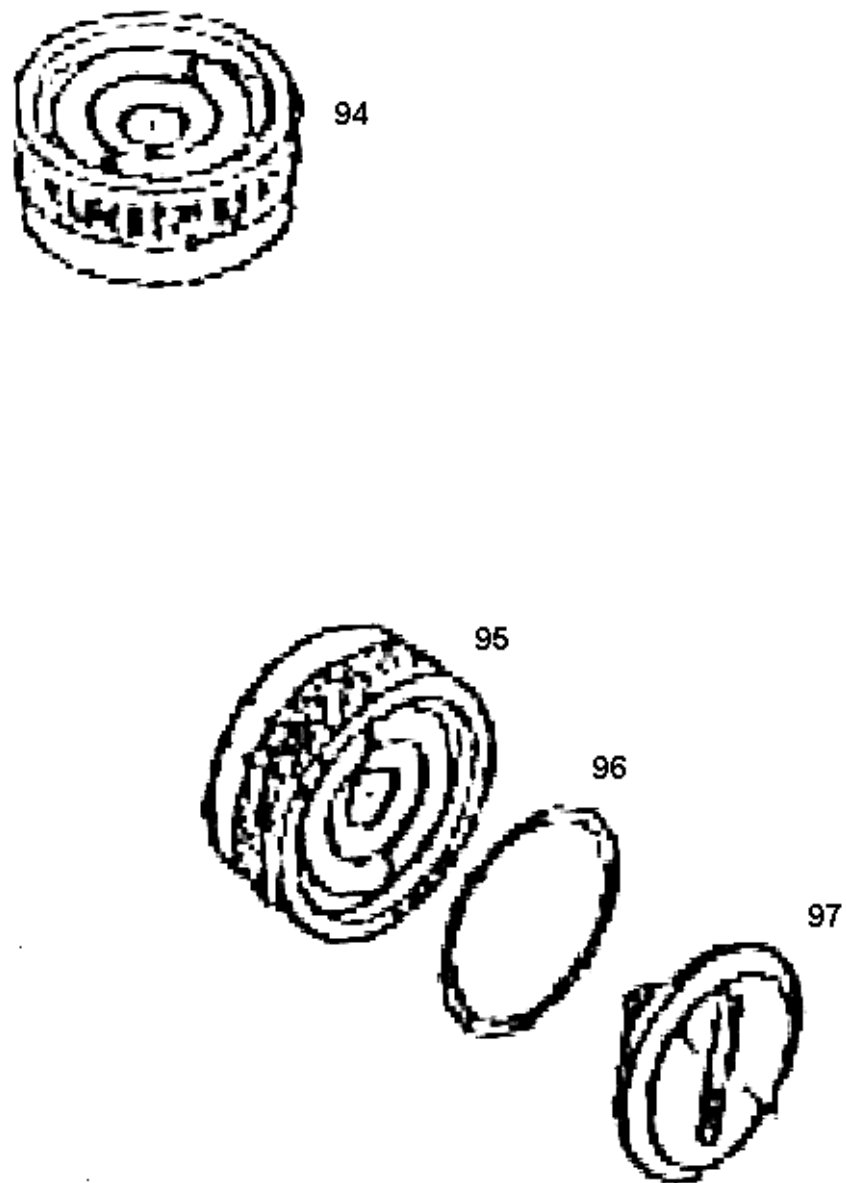
ภาพที่ 10 ชิ้นส่วนของกล่องนิมร็อด
