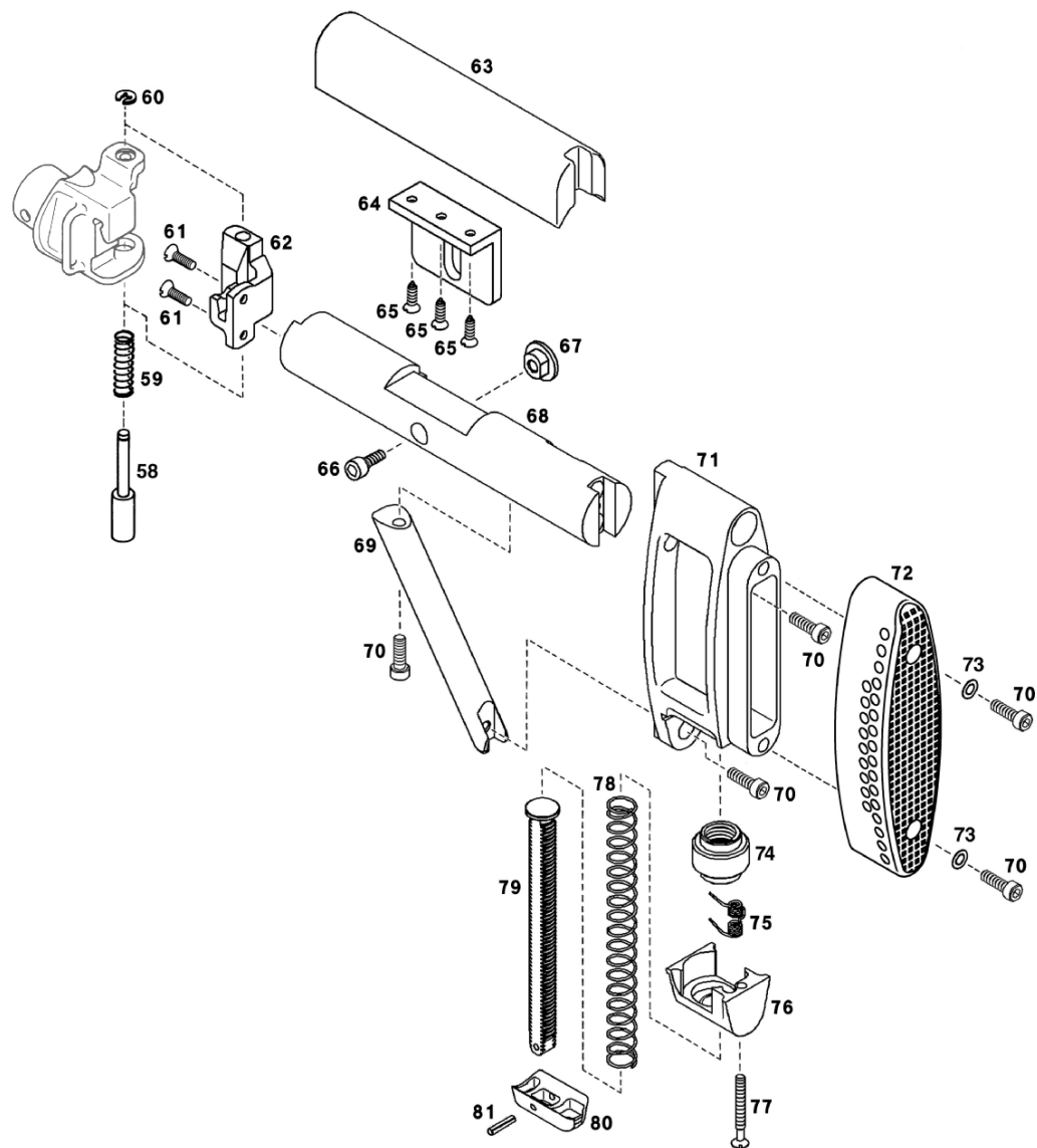
ภาพที่ 7 ชุดพานท้าย
