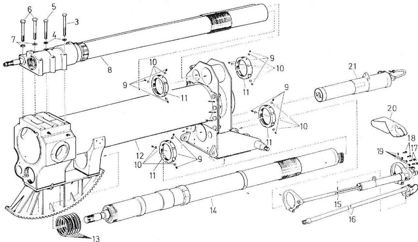
ภาพที่ 14 ชุดเครื่องรับแรงถอย
