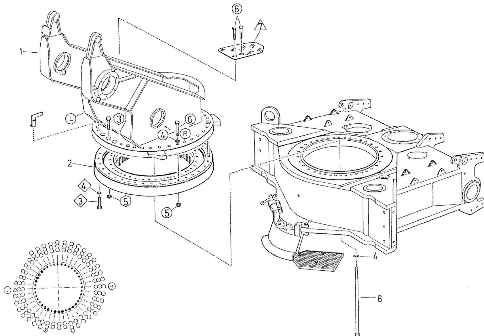
ภาพที่ 4 แคร่บนฐานรองเส้นทางทิศ
