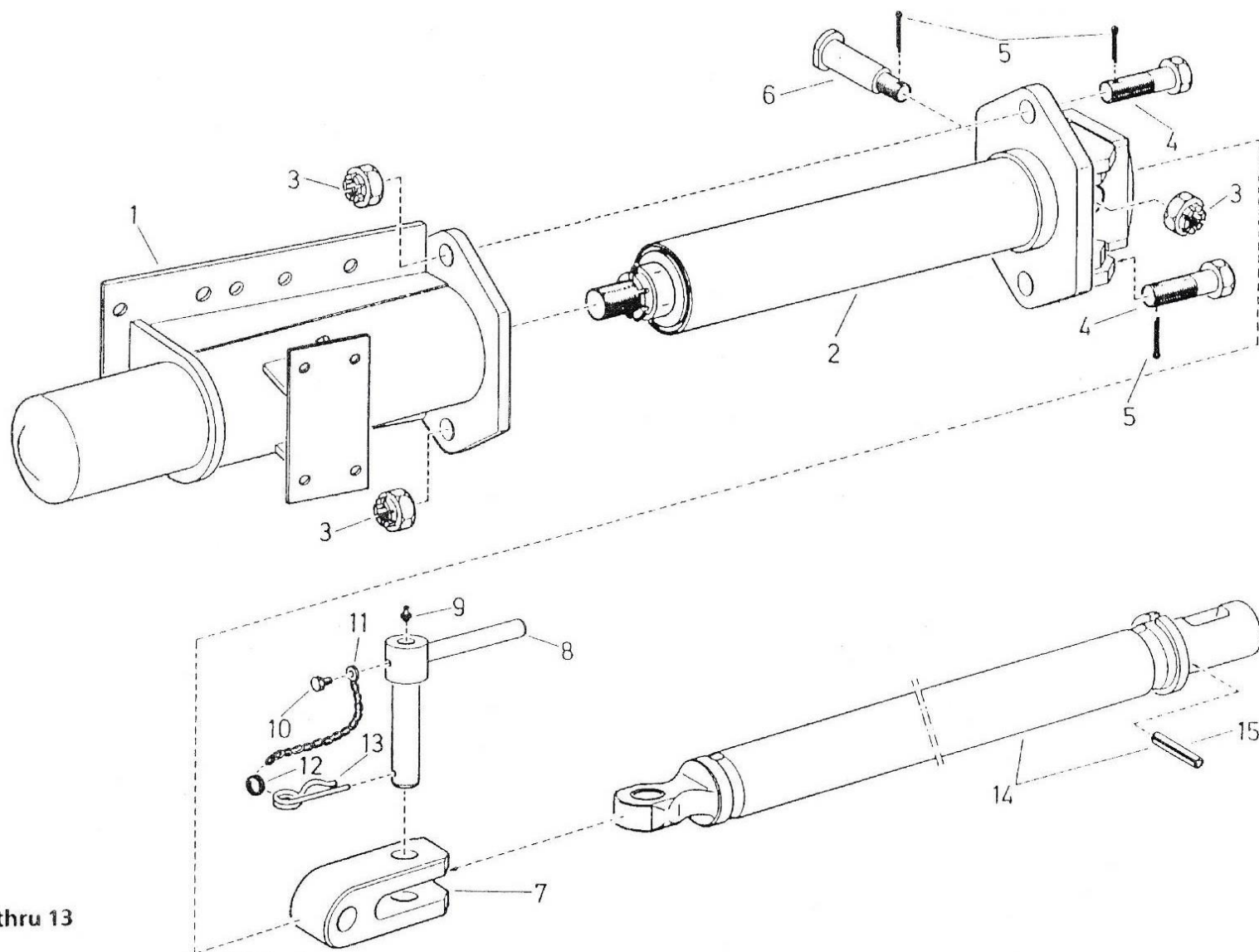
ภาพที่ 30 ปลอกต่อระบบบังคับเลี้ยว
