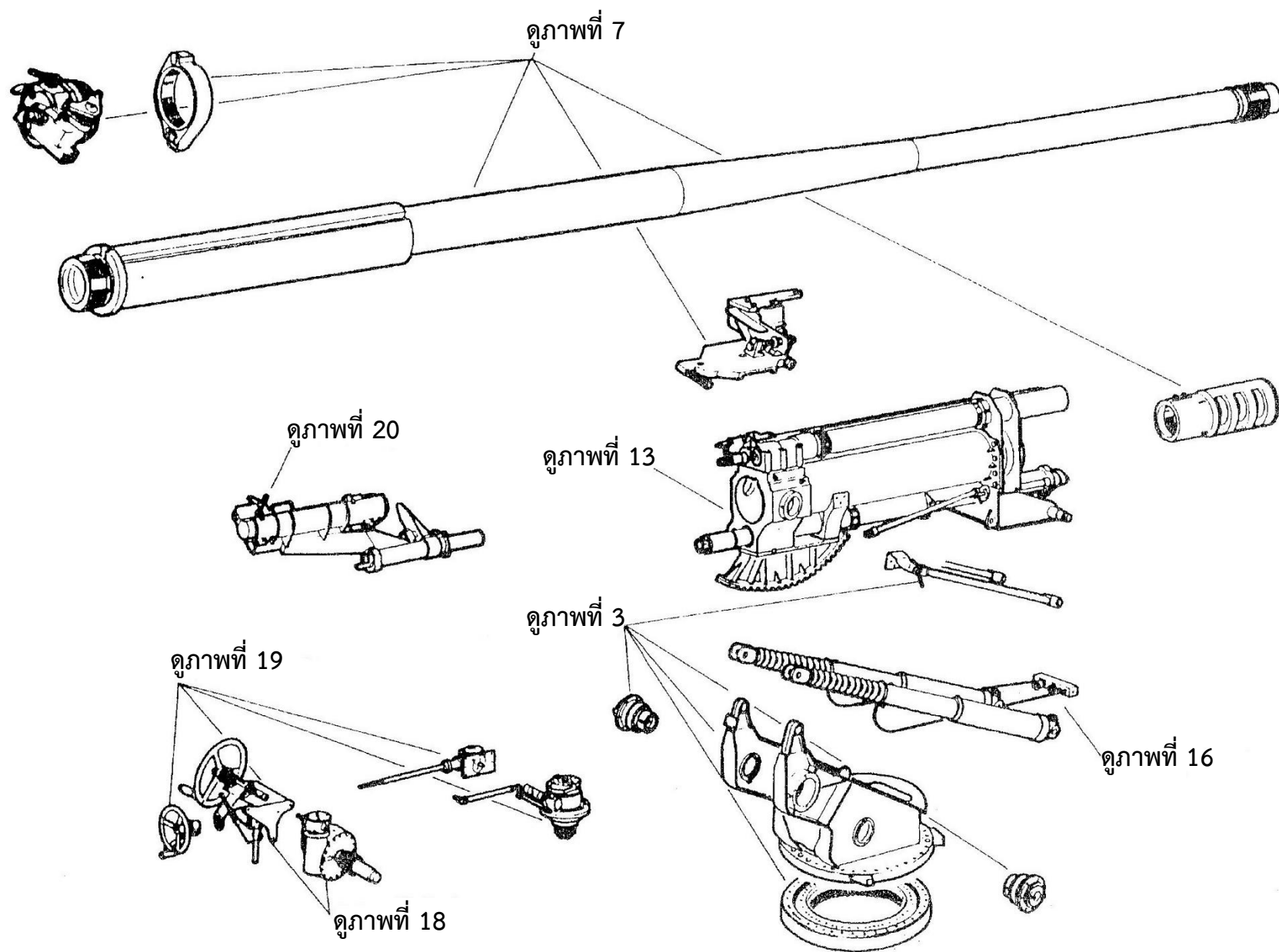
ภาพที่ 1 ชุดแคว่ป็นส่วนบนครบชุด
