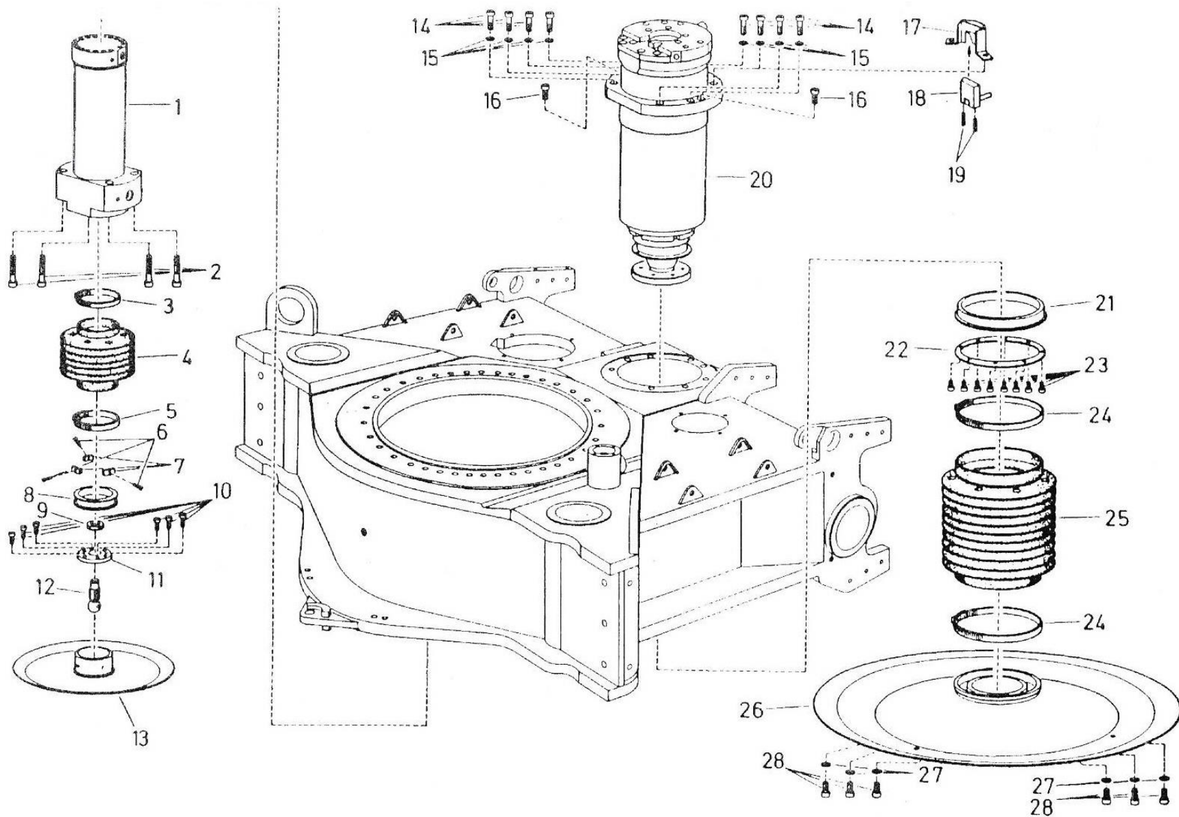
ภาพที่ 39 ชุดแม่แรงหลักและแม่แรงช่วย
