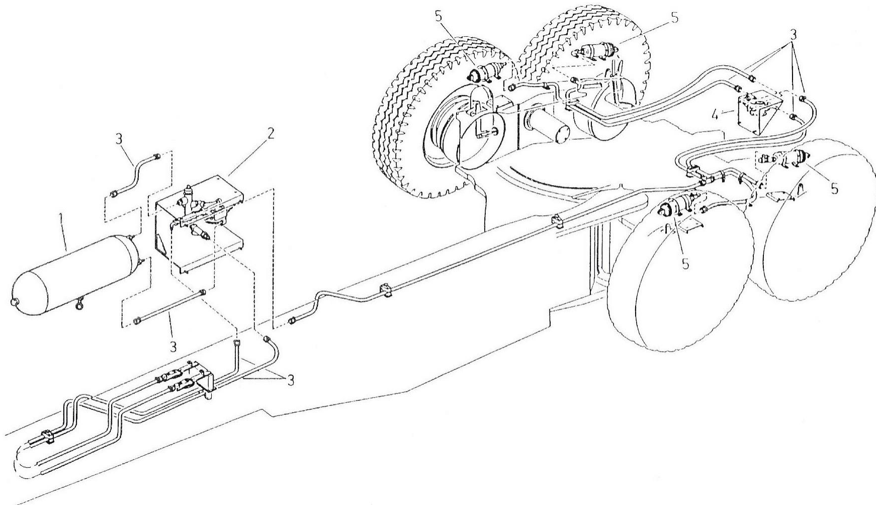
ภาพที่ 37 ระบบเบรกลม
