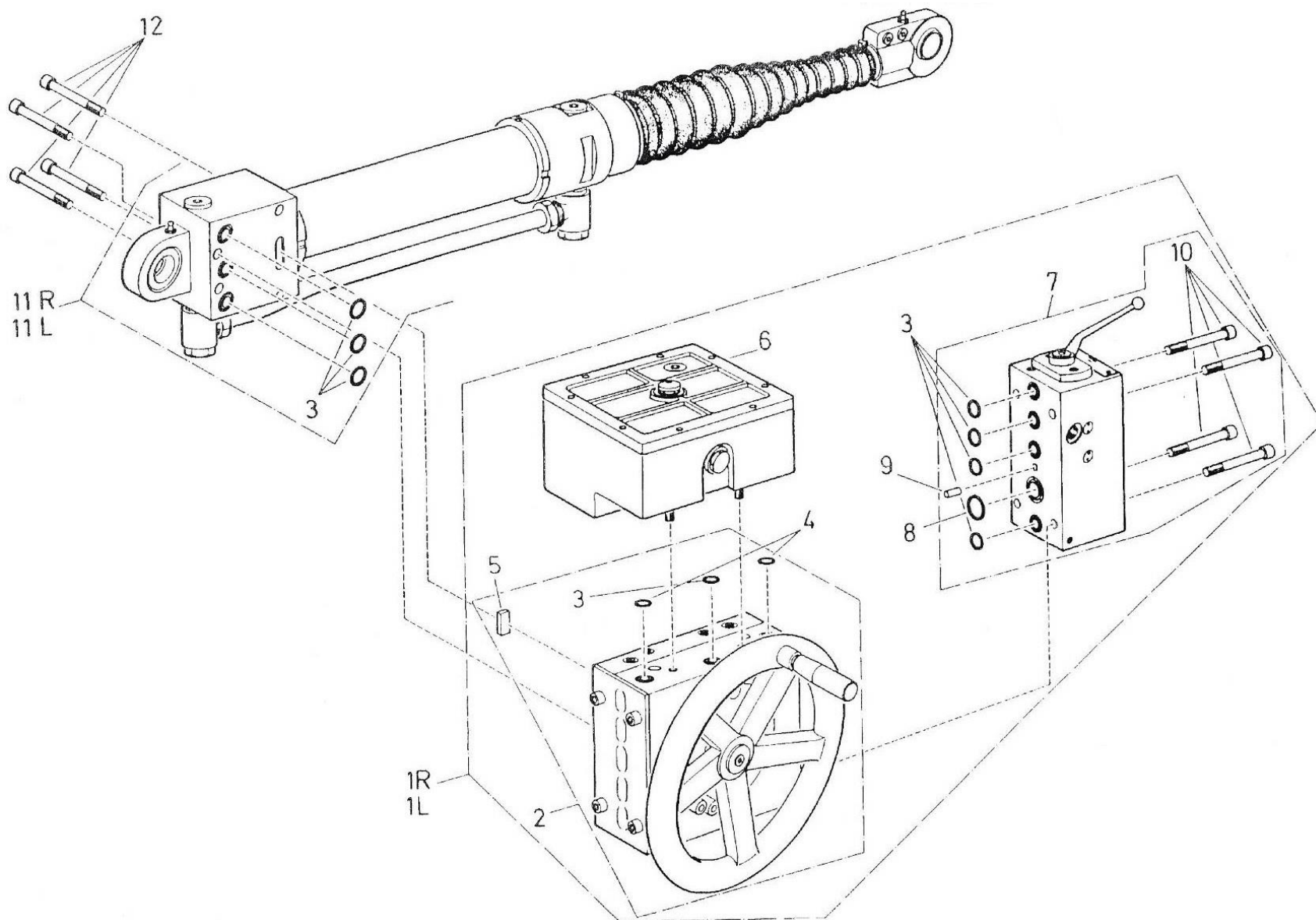
ภาพที่ 40 ล้อยกรางปืน - ชุดไฮดรอลิก
