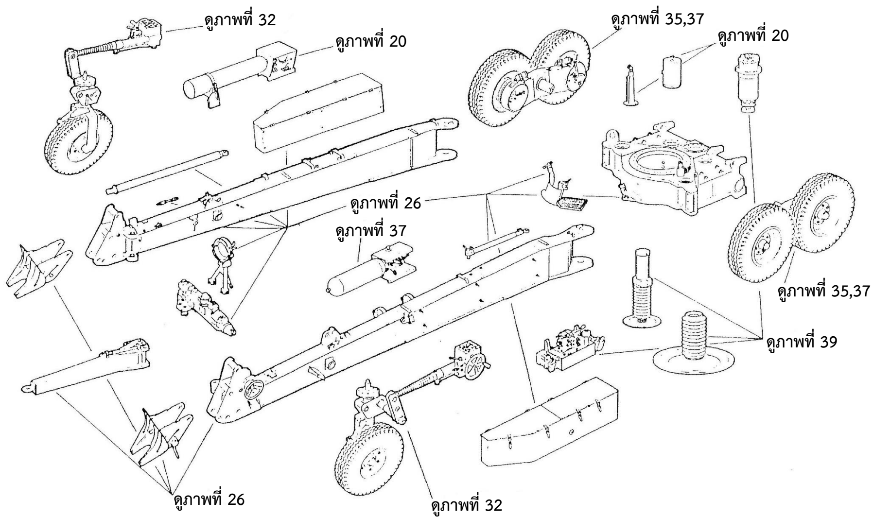
ภาพที่ 2 แครป็นส่วนล่าง
