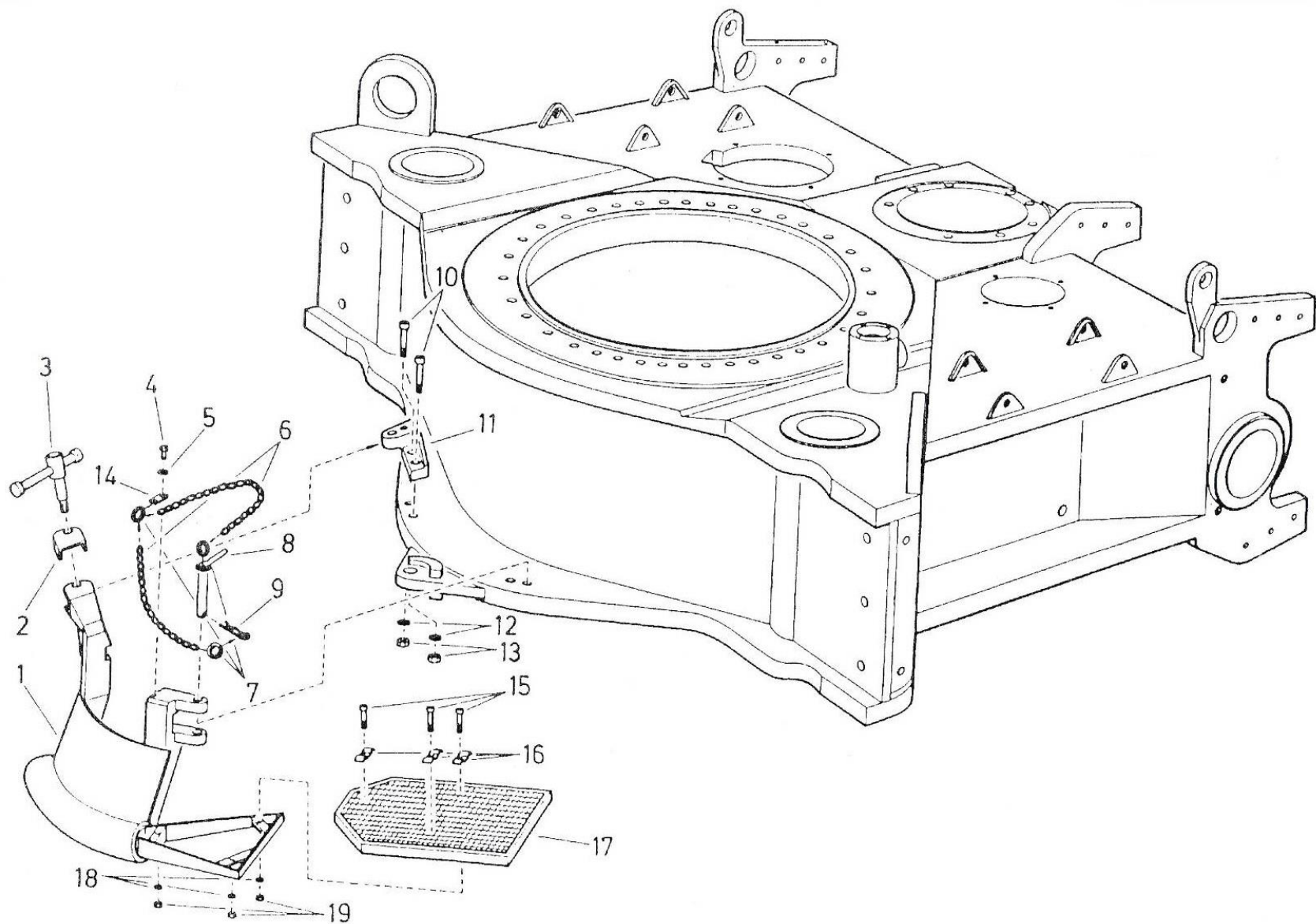
ภาพที่ 29 ก้านชน ฐานปั๊นพลึง
