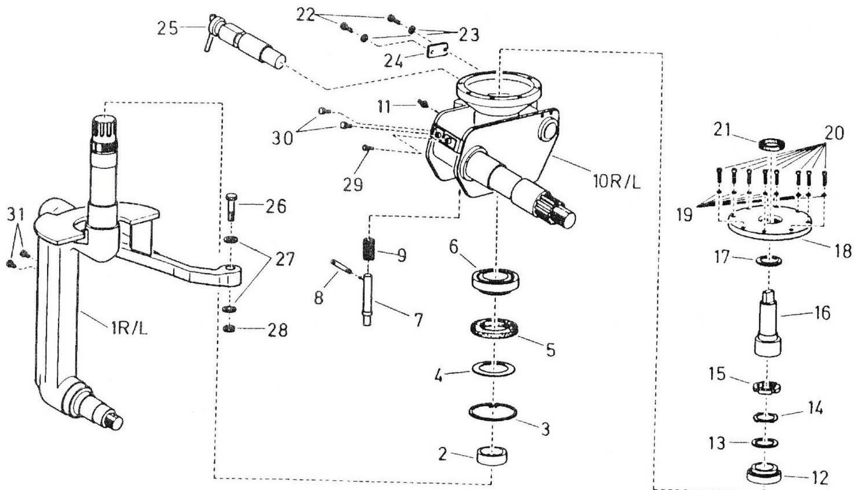
ภาพที่ 33 คั่นบังคับเลี้ยวและจุดหมุน
