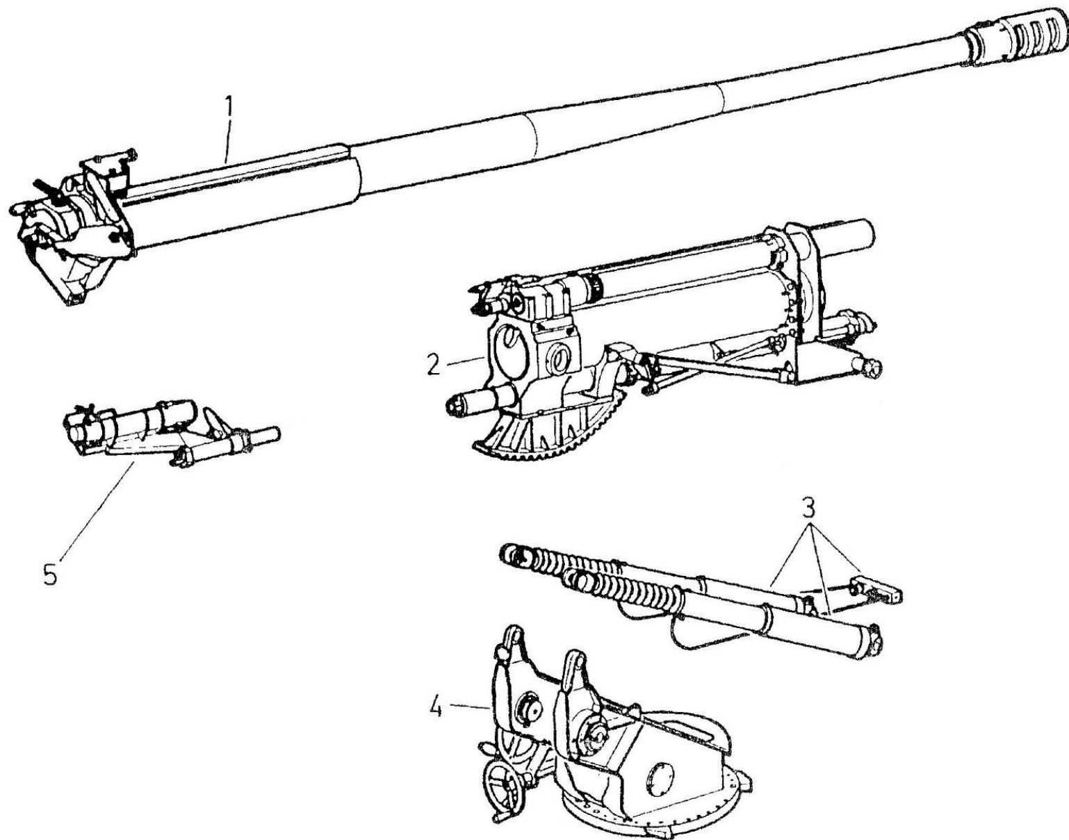
ภาพที่ 3 แคร่ปืนส่วนบน อาวุธ เครื่องรับแรงถอย เครื่องป้อนกระสุน เครื่องช่วยให้มุมทางสูง
