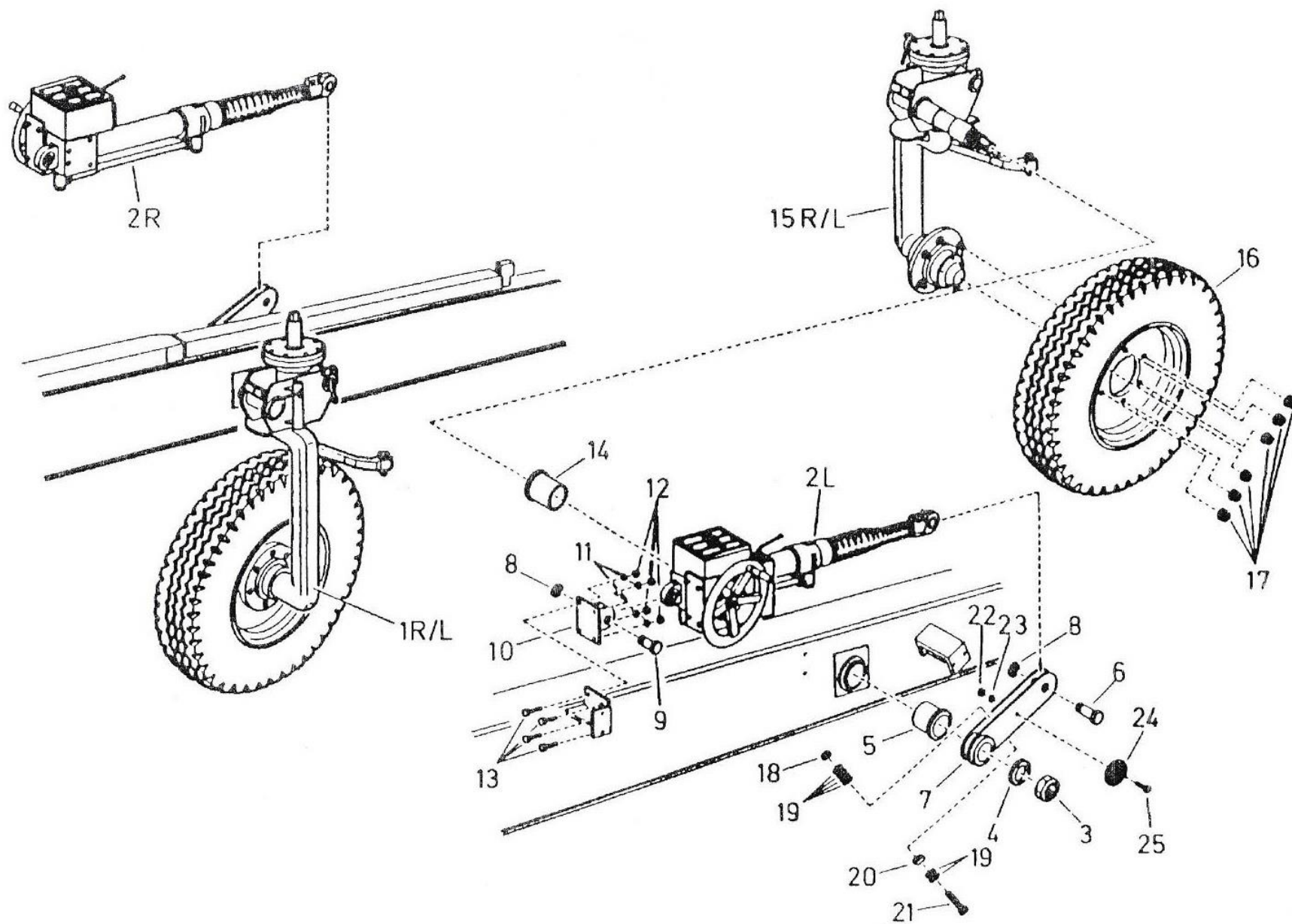
ภาพที่ 32 ล้อยกรางปืน
