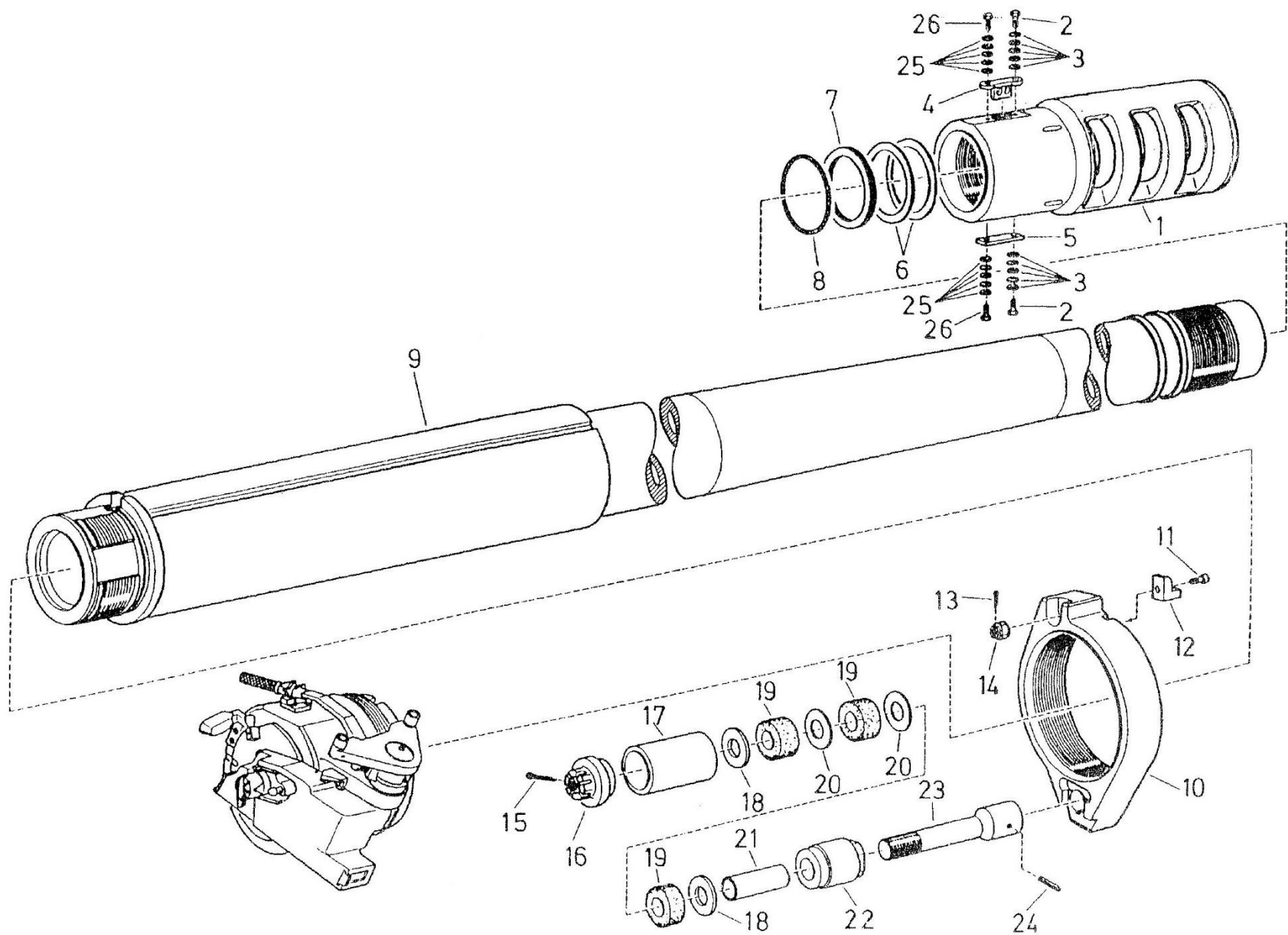
ภาพที่ 8 ลำกล้องปืน ระบบรับแรงถอย ปลอกยิงแรงถอย
