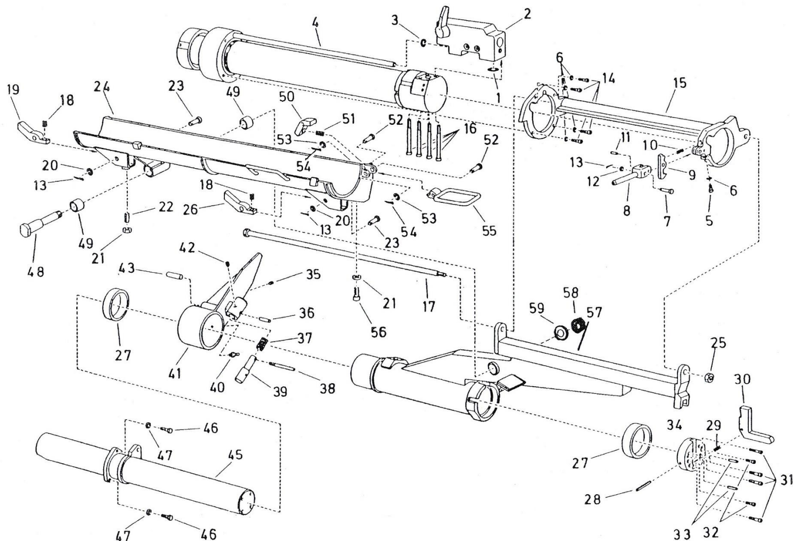
ภาพที่ 21 ชุดเครื่องบรรจุกระสุน
