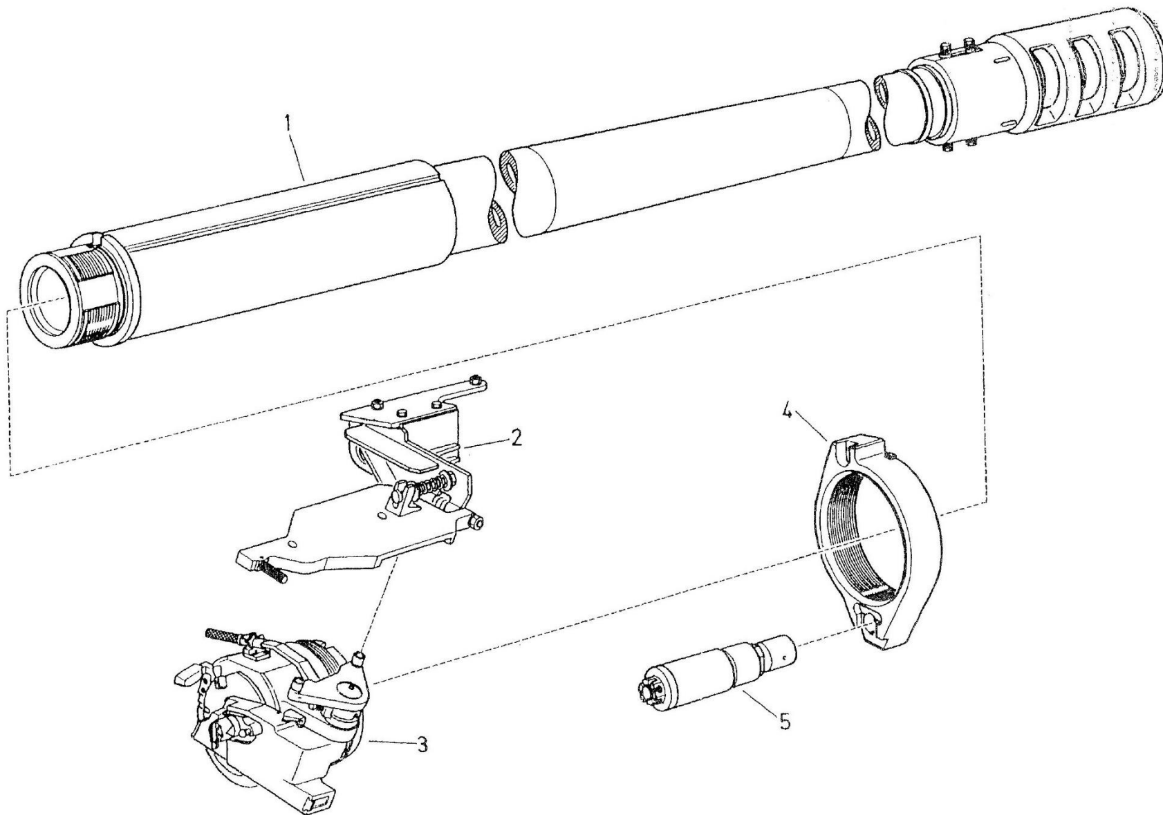
ภาพที่ 7 ลำกล้องปั๊มใหญ่ขนาด 155/45
