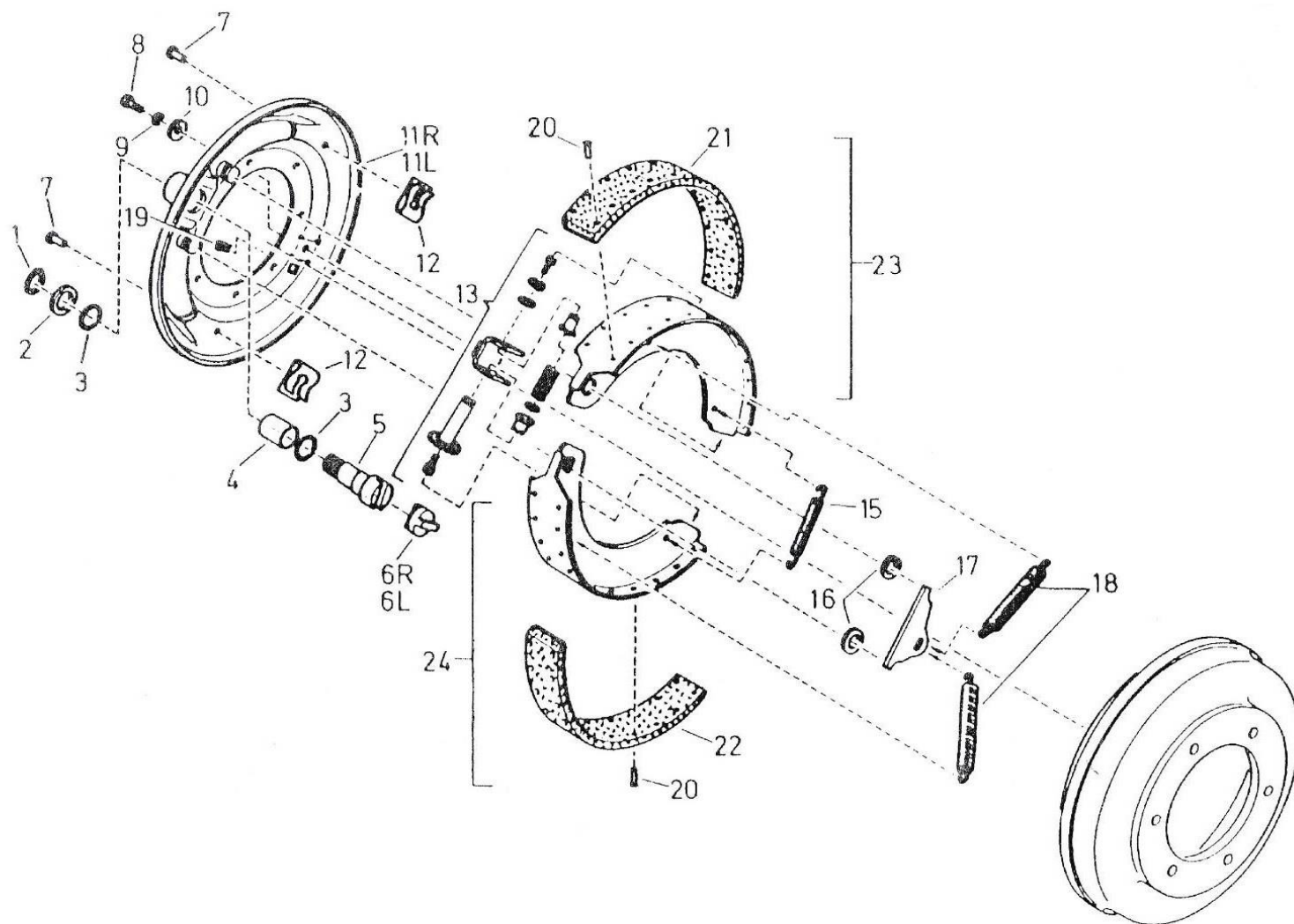
ภาพที่ 36 องค์ประกอบภายในเบรก
