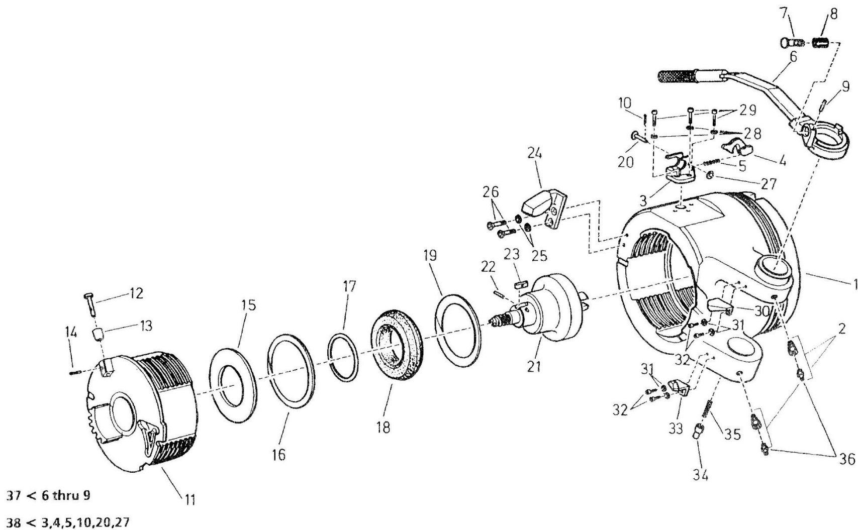
ภาพที่ 10 เรือนเครื่องปิดท้าย แท่งเครื่องปิดท้าย กลไกเรือนเครื่องปิดท้าย
