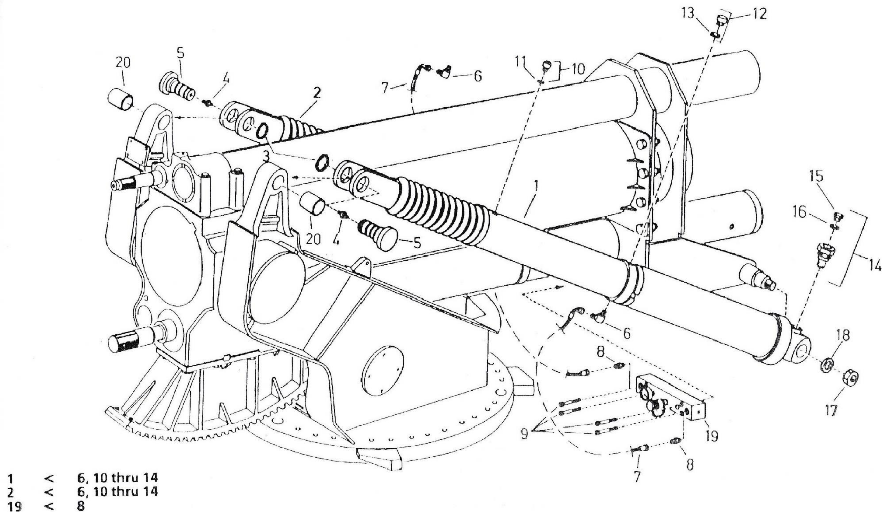
ภาพที่ 16 เครื่องช่วยให้มุมทางสูง
