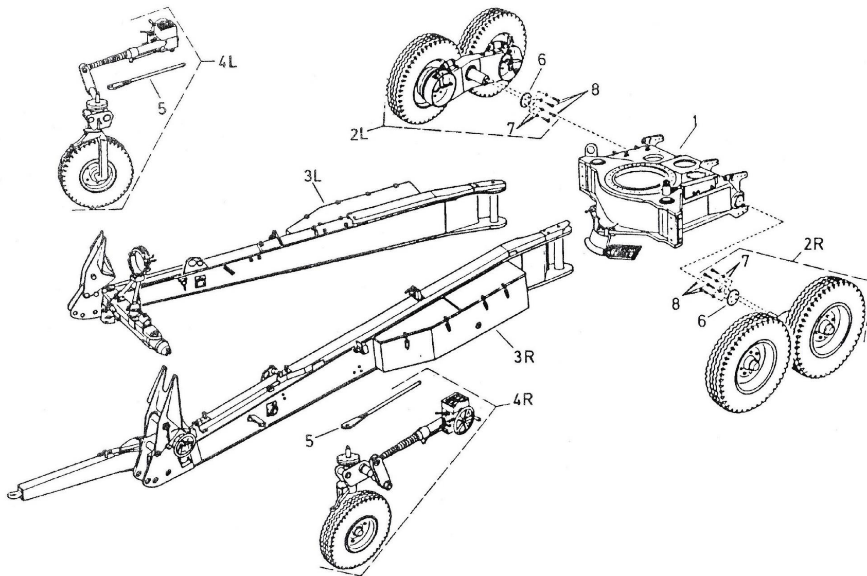
ภาพที่ 26 แคร่ล่าง
