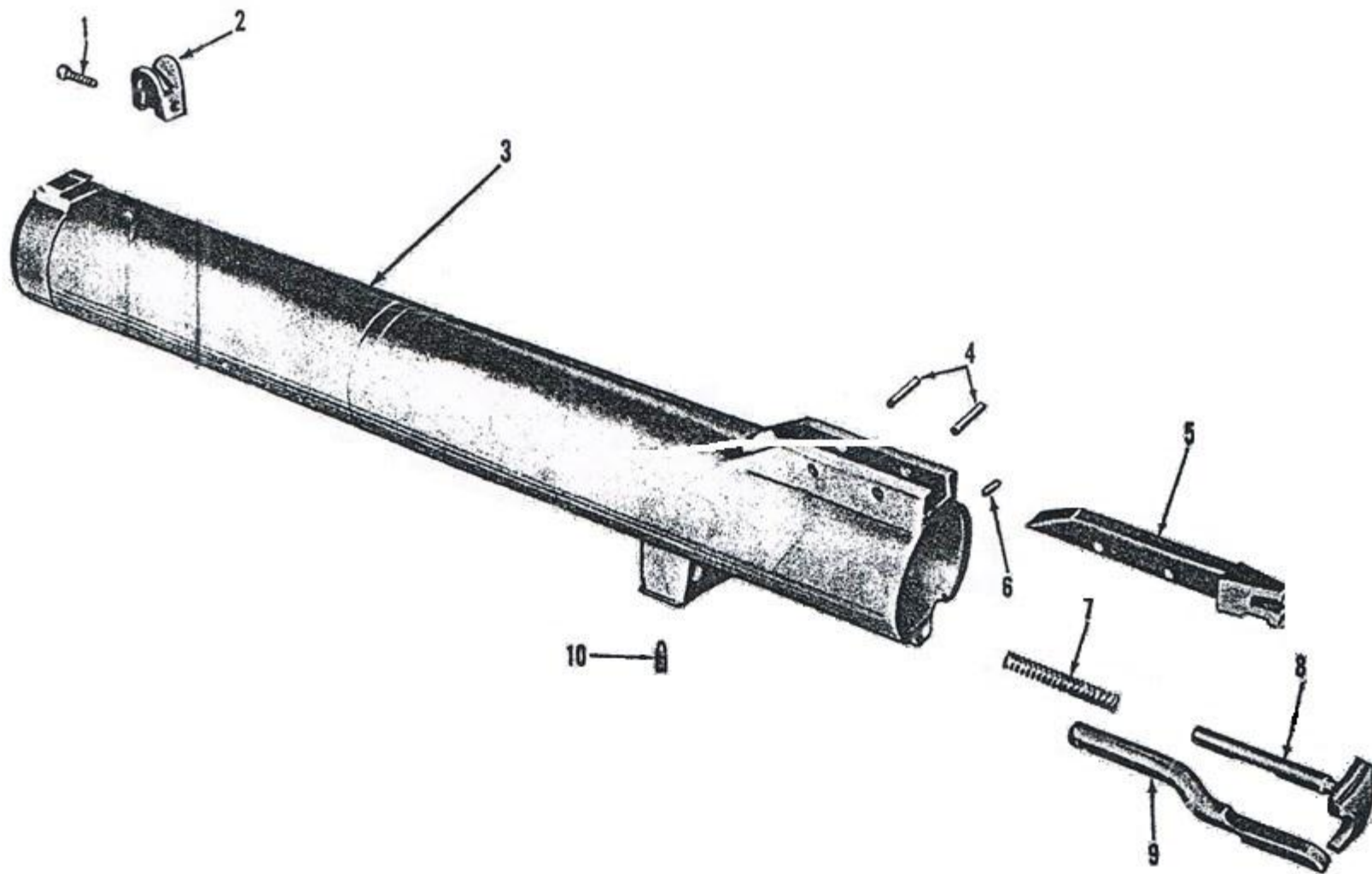
ภาพที่ 2 ชุดลำกล้องและศูนย์หน้า
