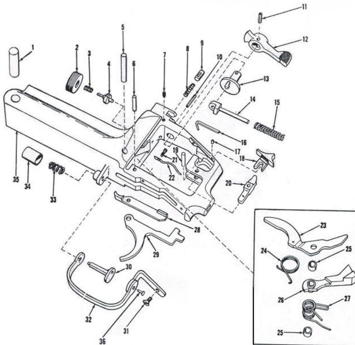
ภาพที่ 4 ชุดโครงป็น
