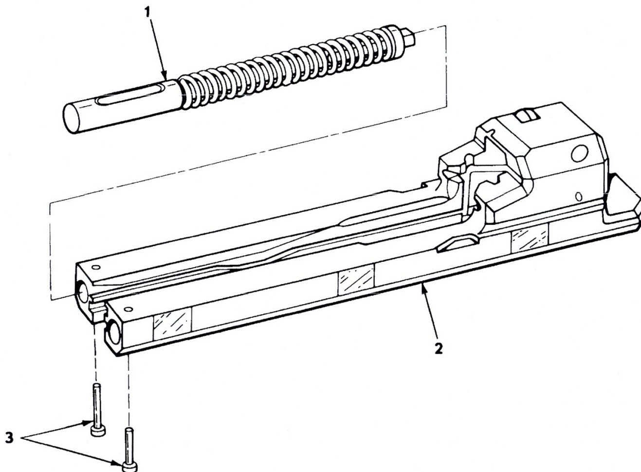
ภาพที่ 10 ชุดโครงต่อท้ายลำกล้อง
