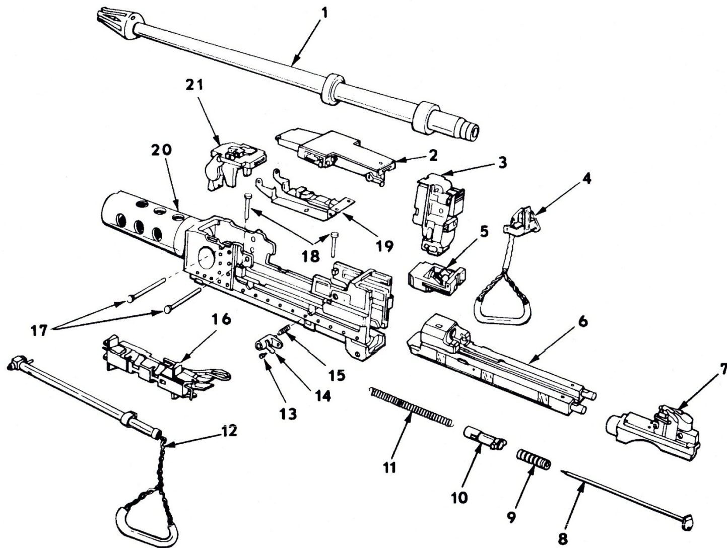
ภาพที่ 1 ปืนกล ขนาด .50 นิ้ว M85
