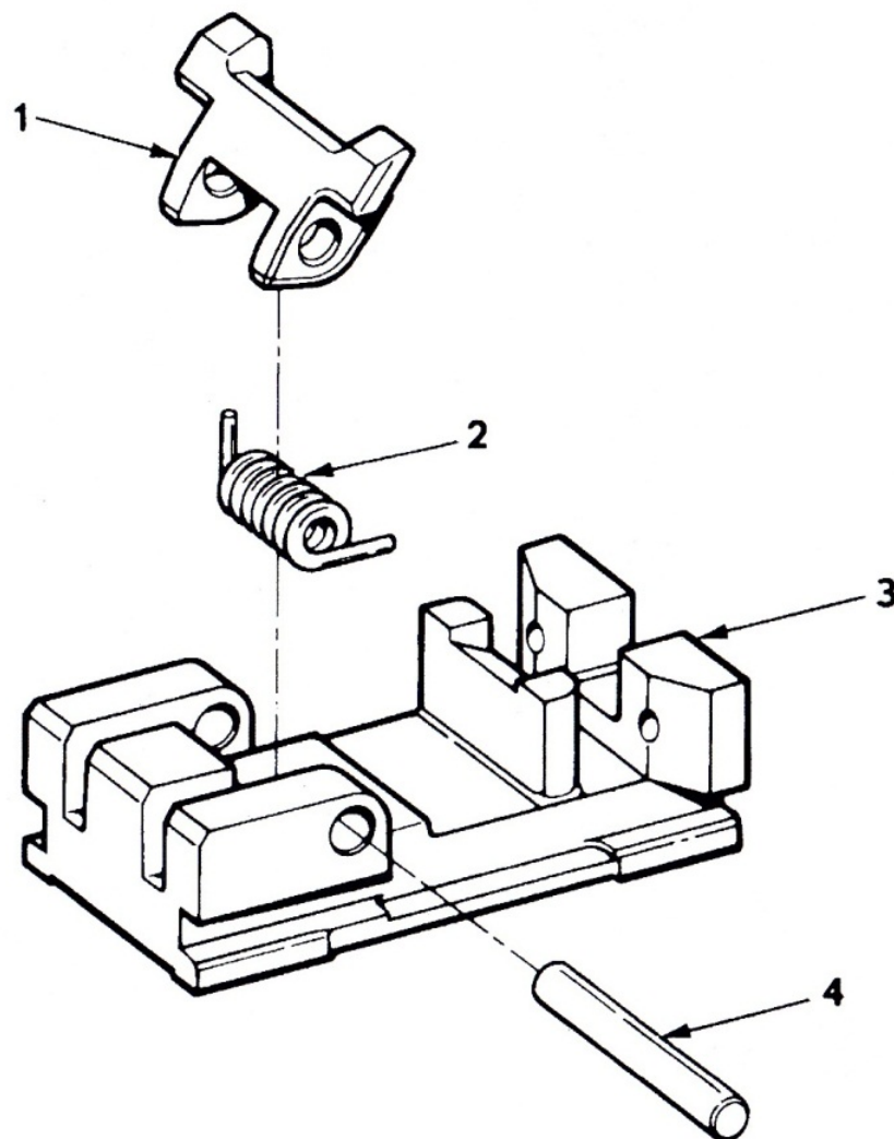
ภาพที่ 14 ชุดลิ้นเลื่อนสายกระสุน
