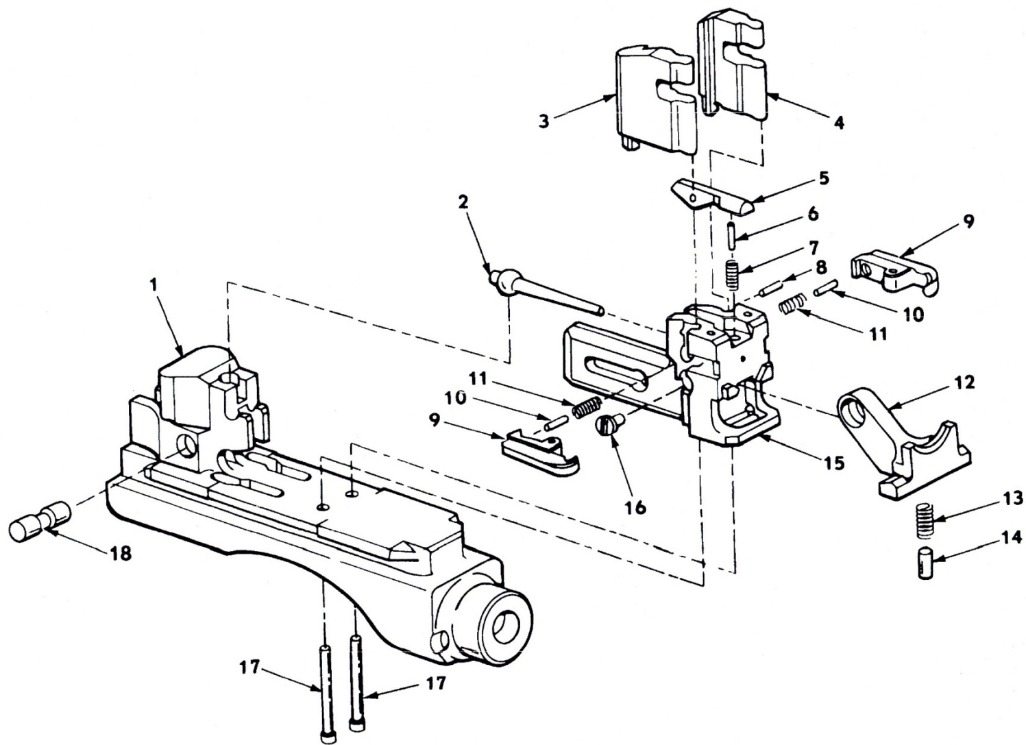
ภาพที่ 9 ชุดลูกเลื่อน
