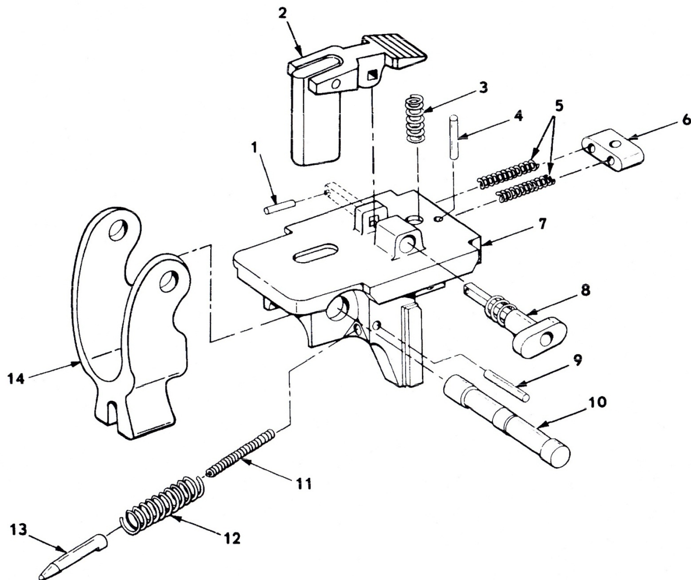
ภาพที่ 18 ชุดตัวเร่งการปลดกลอน
