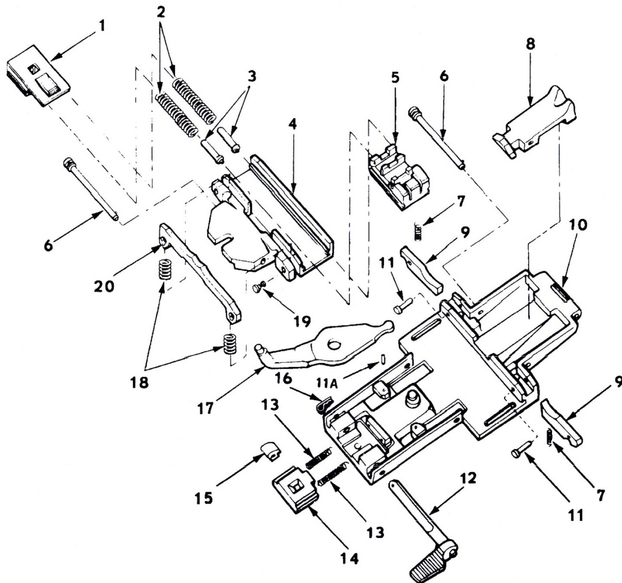
ภาพที่ 13 ชุดฝาปิดห้องลูกเลื่อน
